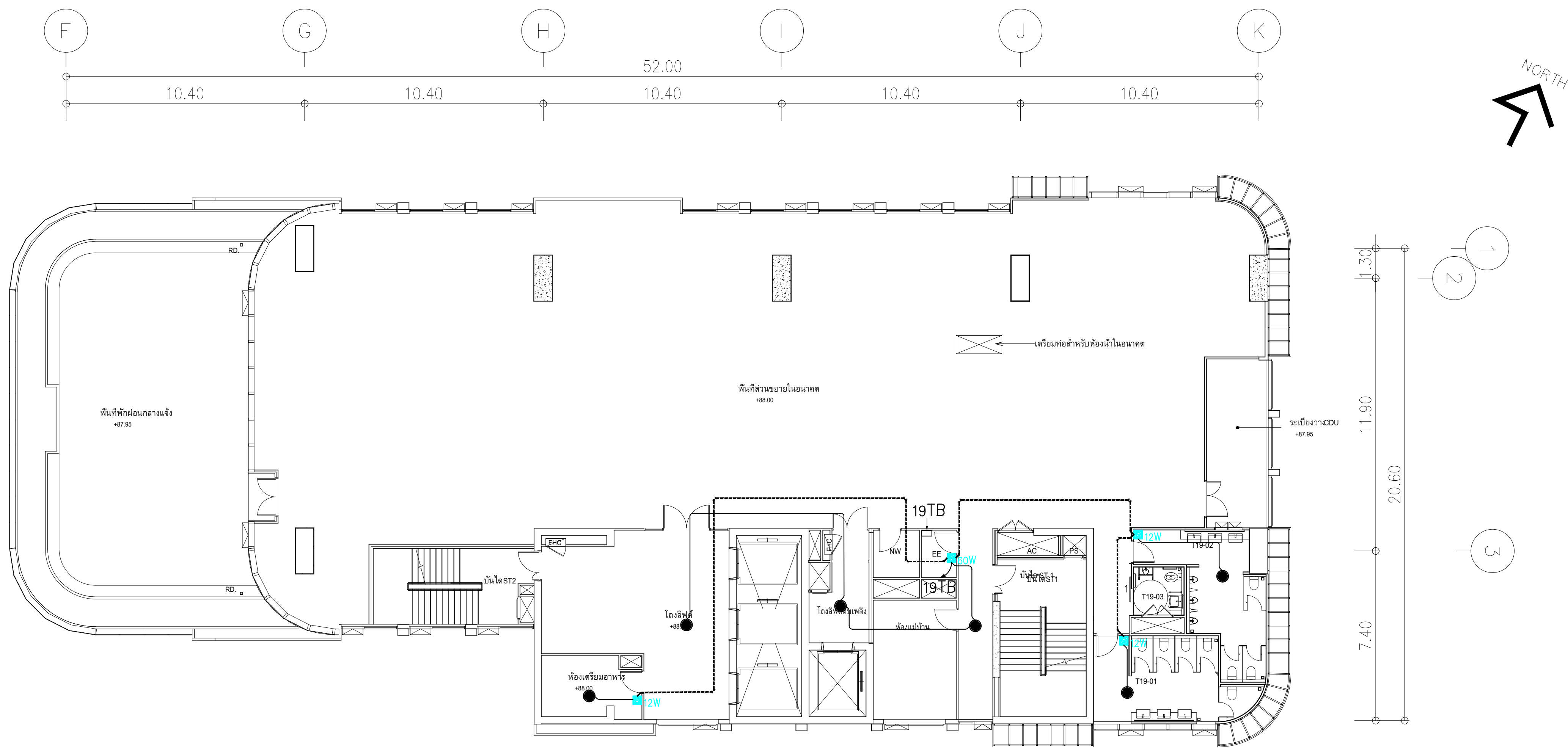
ผังแปลนระบบเสียงประกาศและ BAS ชั้น 18 มาตรฐาน 1:125
