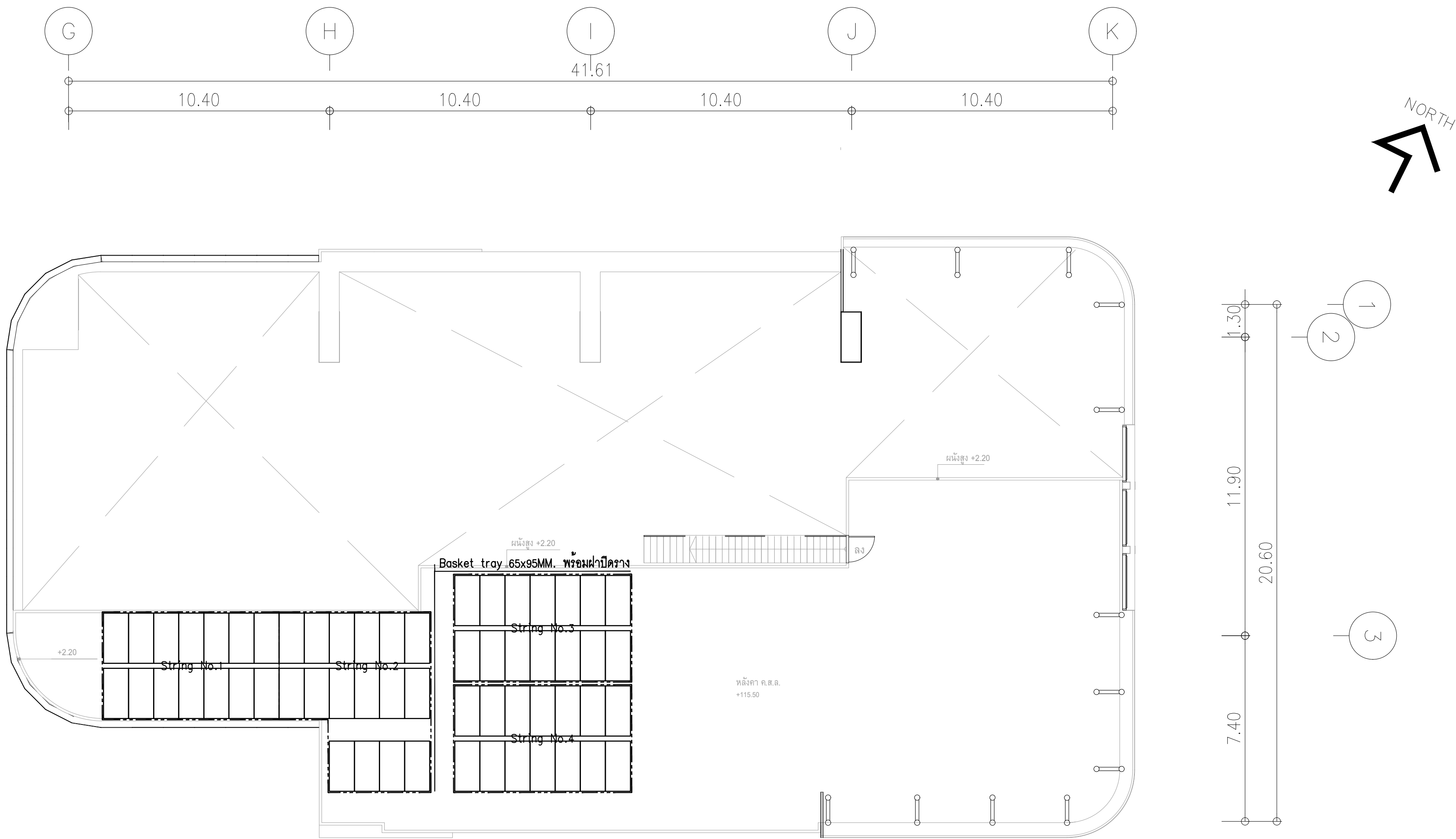
สายที่เดินจาก PV ไป DC Combiner box ใช้สาย 2x1C-4 sq.mm.PV-H1Z2Z2-K ในแต่ละ String ในราง Basket tray
