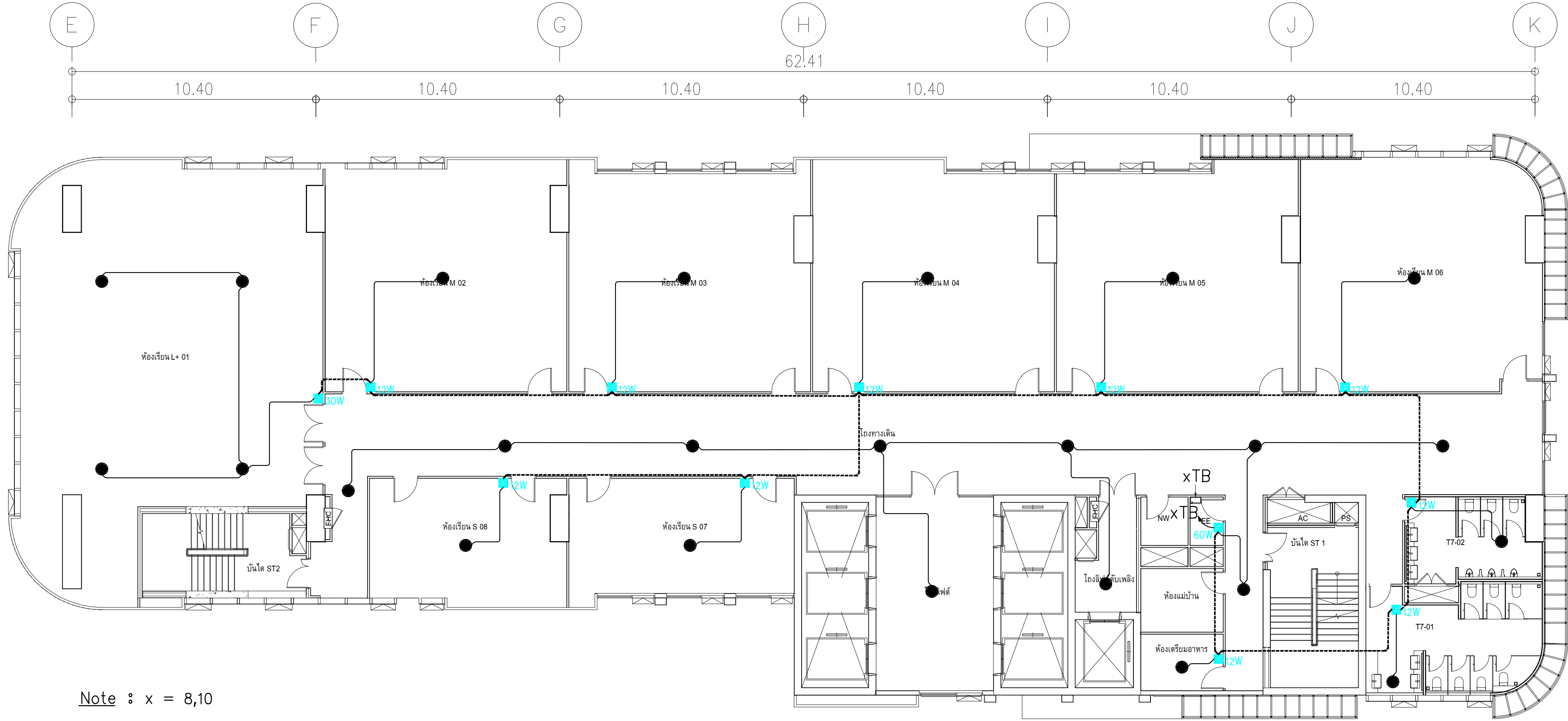
ผังแปลนระบบเสียงประกาศและ BAS ชั้น 8,10 มาตรฐาน 11125
