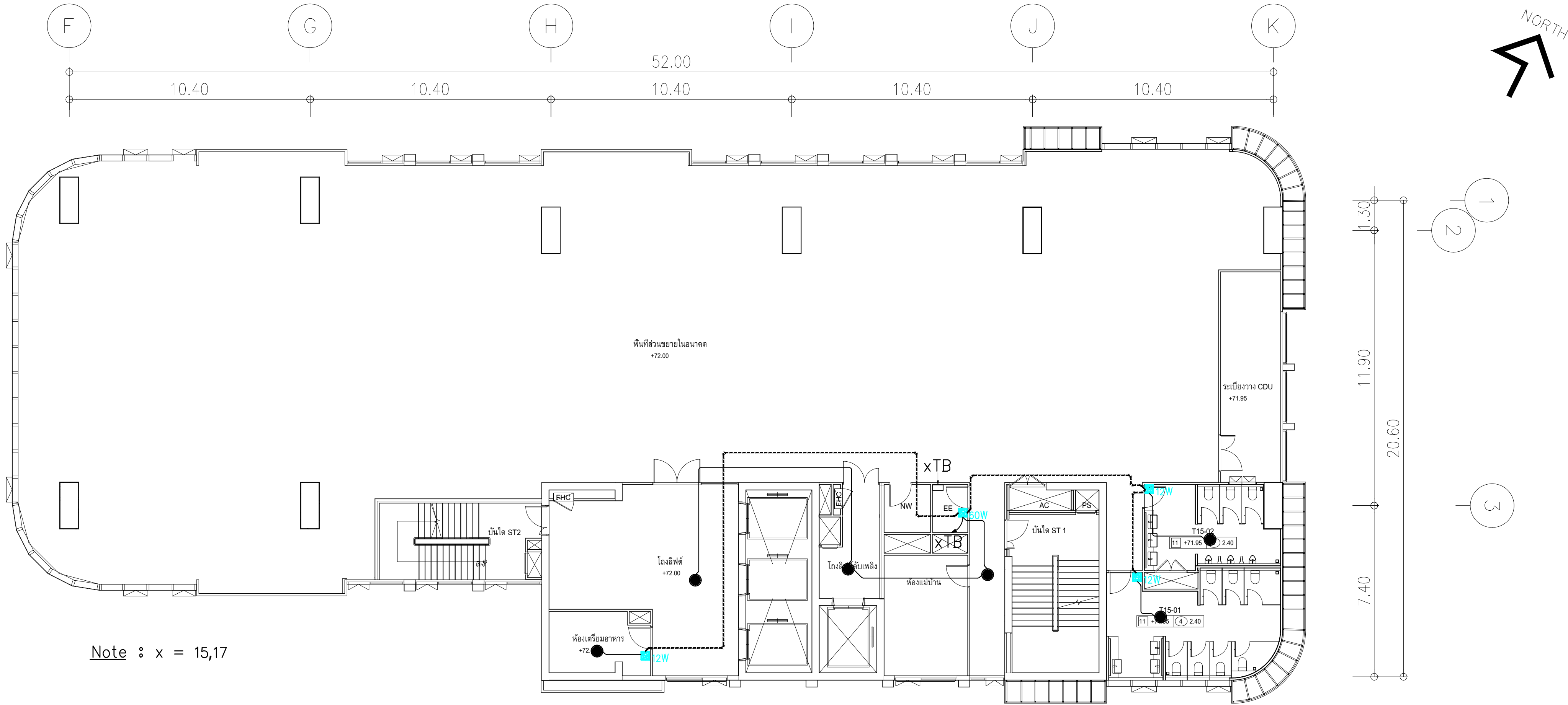
ผังแปลนระบบเสียงประกาศและ BAS ชั้น 15,17 มาตรฐาน 1:125
