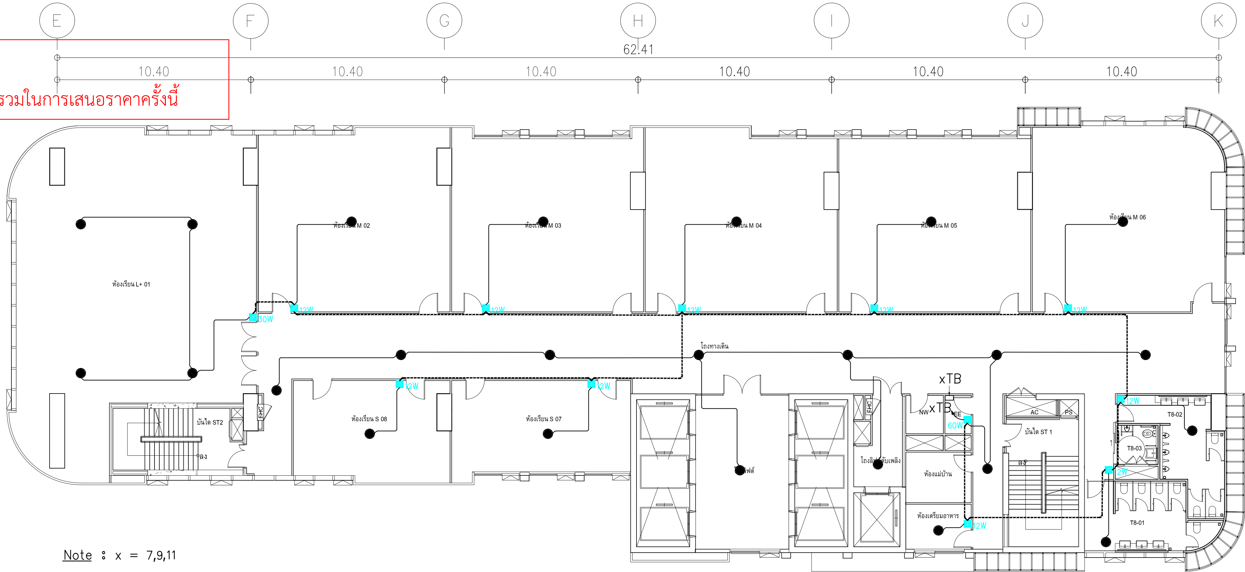
ผังแปลนระบบเสียงประกาศและ BAS ชั้น 7,9 มาตรฐาน 11125
