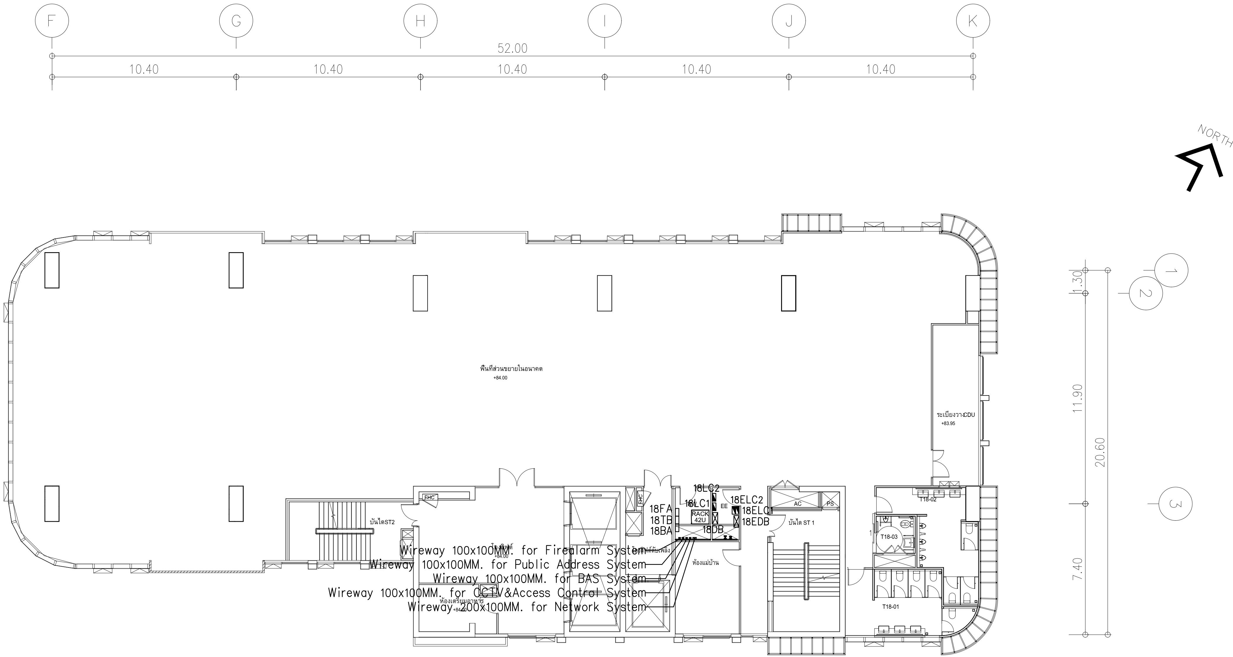
ผังแปลนแนวสายเมนไฟฟ้า ชั้น 18 ขนาดฐาน 1:125
