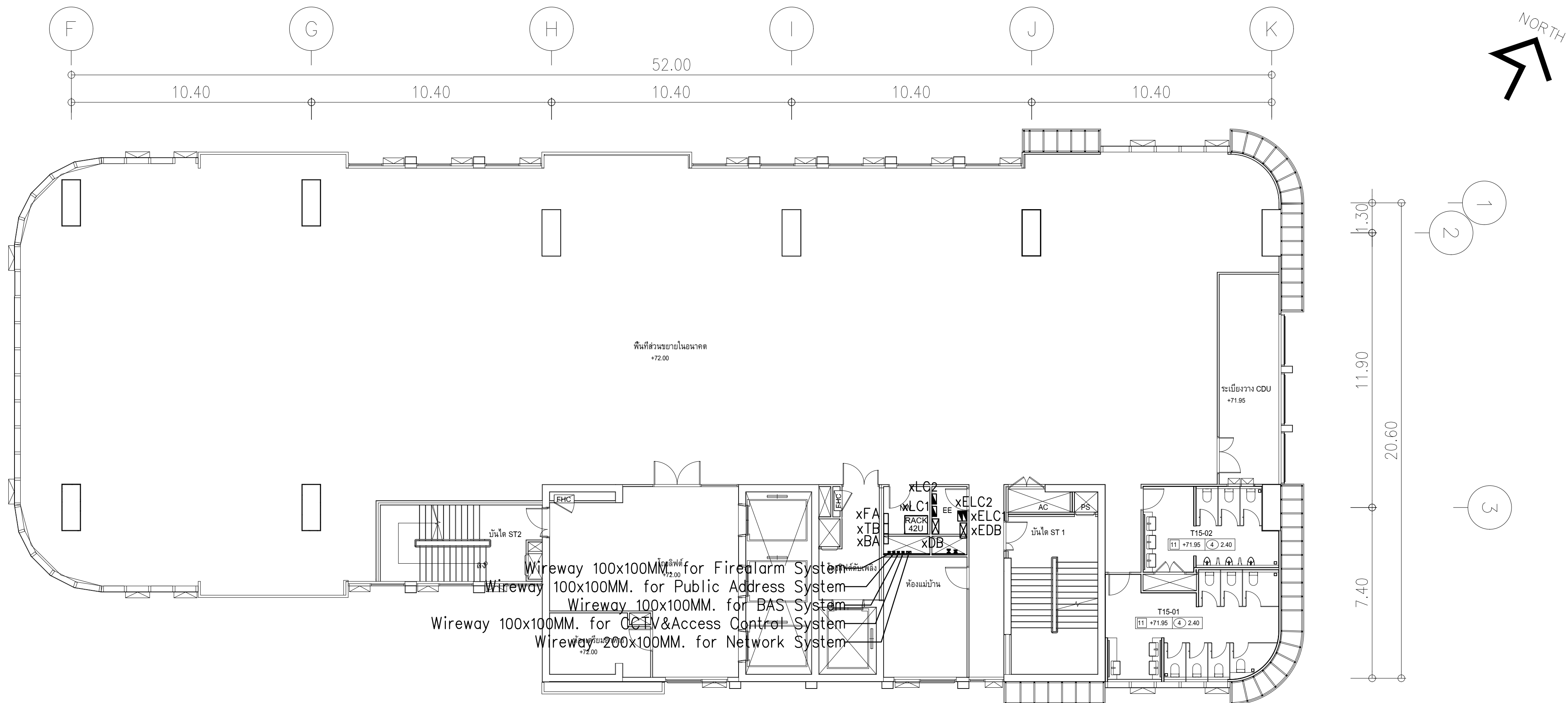
ผังแปลนแนวสายเมนไฟฟ้า ชั้น 15,17 มาตราส่วน 1:125
