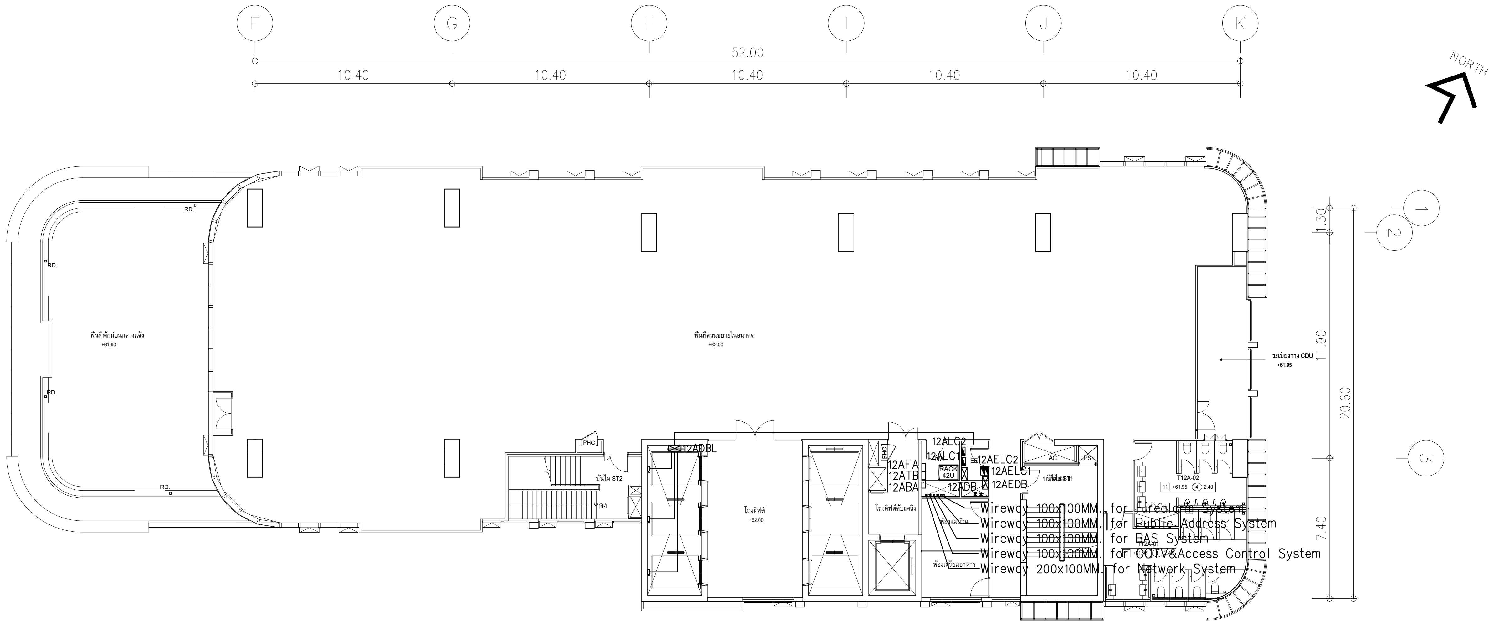
ผังแปลนแนวสายเมนไฟฟ้า ชั้น 12A มาตรฐาน 1:125
