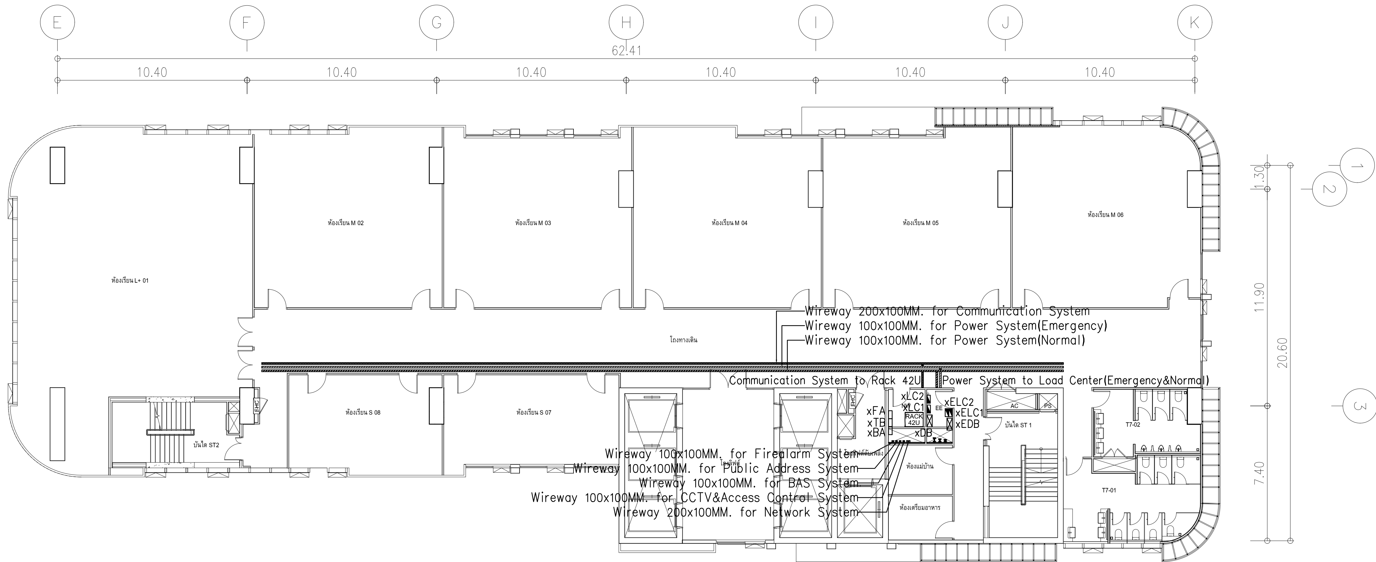
ผังแปลนแนวสายเมนไฟฟ้า ชั้น 8,10 มาตราส่วน 1:125
