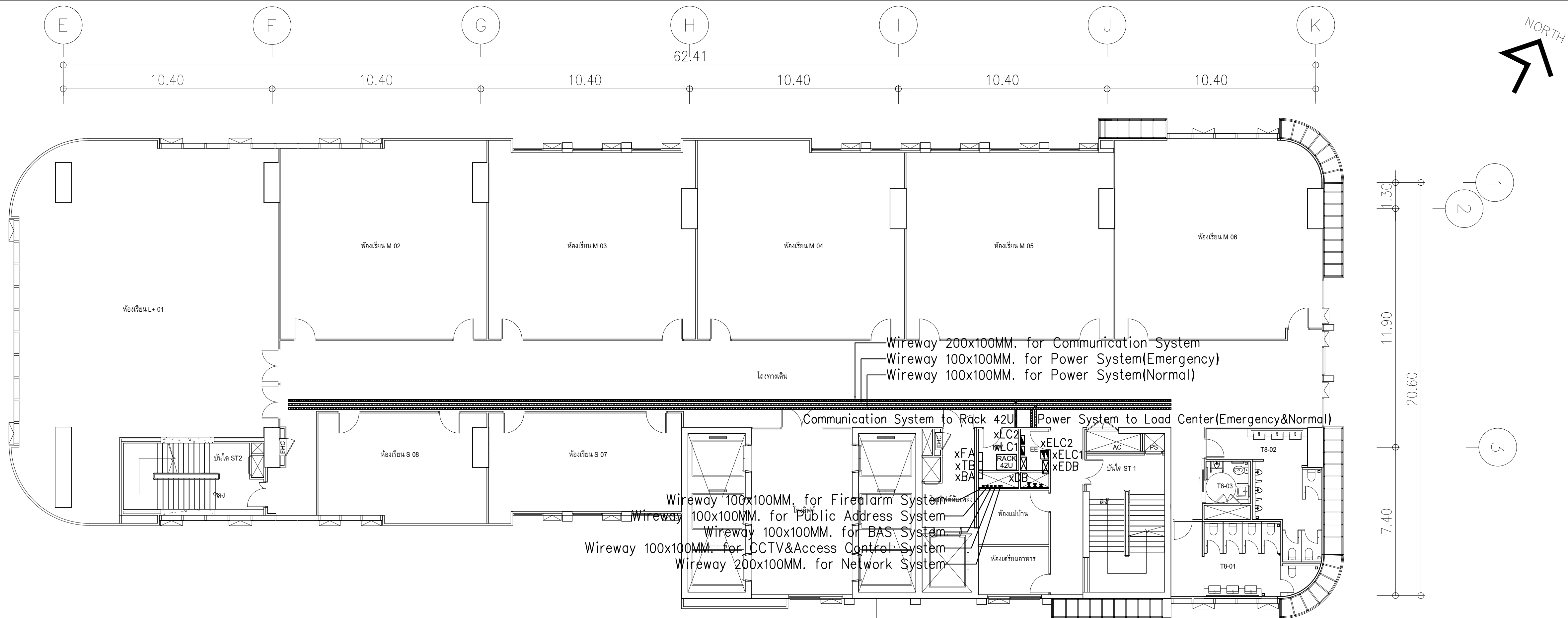
ผังแปลนแนวสายเมนไฟฟ้า ชั้น 7,9 มาตราส่วน 1:125
