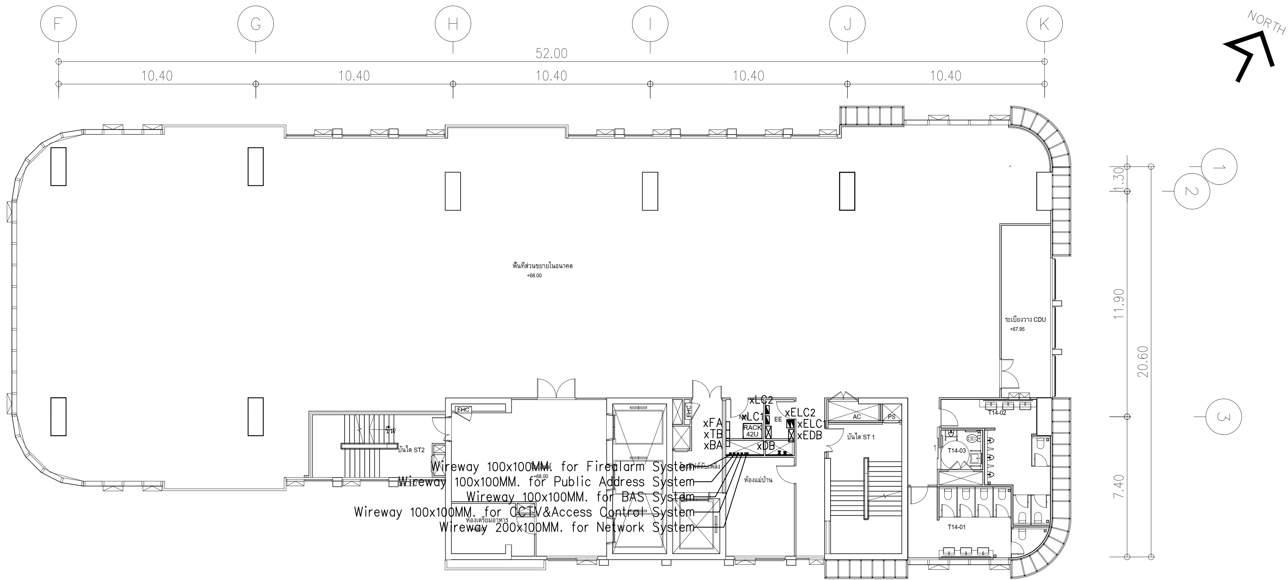
ผังแปลนแนวสายเมนไฟฟ้า ชั้น 14,16 มาตราส่วน 1:125
