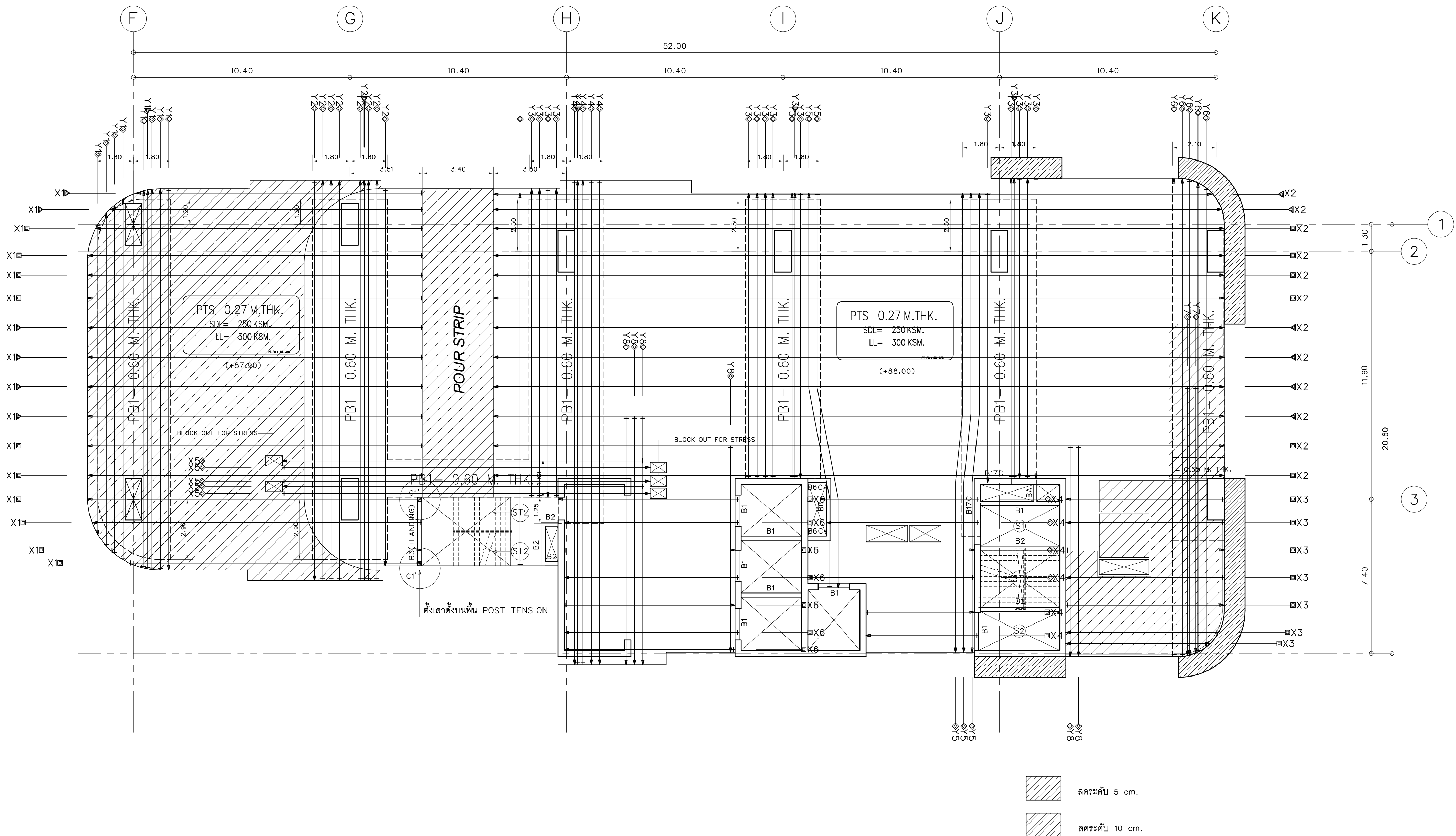
ผัง คาน, พื้นชั้นที่ 19 มาตราส่วน 1:125 (TENDONS LAY-OUT)
