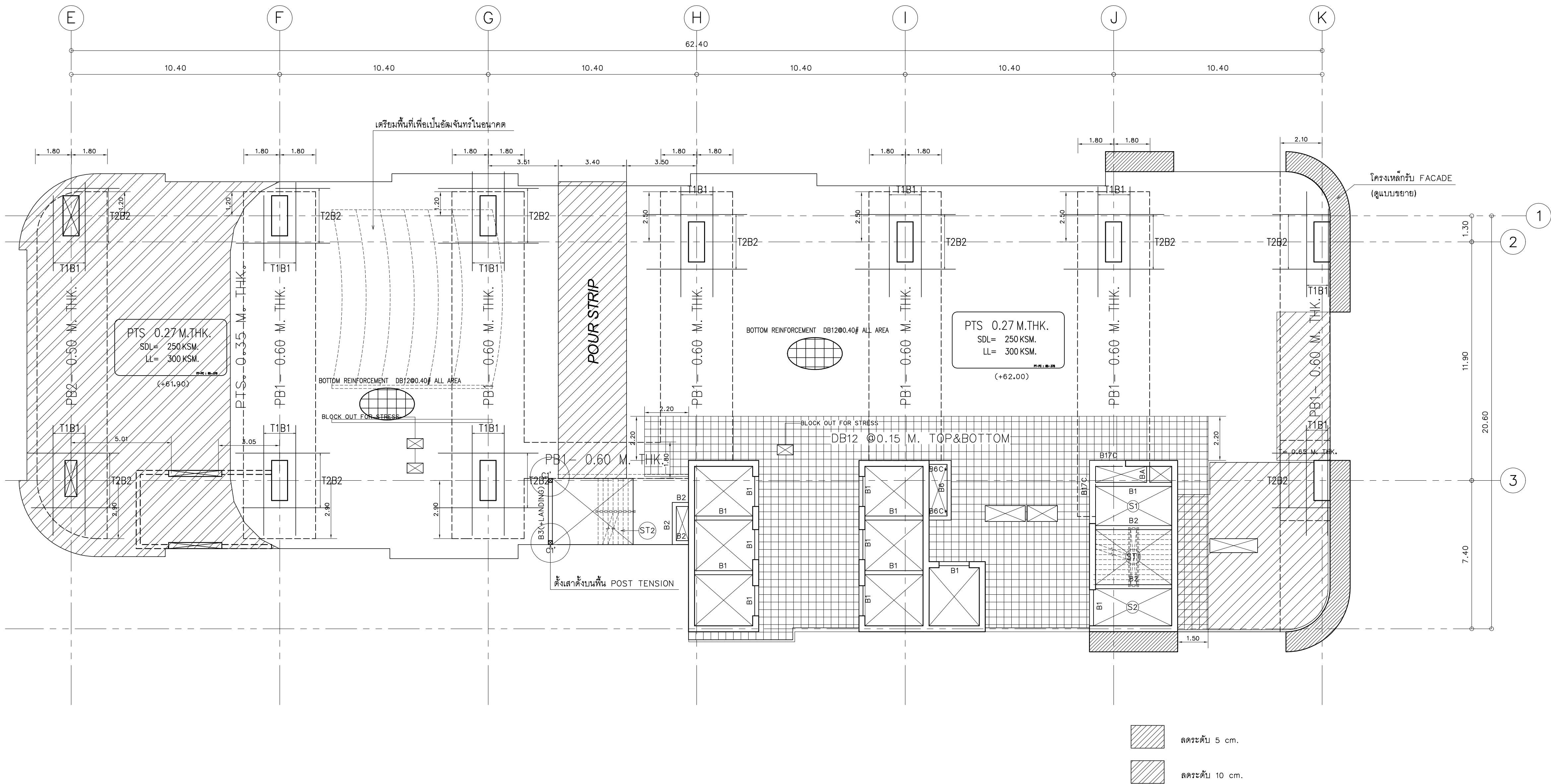
ผัง คาน, พื้นชั้นที่ 12A มาตราส่วน 1:125 (MILD STEELS LAY-OUT)
