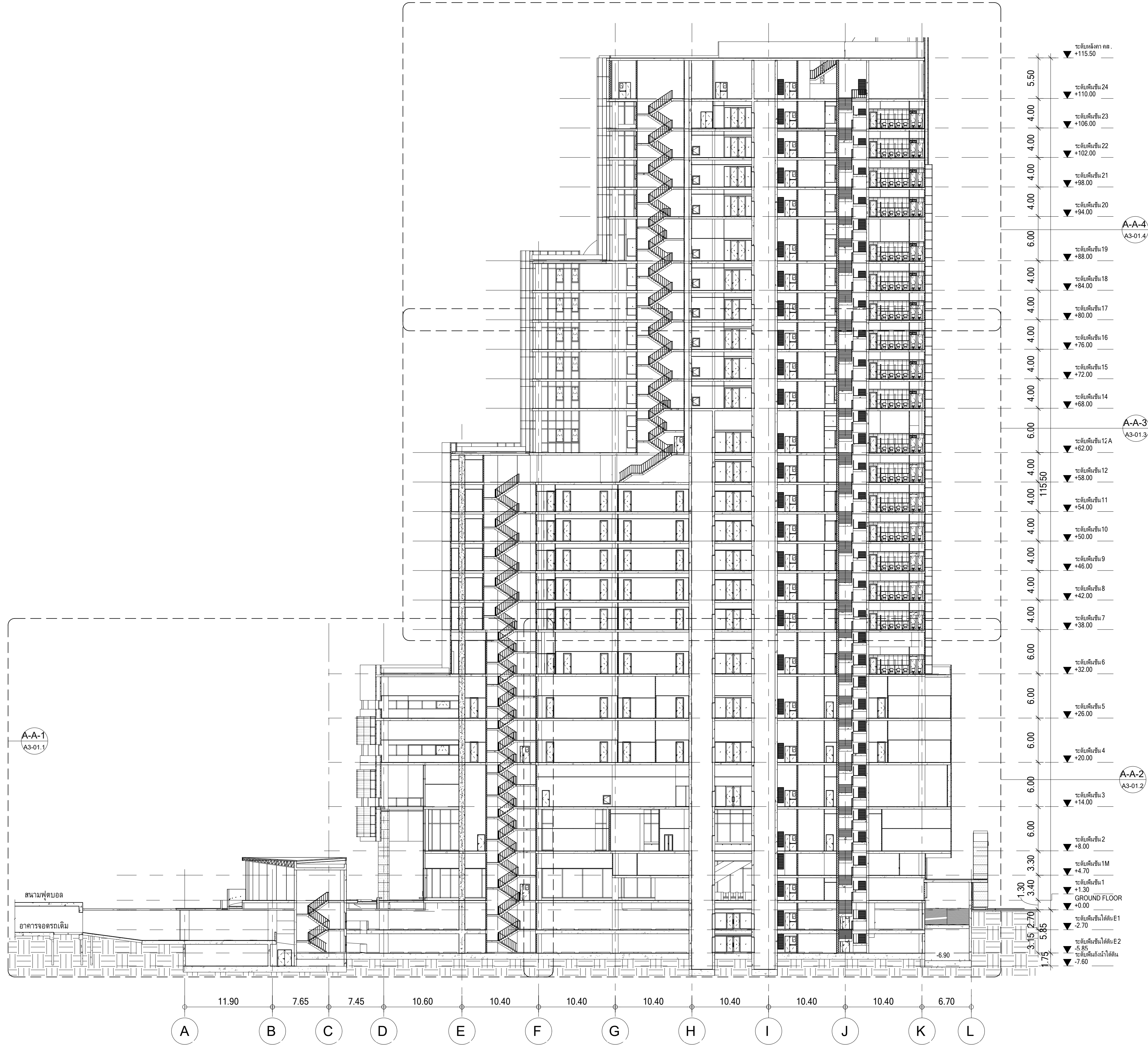
รูปตัดอาคารแนว A-A มาตราส่วน 1 : 300
