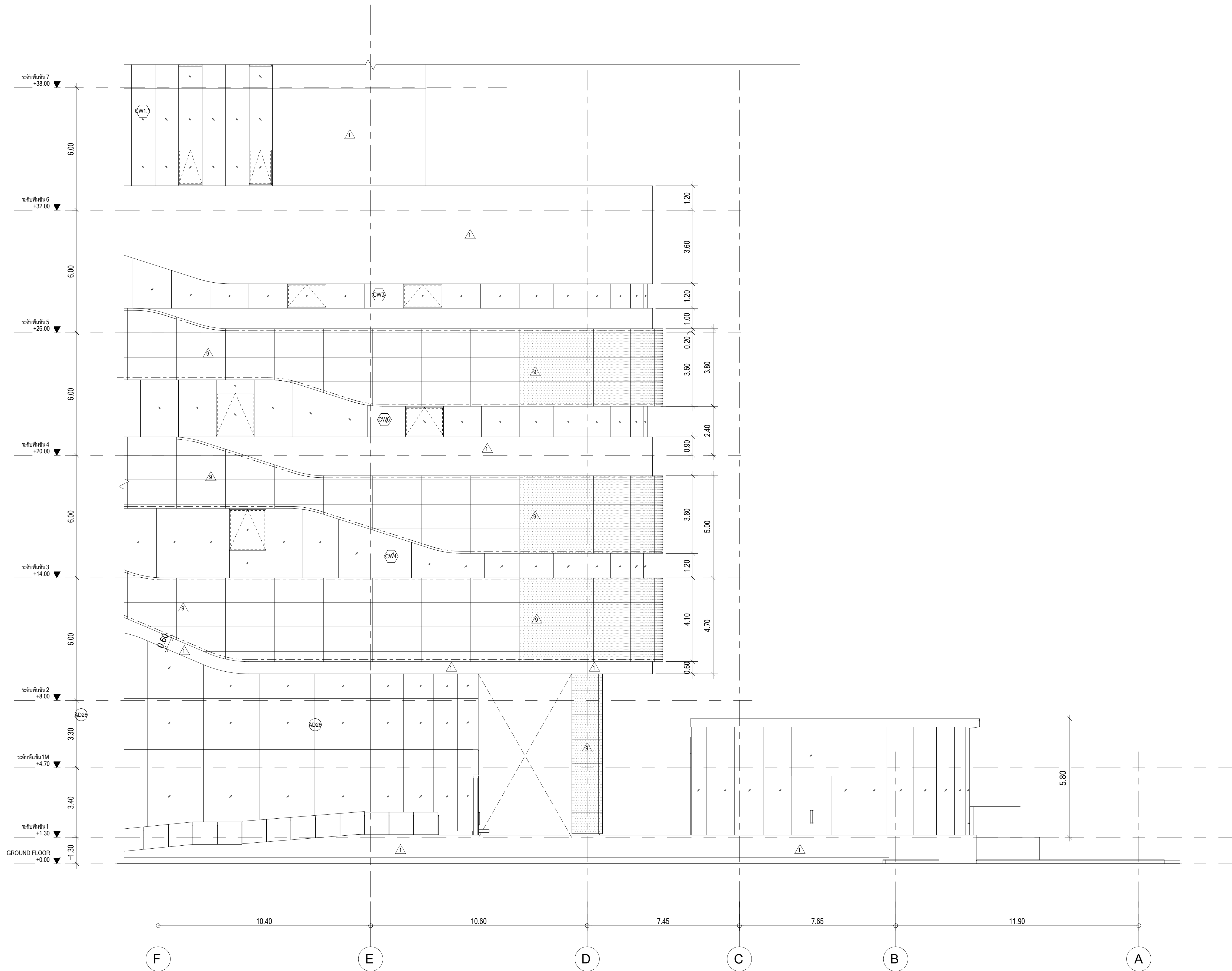
รูปด้านอาคาร 2, ส่วนที่ 2 มาตราส่วน 1 : 100
