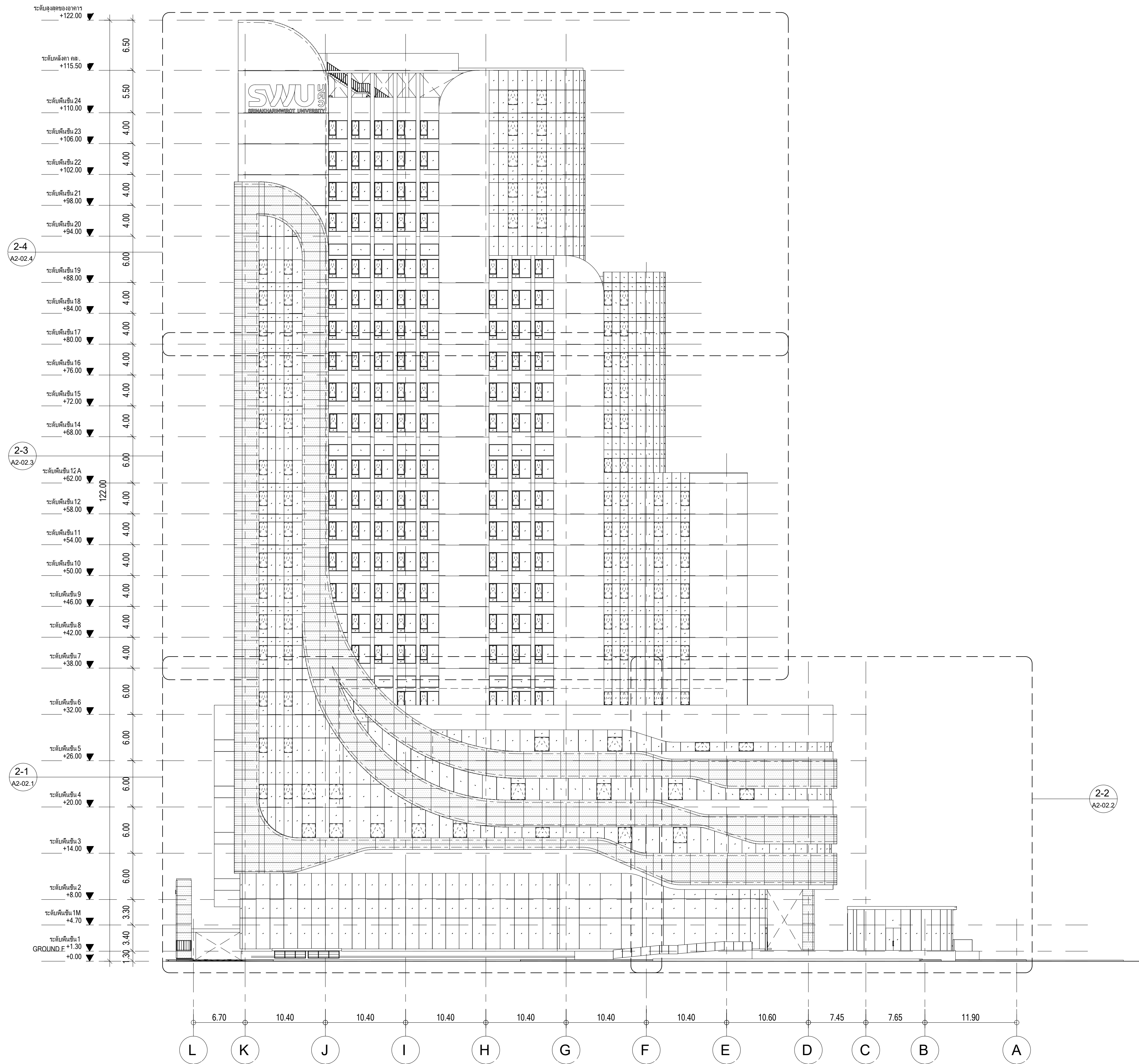
รูปด้านอาคาร 2 มาตราส่วน 1 : 300
