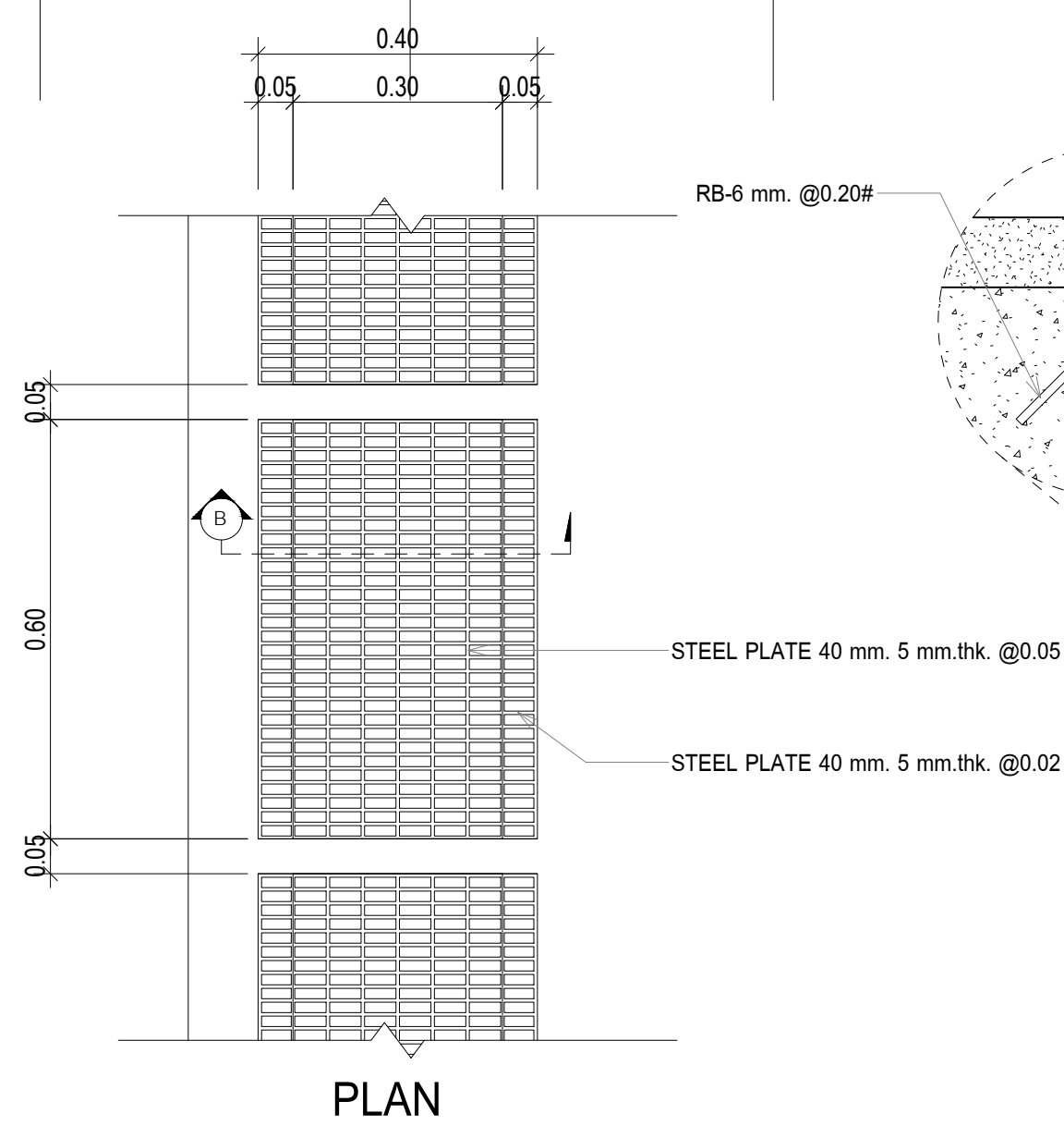
แบบขยาย GUTTER มาตราส่วน 1 : 10
