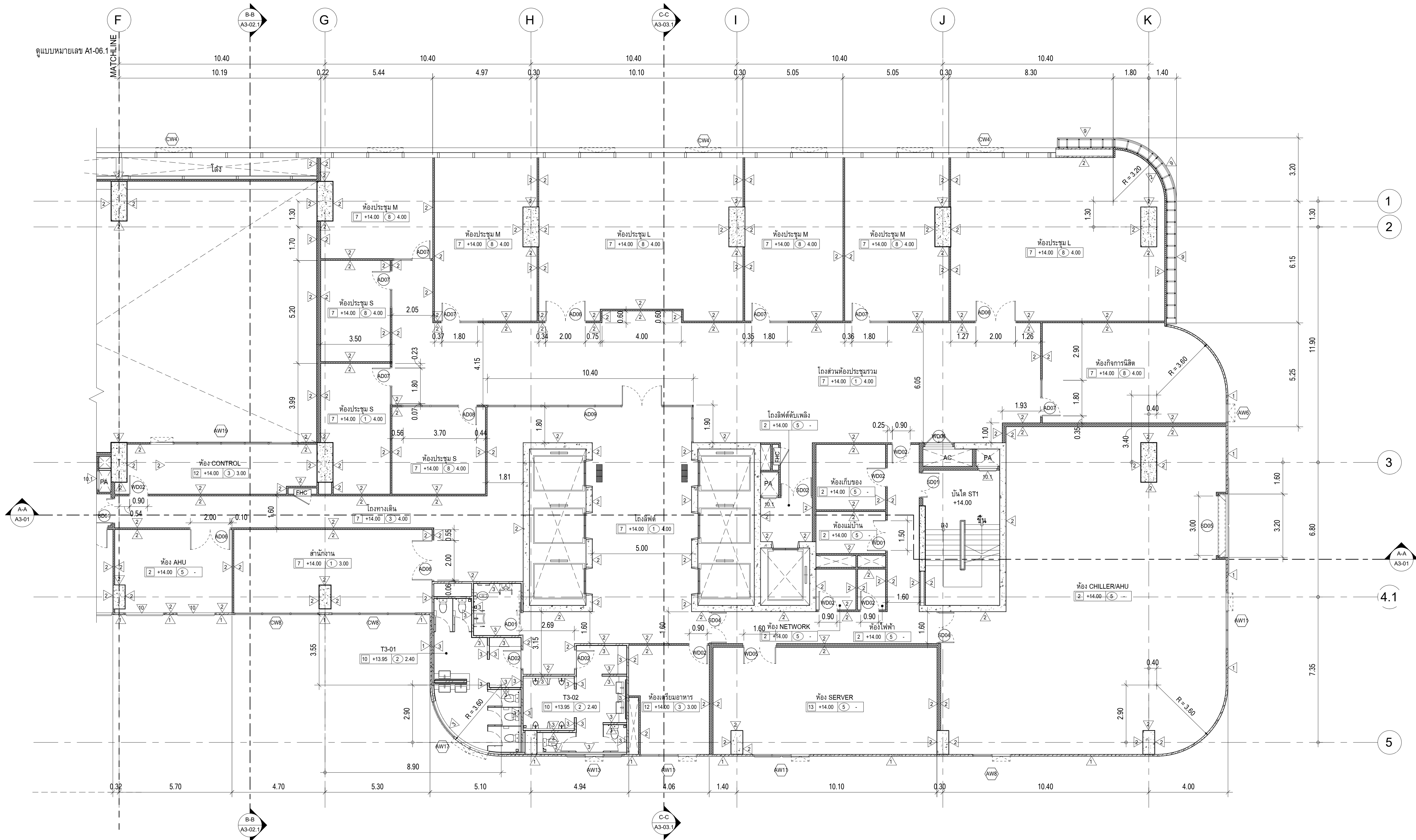
ผังพื้นที่ 3, ส่วนที่ 2 มาตราส่วน 1 : 100
