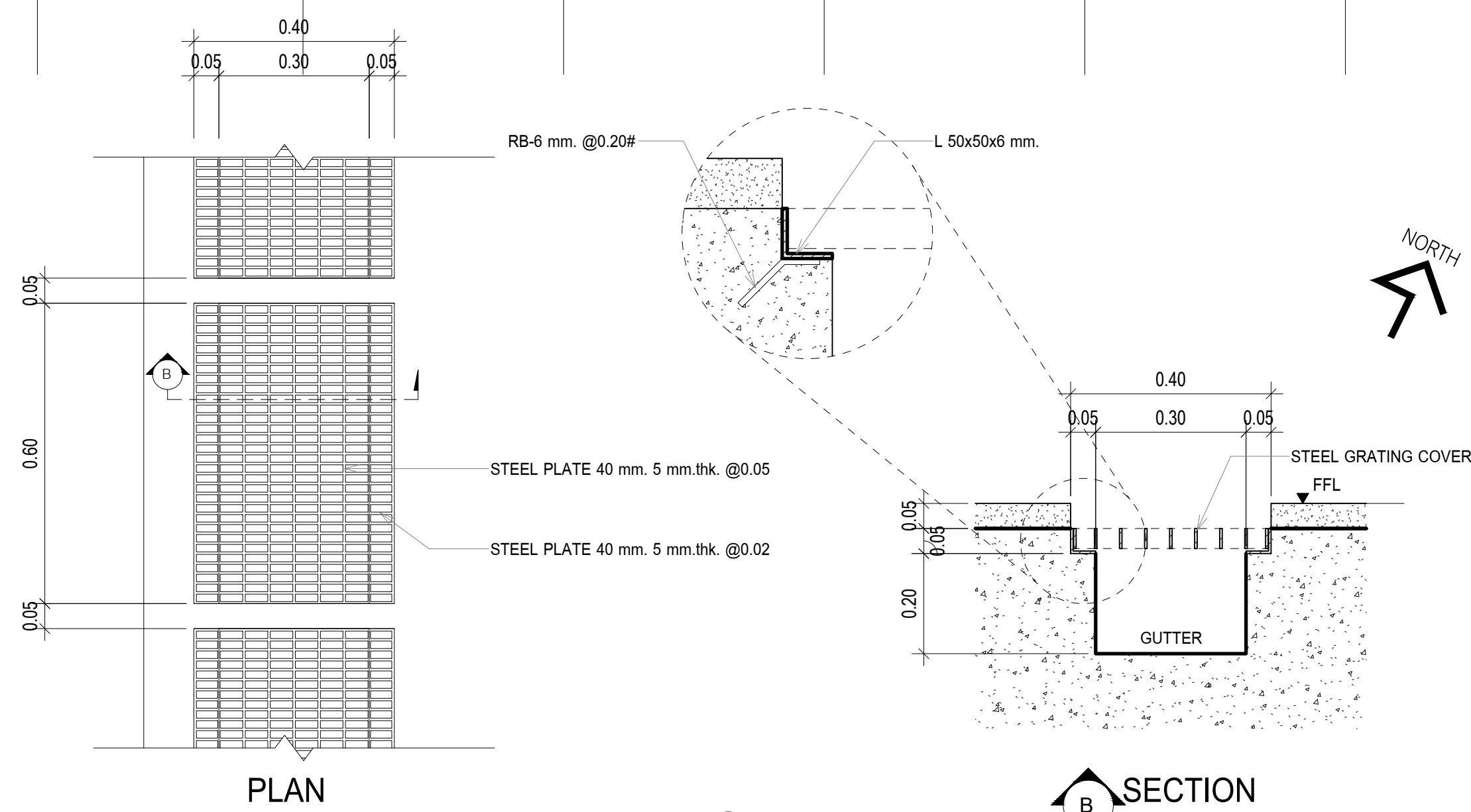
แบบขยาย GUTTER มาตราส่วน 1 : 10
