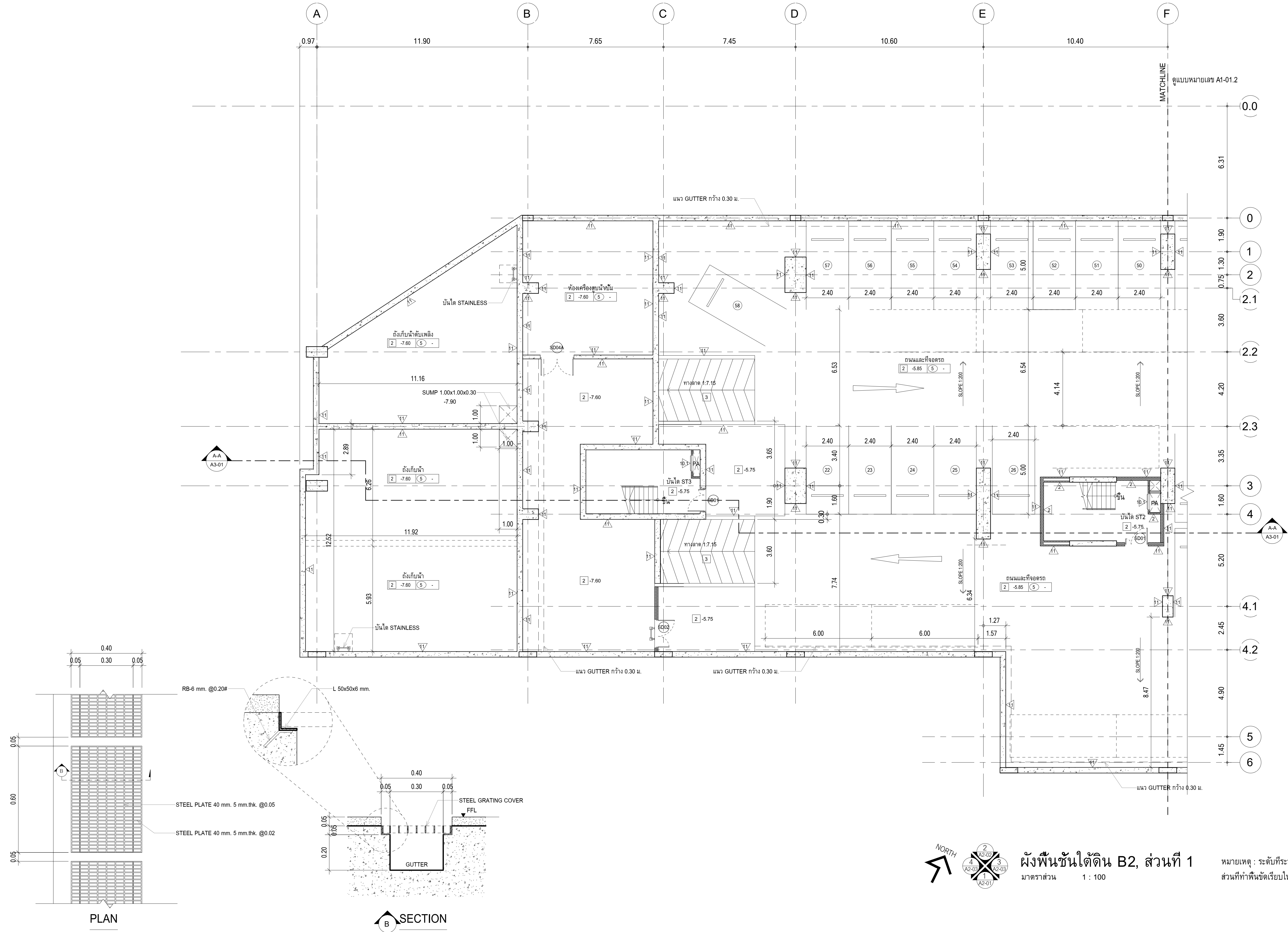
แบบขยาย GUTTER มาตราส่วน 1 : 10
