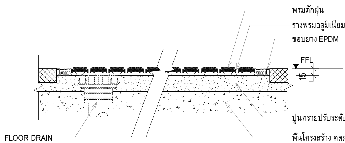
แบบขยายพรมดักฝุ่น มาตราส่วน 1 : 5
