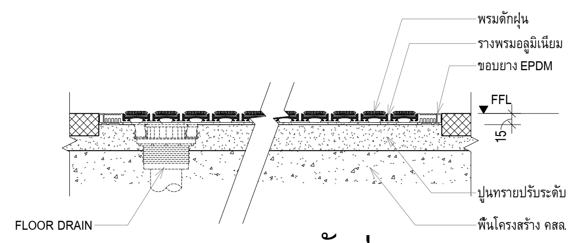
แบบขยายพรมดักฝุ่น มาตราส่วน 1 : 5
