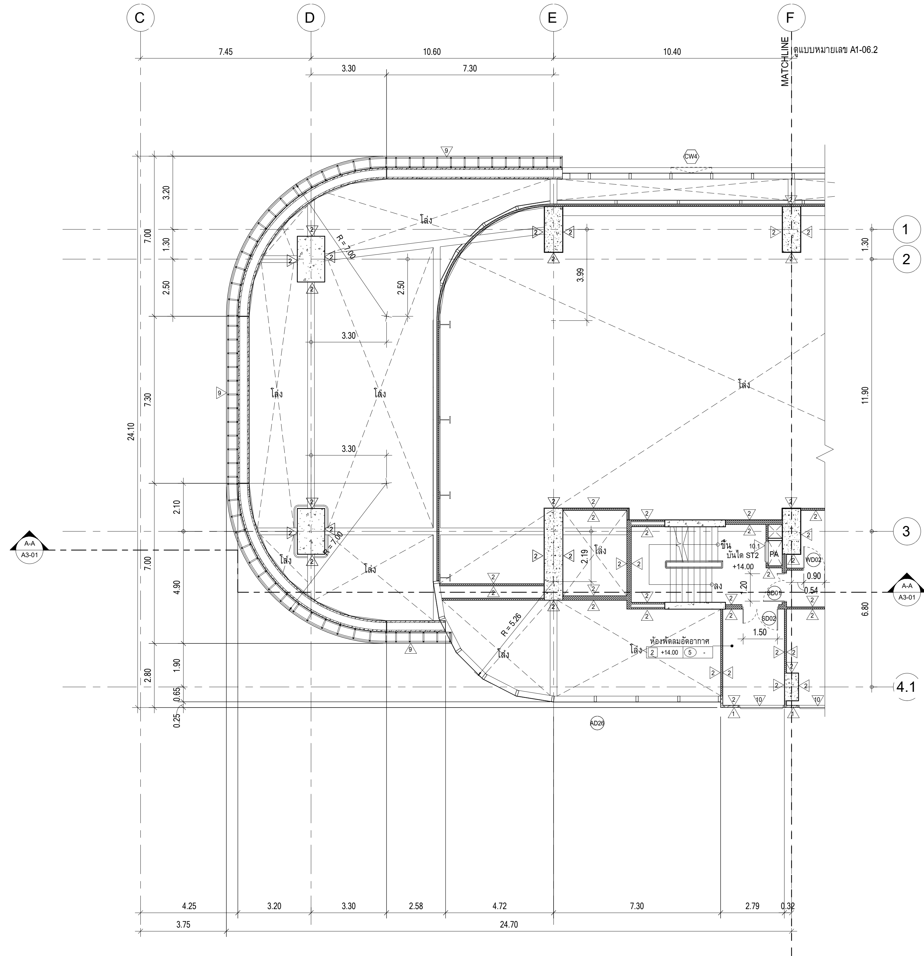
ผังพื้นชั้น 3, ส่วนที่ 1 มาตราส่วน 1 : 100
