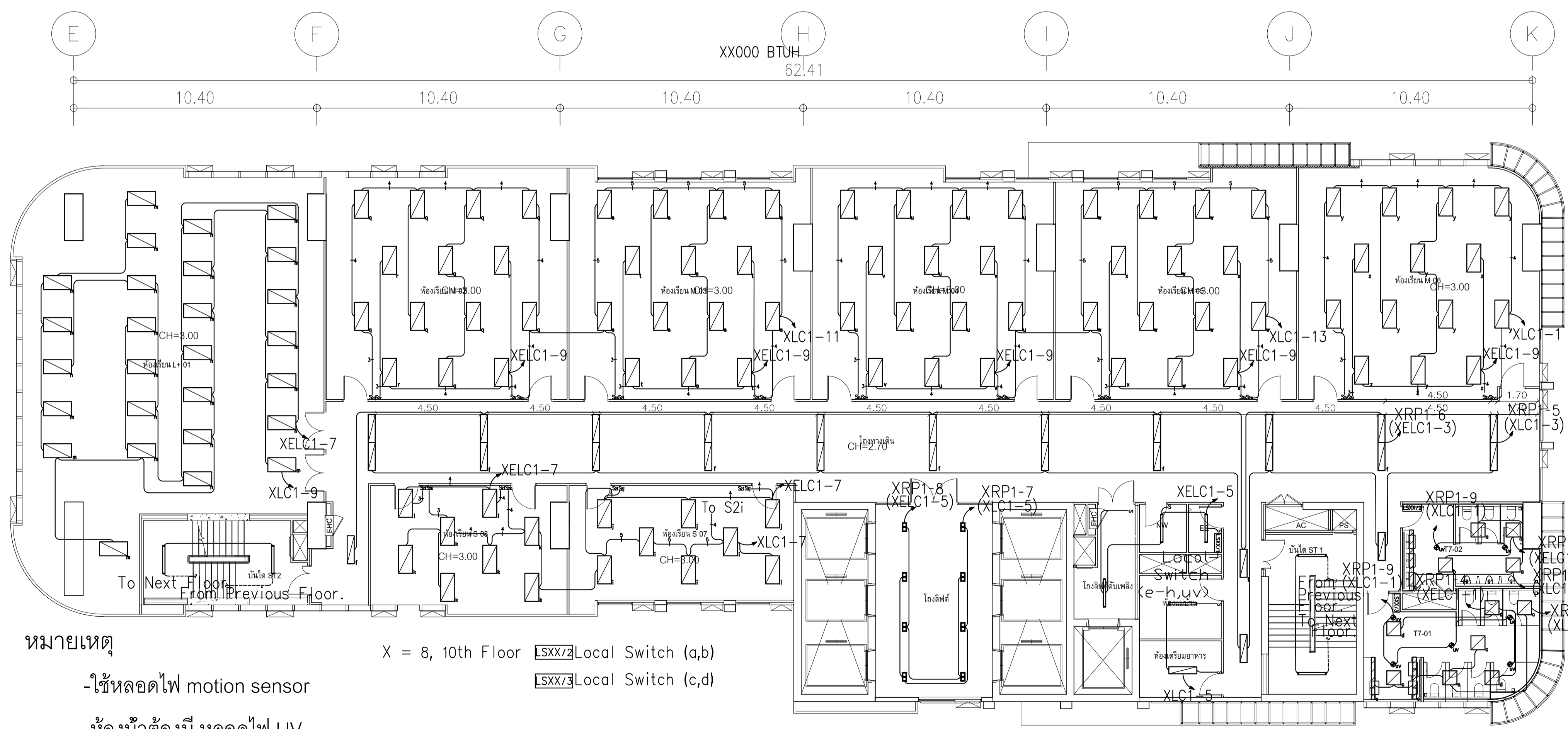
ผังแปลนระบบแสงสว่าง ชั้น 8,10 มกราคม 11125
