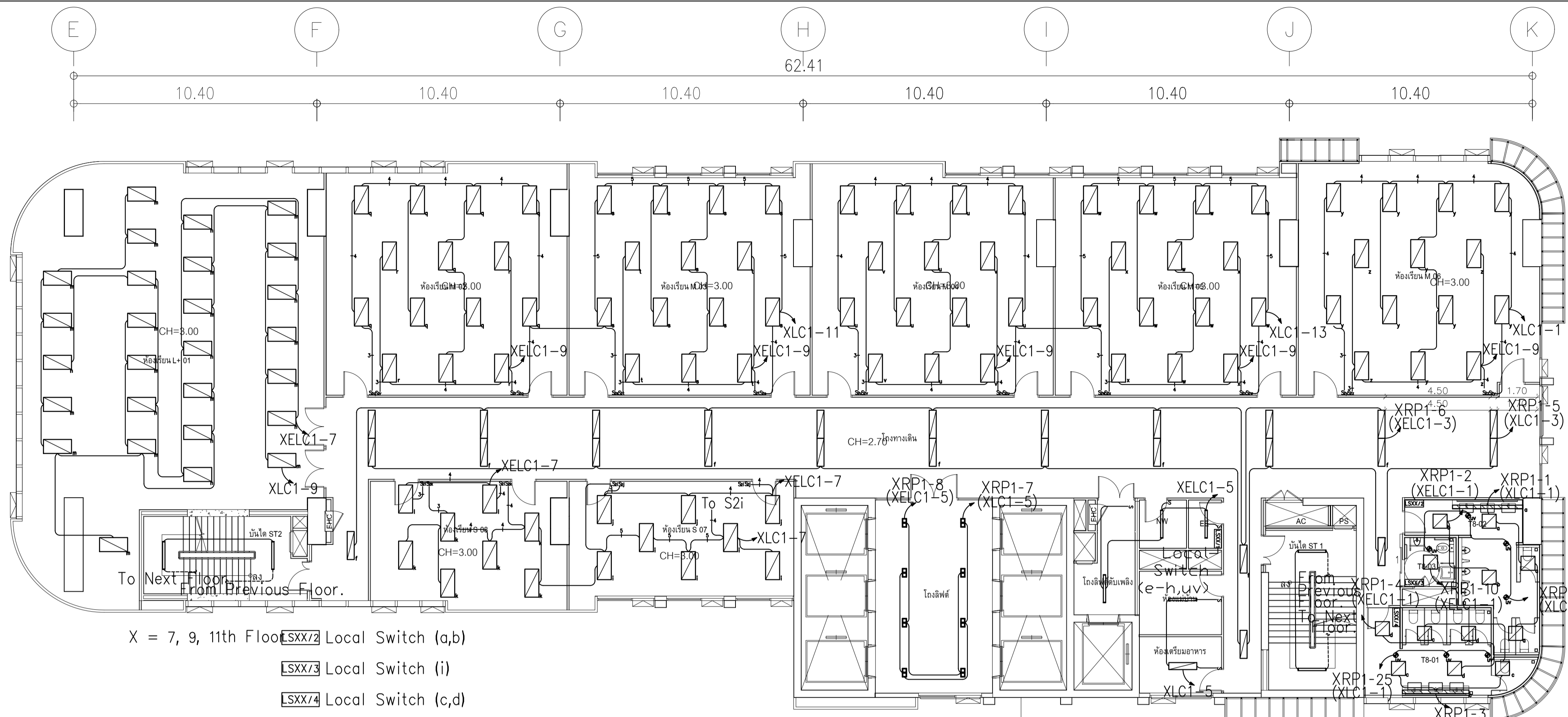
ผังแปลนระบบแสงสว่าง ชั้น 7,9 มกราคม 11125
