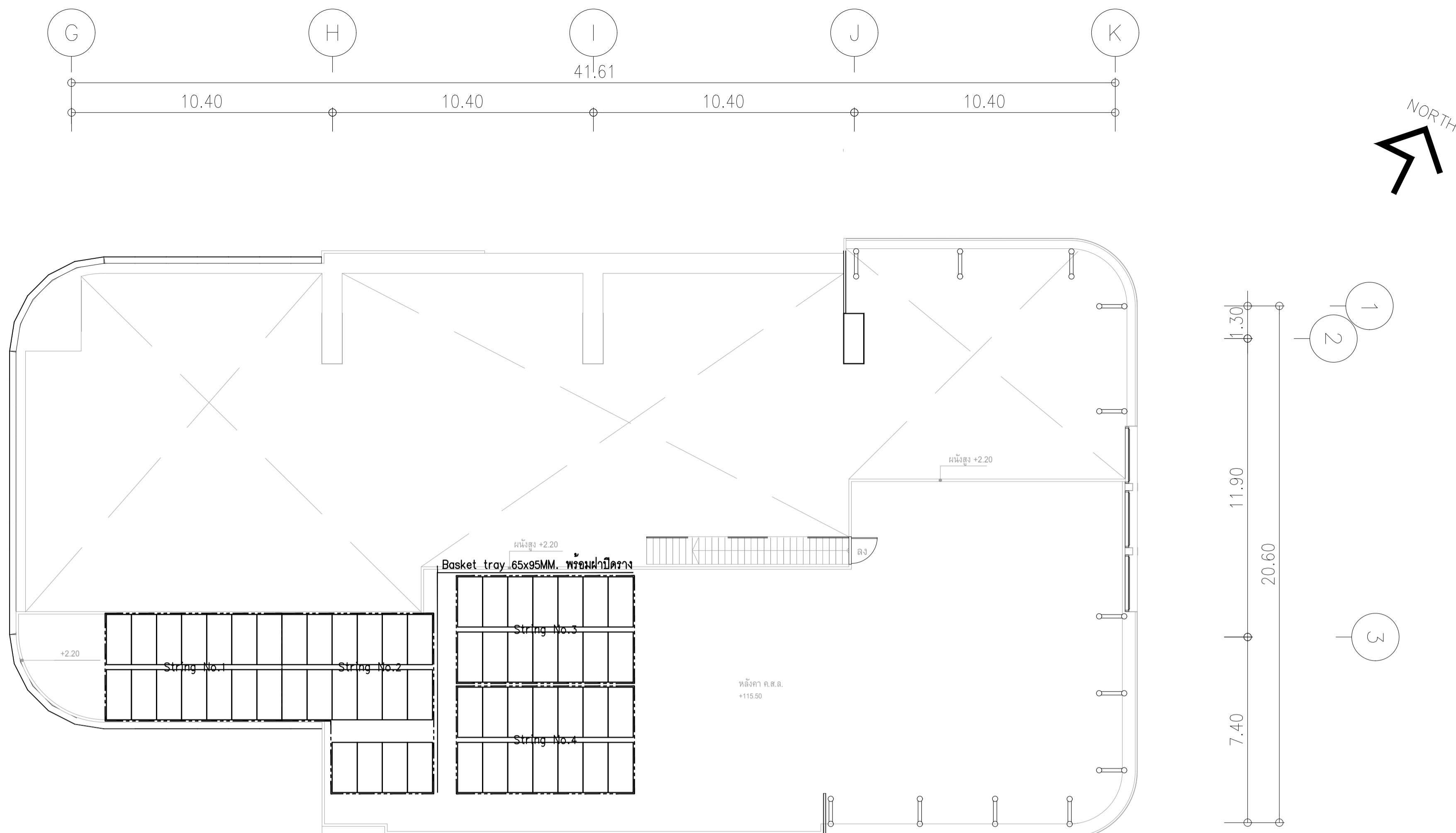
สายที่เดินจากแผง PV ไป DC Combiner box ไซส์สาย 2x1C-4 sq.mm.PV-H1Z2Z-K ในแต่ละ String ในวาง Basket tray ผังแปลนระบบผลิตไฟฟ้า พลังงานแสงอาทิตย์ ชั้นหลังคา มาตรฐาน 1:125
