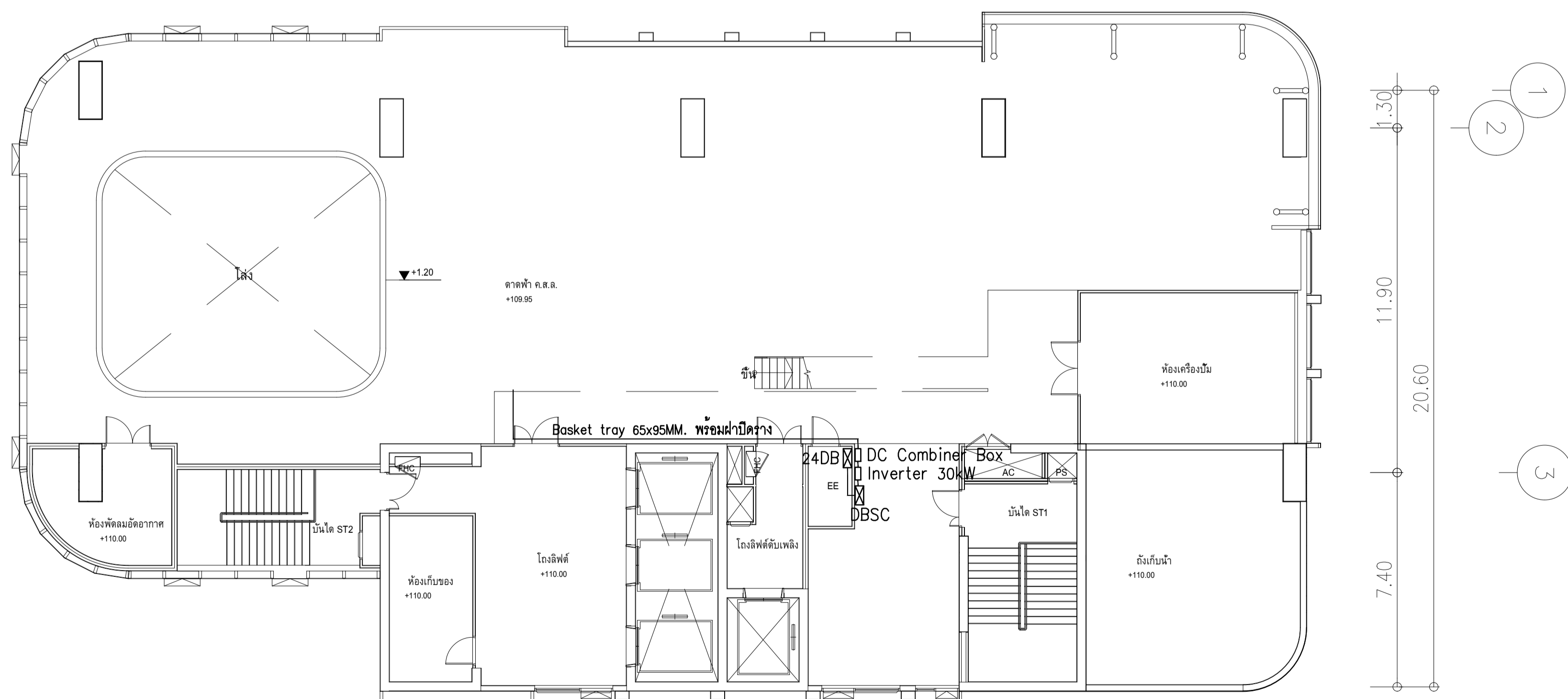
ผังแปลนระบบผลิตไฟฟ้า พลังงานแสงอาทิตย์ ชั้น 24 มาตรฐาน 1:125
