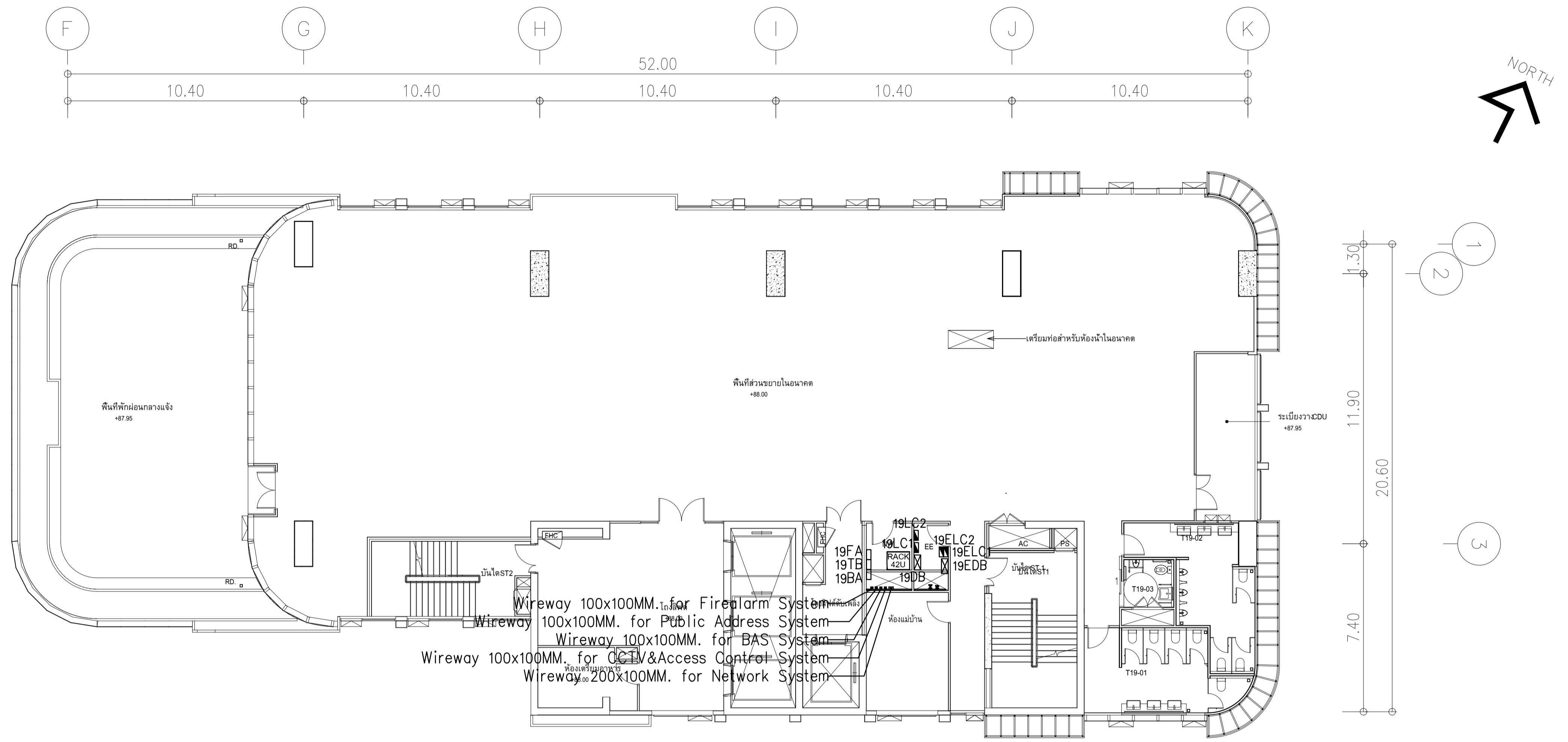
ผังแปลนแนวสายเมนไฟฟ้า ชั้น 19 มาตรฐาน 1:125
