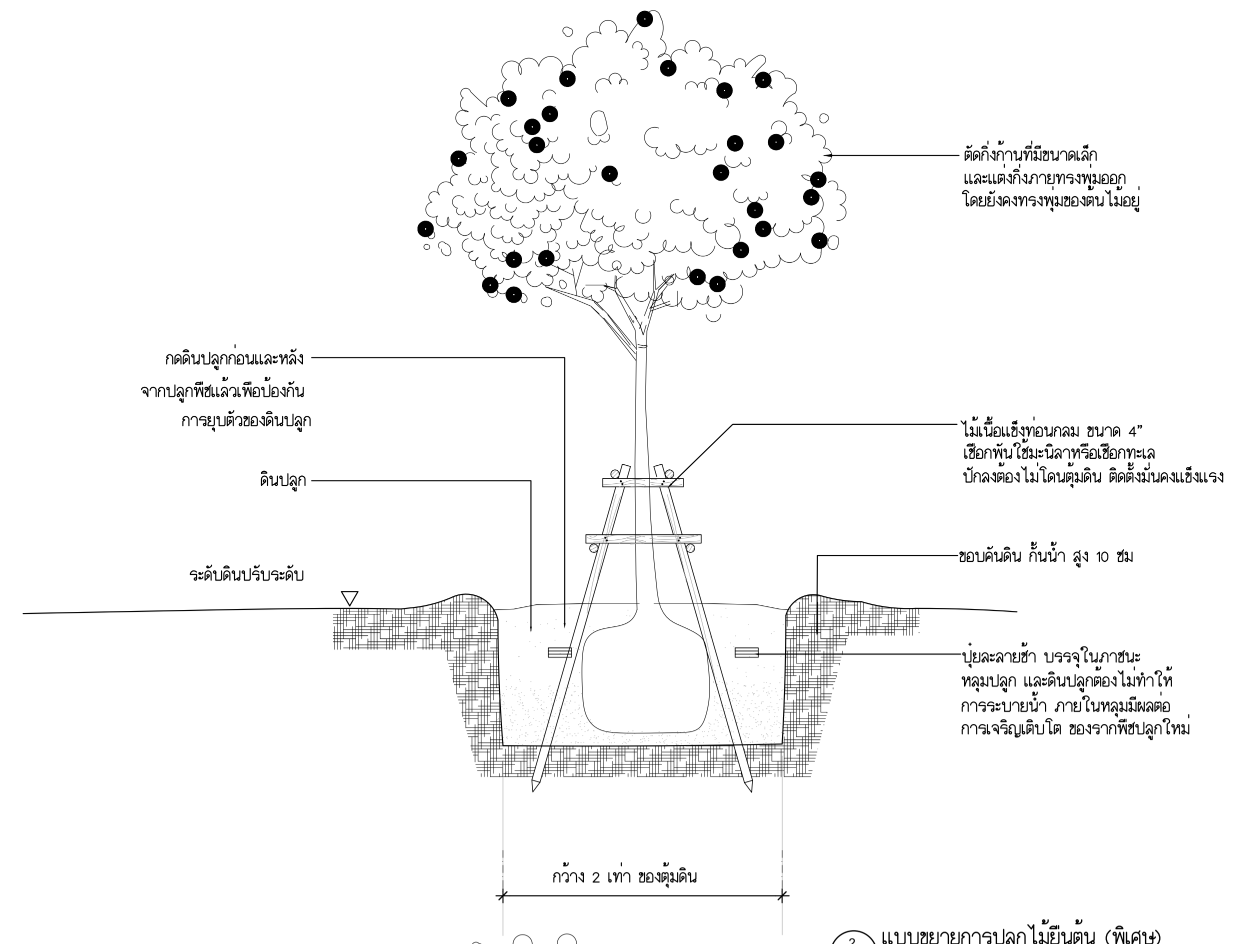
2 แบบขยายการปลูกไม้ยืนต้น (พิเศษ) LA-02.2 มาตรฐาน 1 : 25
