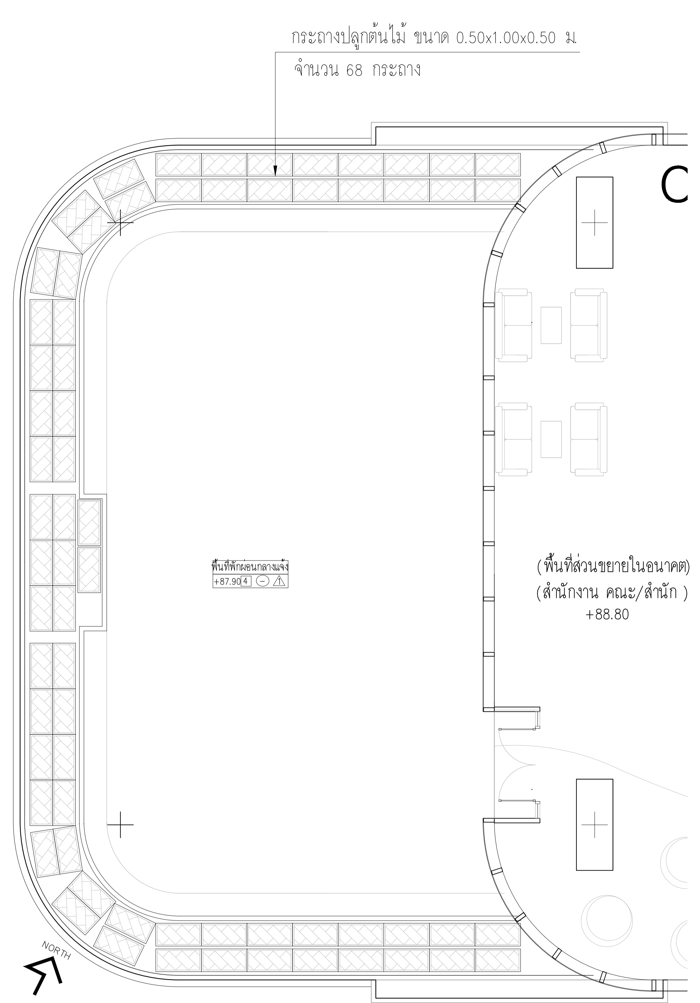
ผังแสดงจำนวนกระถางต้นไม้ ชั้นที่ 19 มาตรฐาน 1:50
