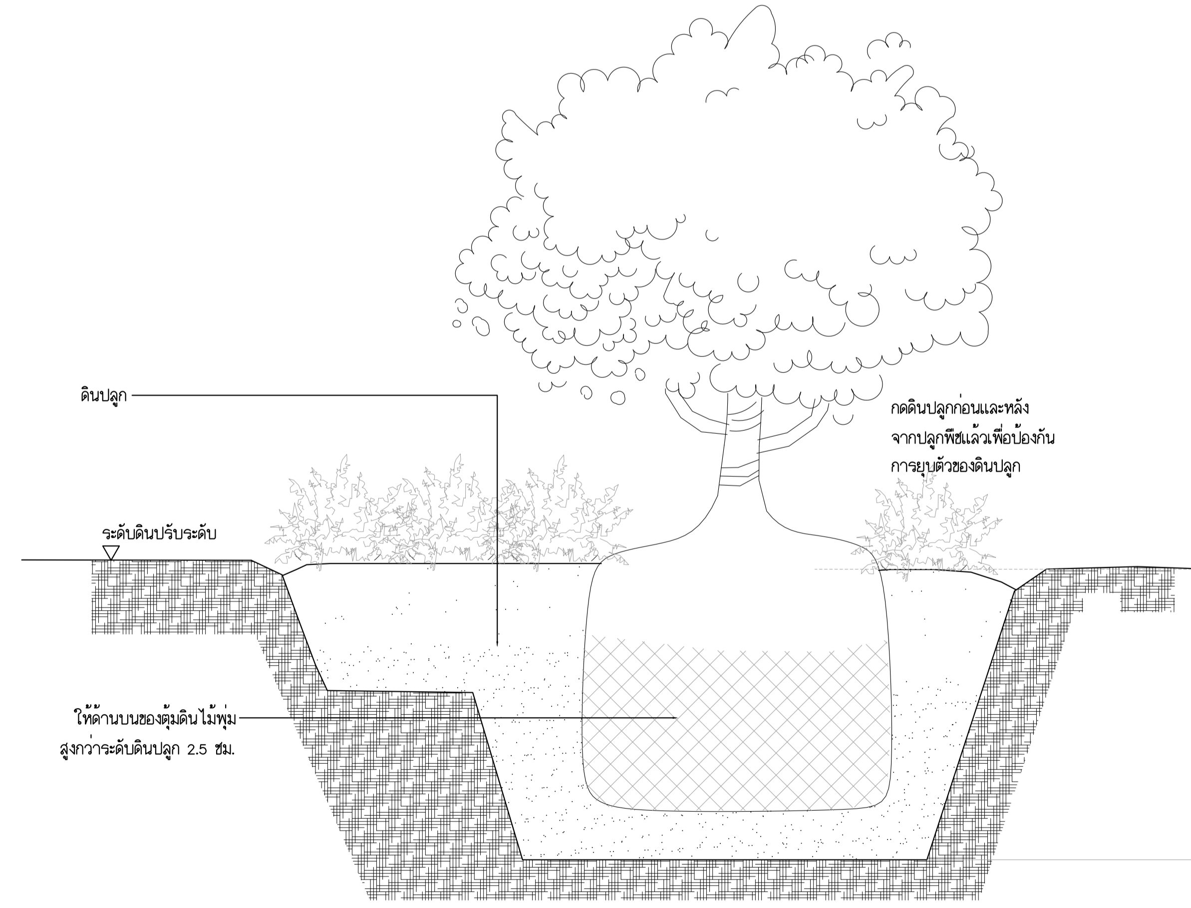
3 แบบขยายการปลูกไม้พุ่ม - ไม้คลุมดิน LA-02.2 มาตรฐาน 1 : 25
