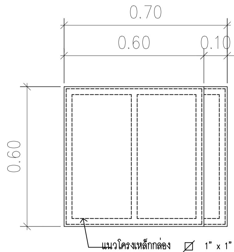
F - 1 SIDE TABLE ( เฟอร์นิเจอร์ลอยตัว ) - โครงเหล็กกล่อง 1" x 1" - กุ๊ไม้ HMR 9 มม - ปิดผิวลามิเนต L-M-4
