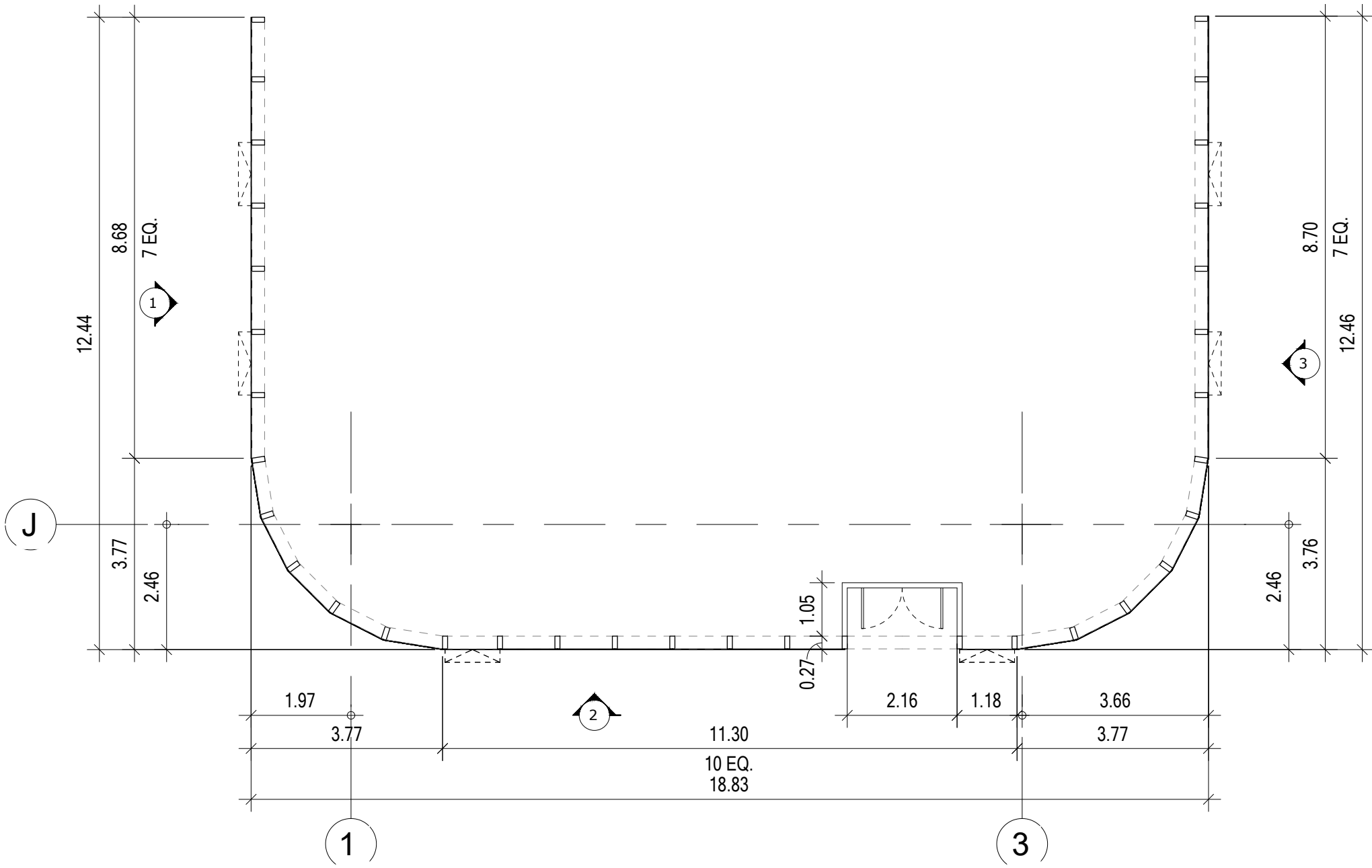
CW5 PLAN มาตราส่วน 1 : 100
