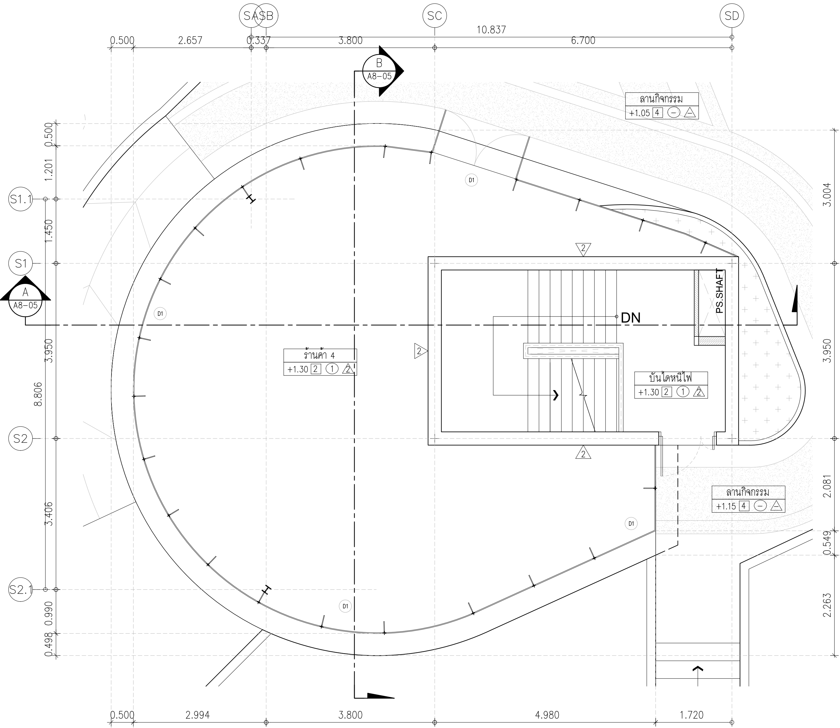
ผังพื้นที่ร้านค้า 4 มาตราส่วน 1:50
