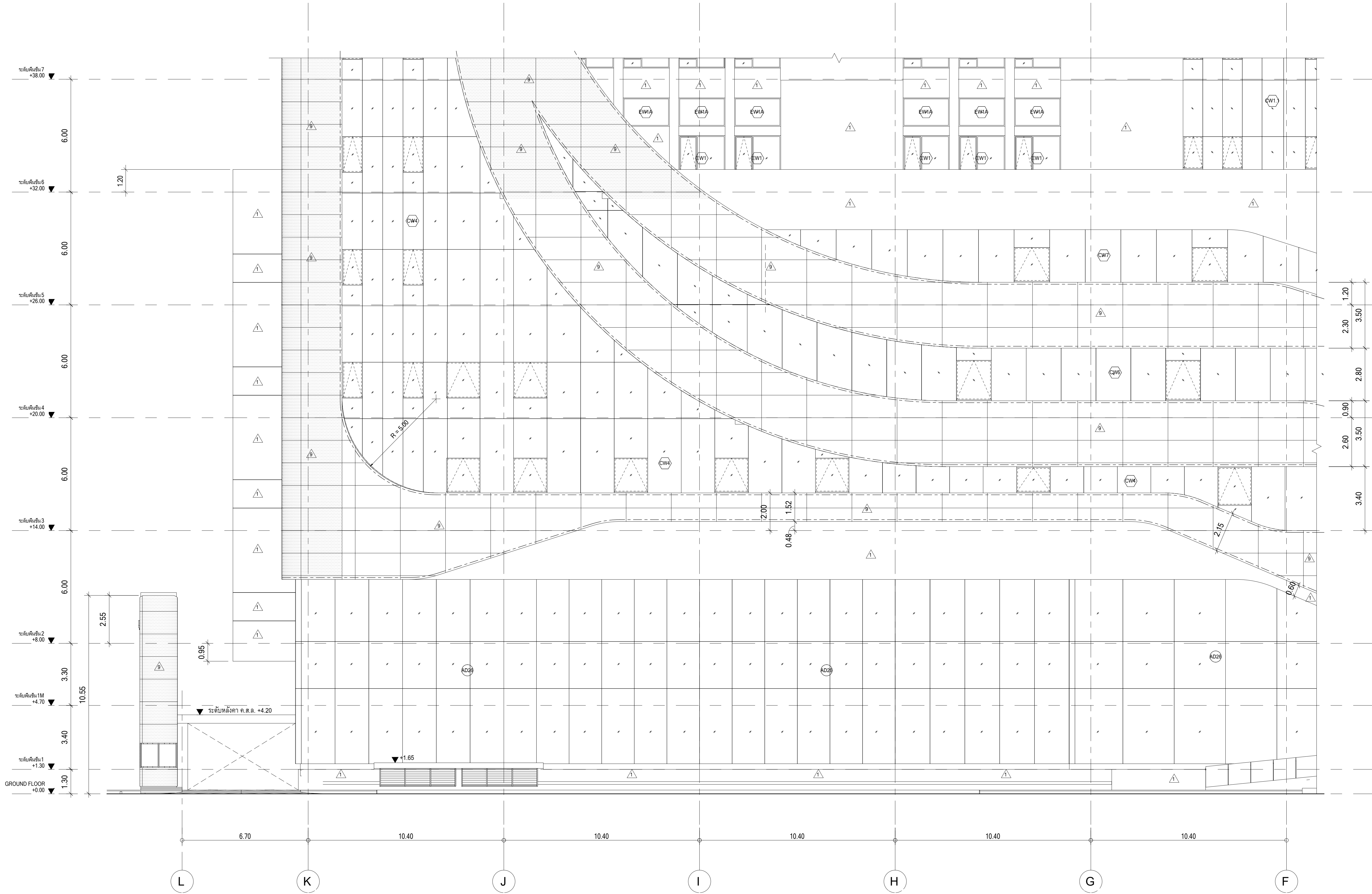
รูปด้านอาคาร 2, ส่วนที่ 1 มาตราส่วน 1 : 100
