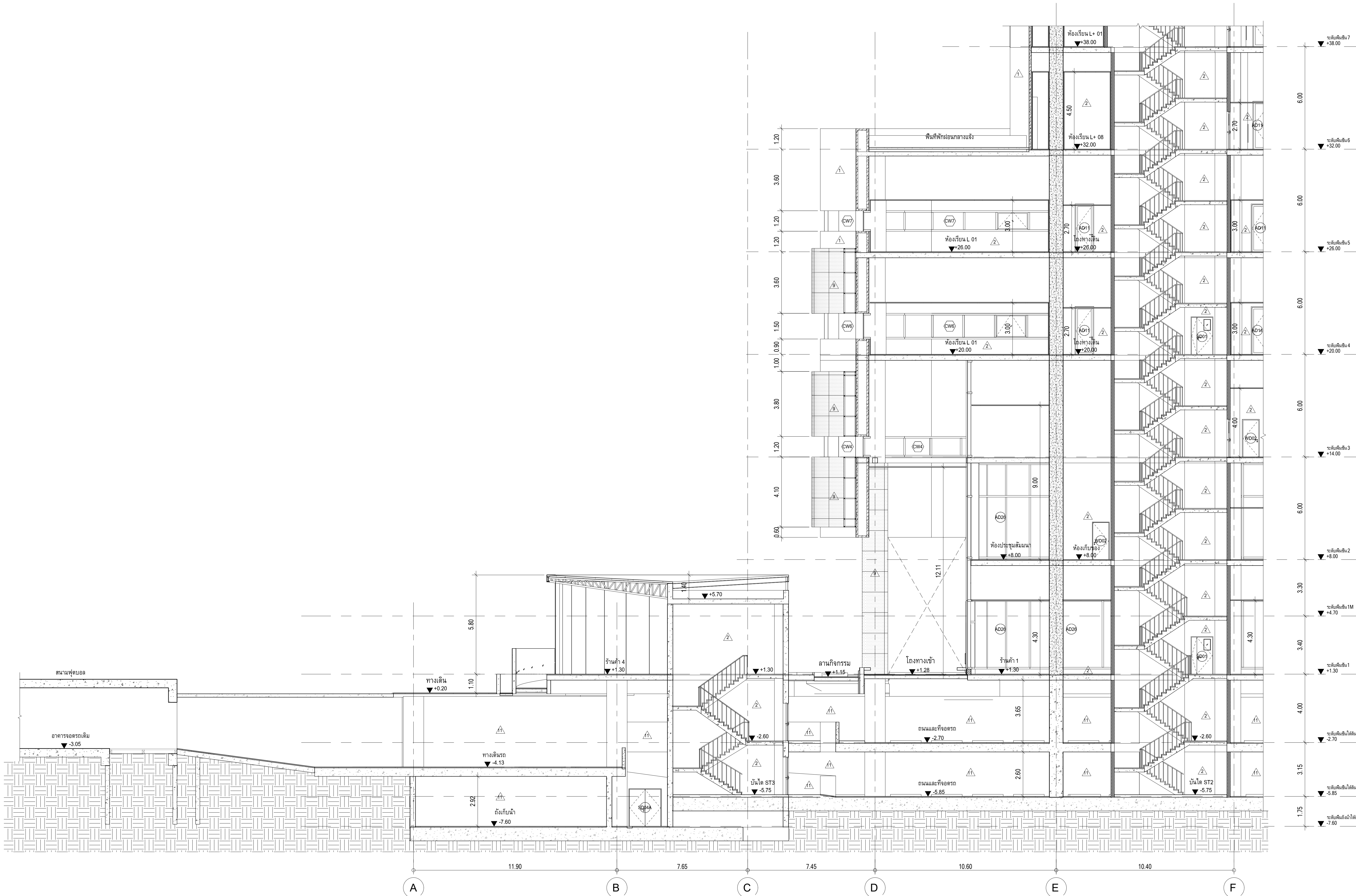
รูปตัดอาคารแนว A-A, ส่วนที่ 1 มาตราส่วน 1 : 100
