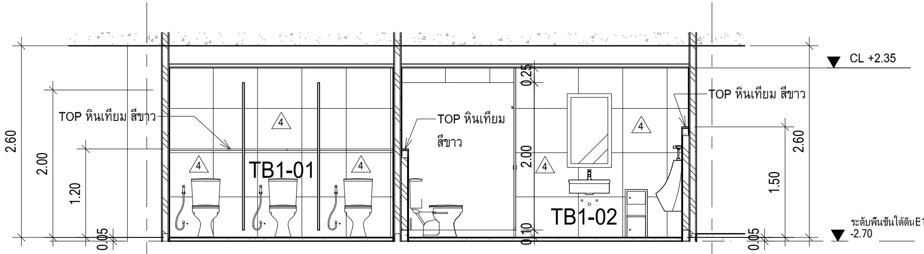
WC7 - รูปด้าน E01 มาตราส่วน 1 : 50
