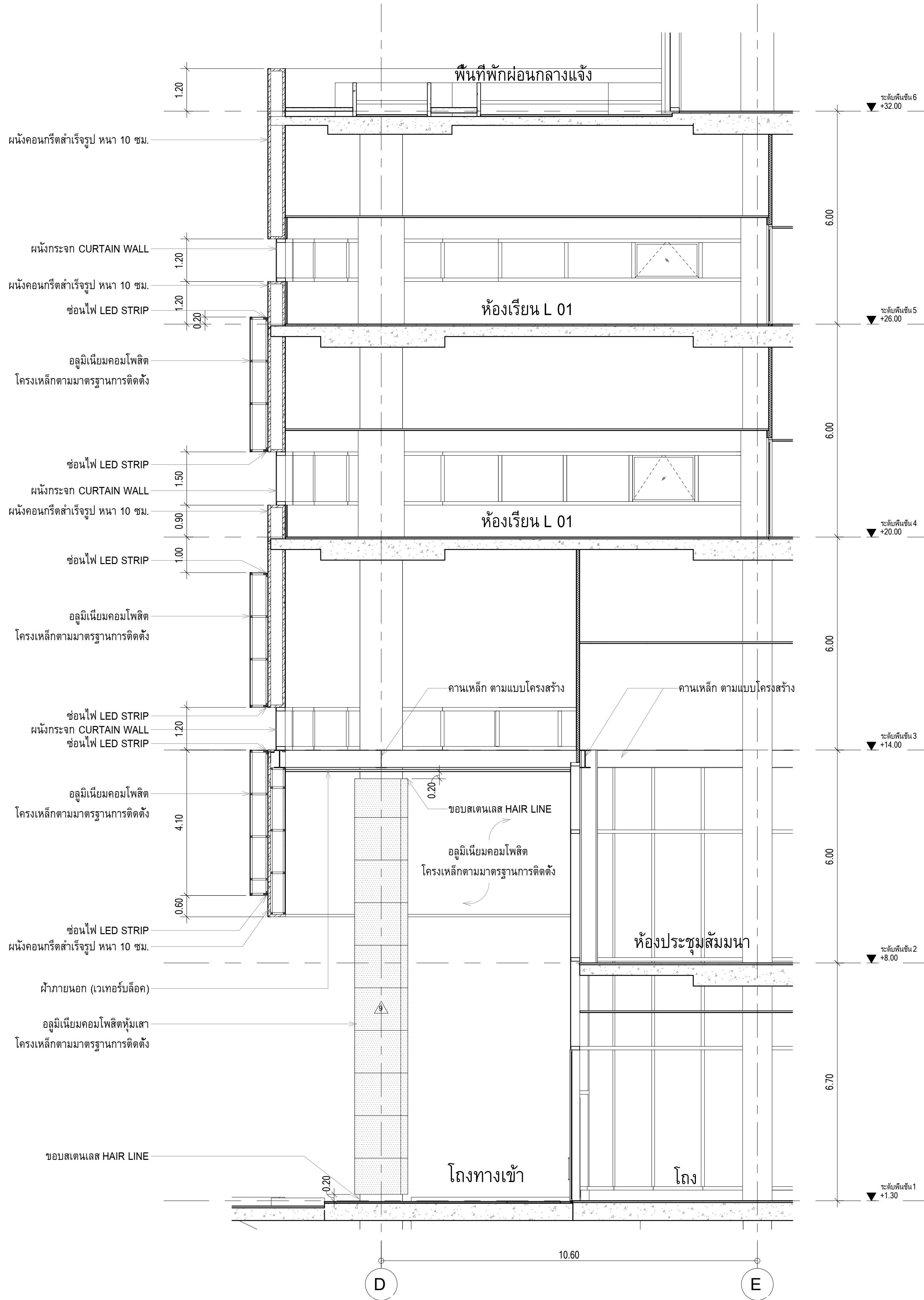
แบบขยายการติดตั้งผนังอลูมิเนียมคอมโพสิต มาตราส่วน 1 : 75
