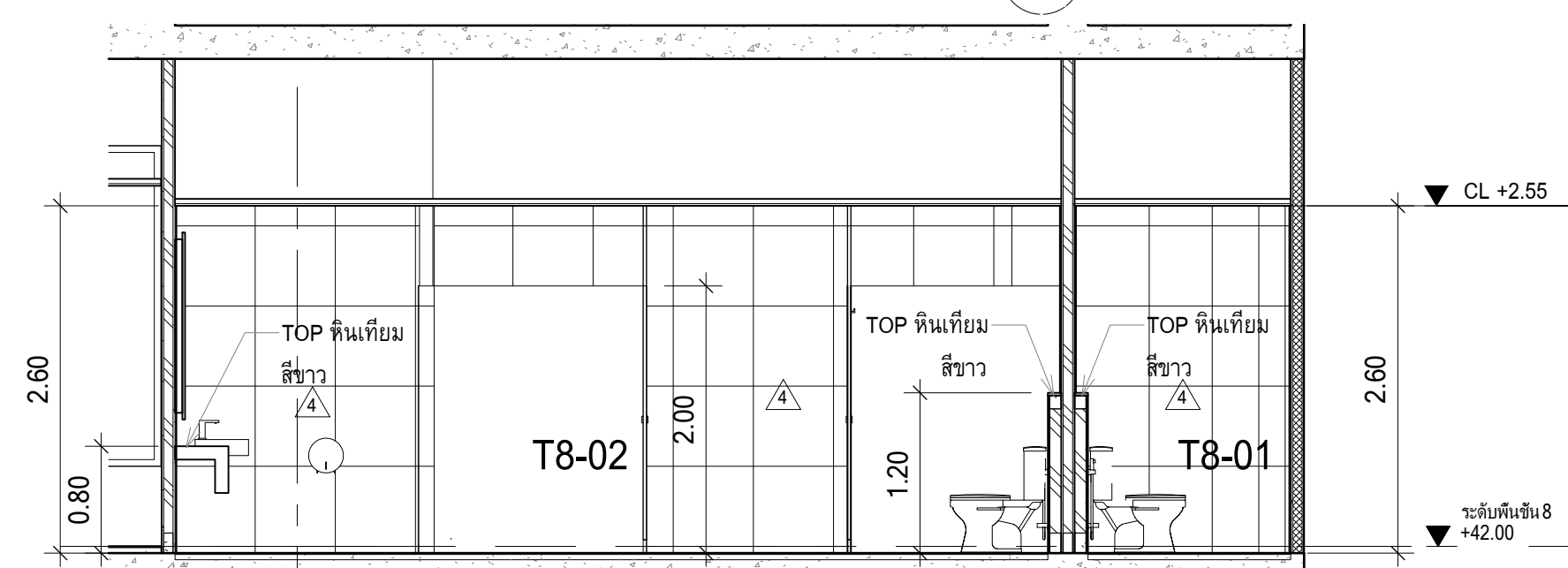
WC6 - รูปด้าน E07 มาตราส่วน 1 : 50
