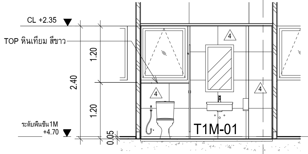
WC2 - รูปด้าน E03 มาตราส่วน 1 : 50
