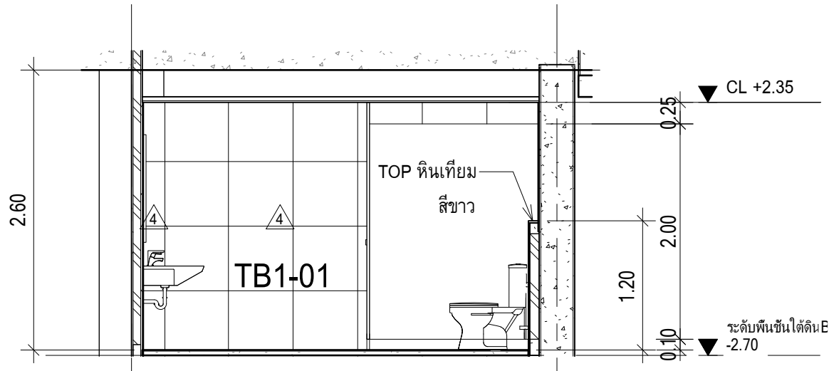
WC7 - รูปด้าน E01 มาตราส่วน 1 : 50
