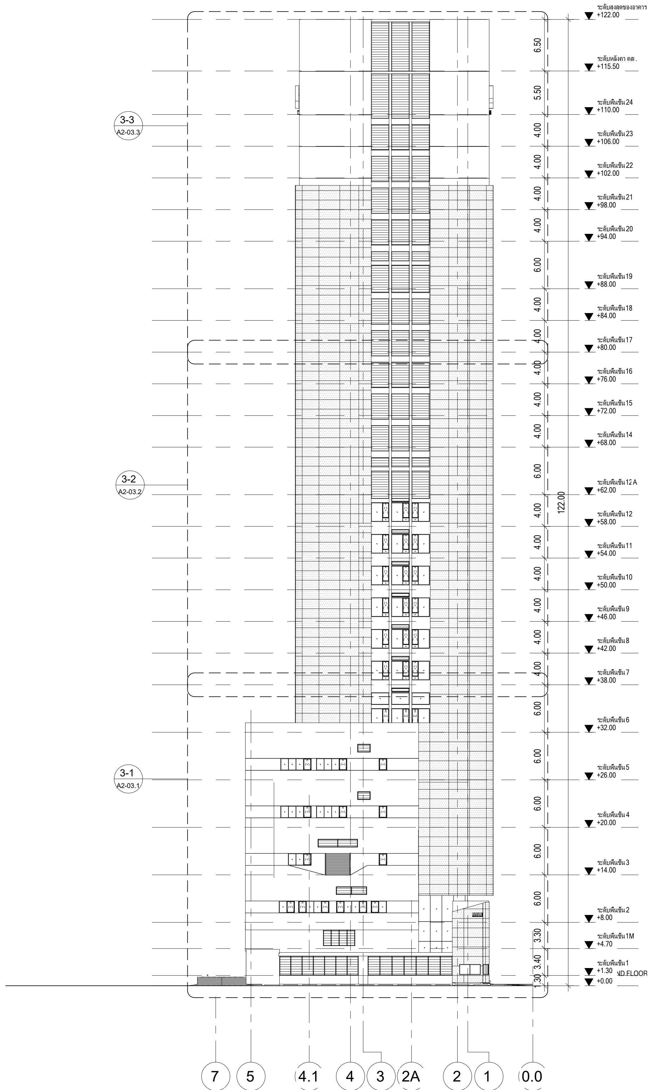
รูปด้านอาคาร 3 มาตราส่วน 1 : 300
