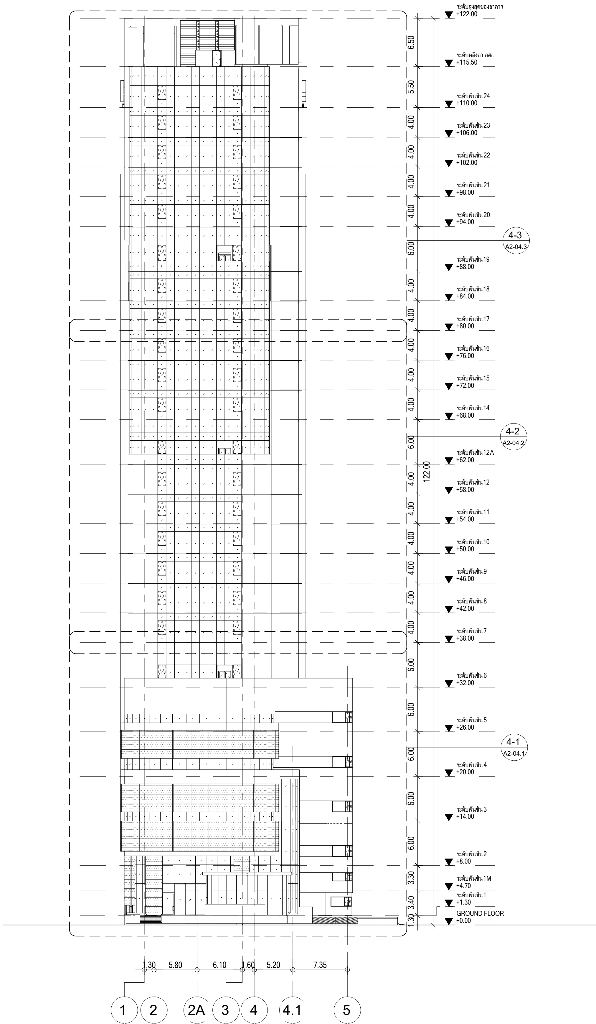
รูปด้านอาคาร 4 มาตราส่วน 1 : 300
