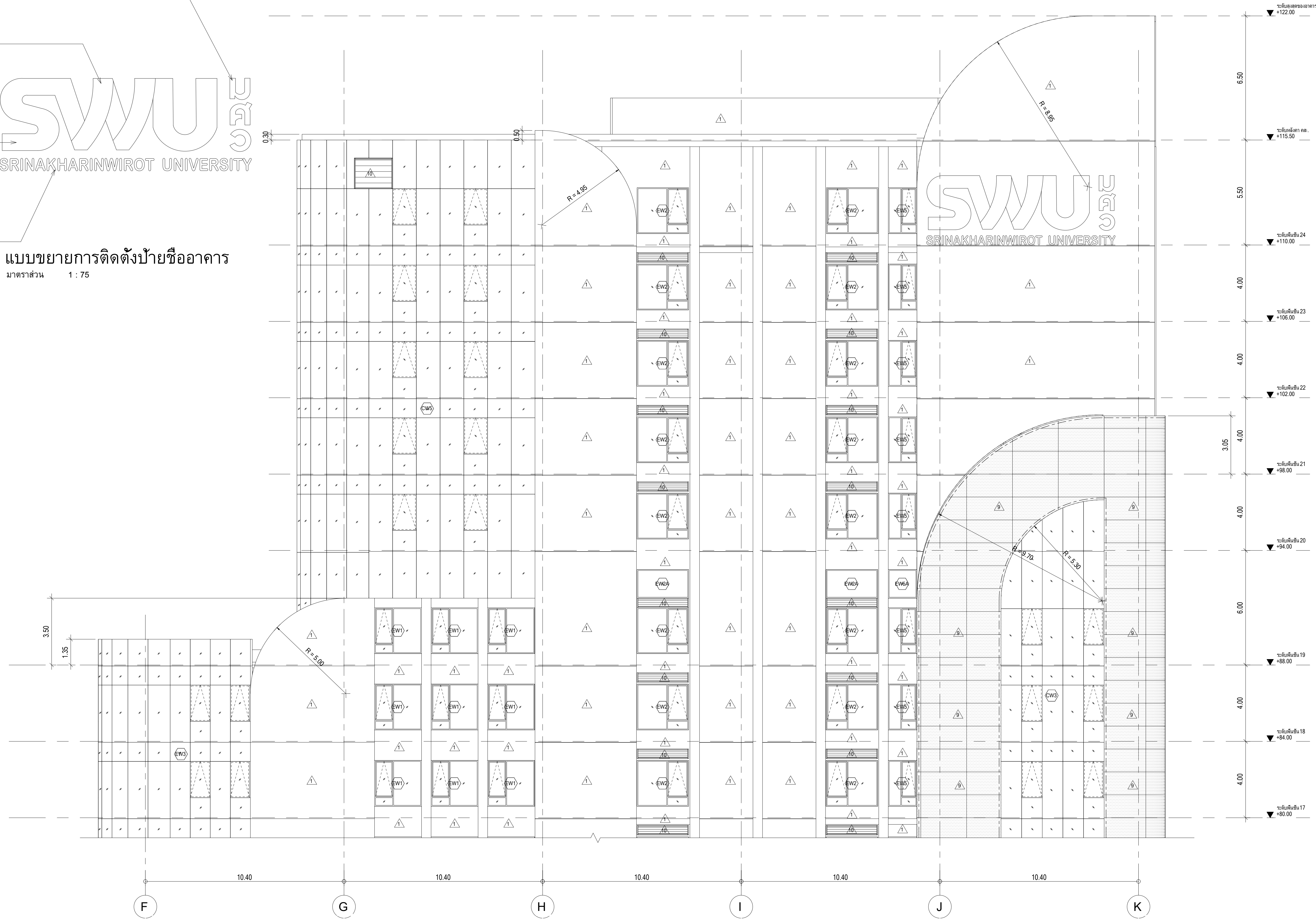
รูปด้านอาคาร 1, ส่วนที่ 4 มาตราส่วน 1 : 100
