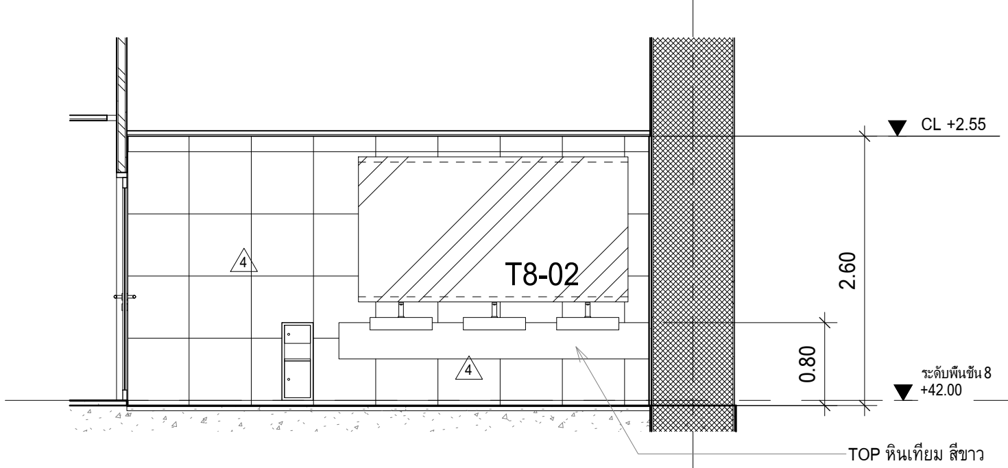
WC6 - รูปด้าน E01 มาตราส่วน 1 : 50
