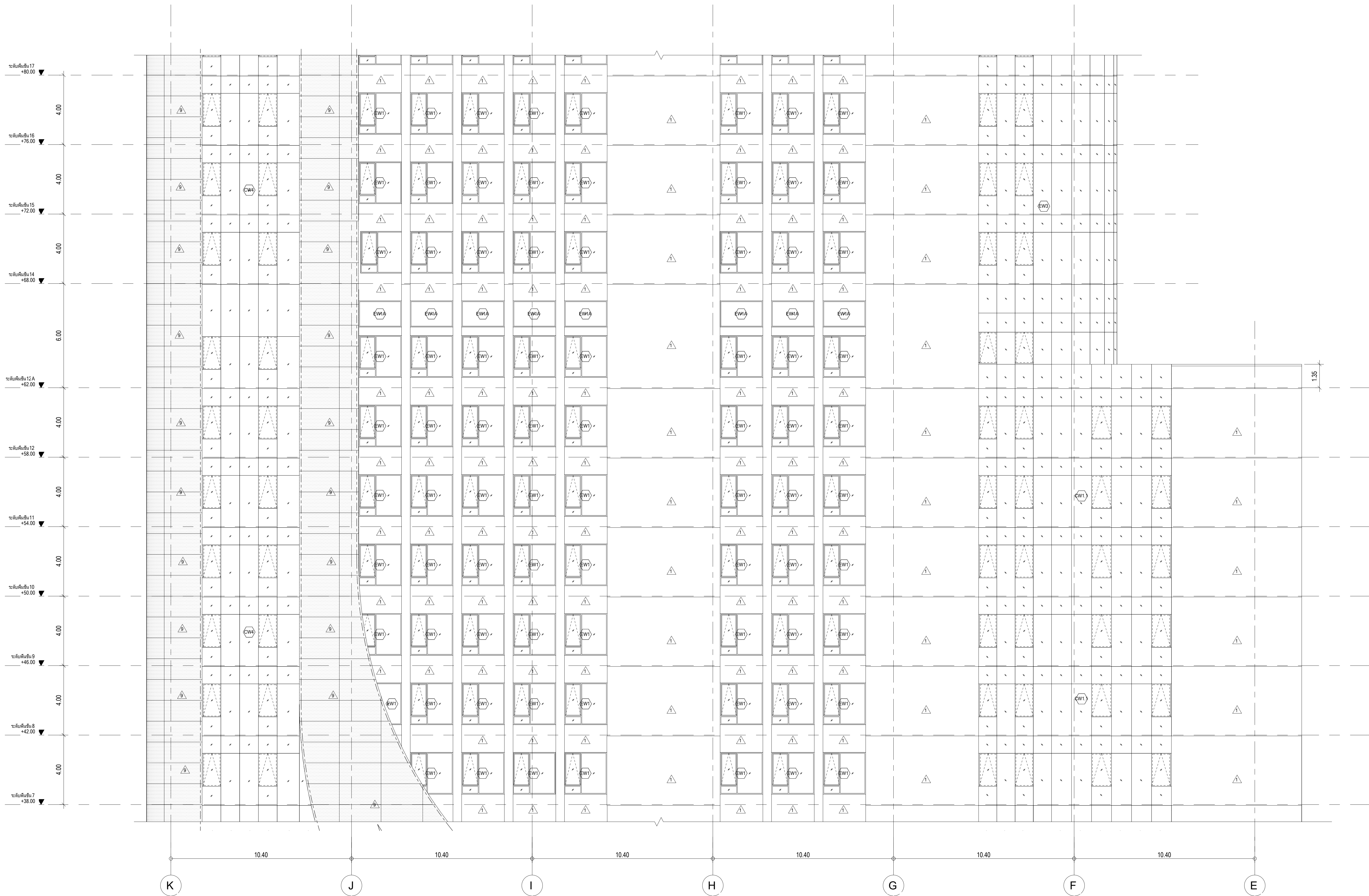
รูปด้านอาคาร 2, ส่วนที่ 3 มาตราส่วน 1 : 100
