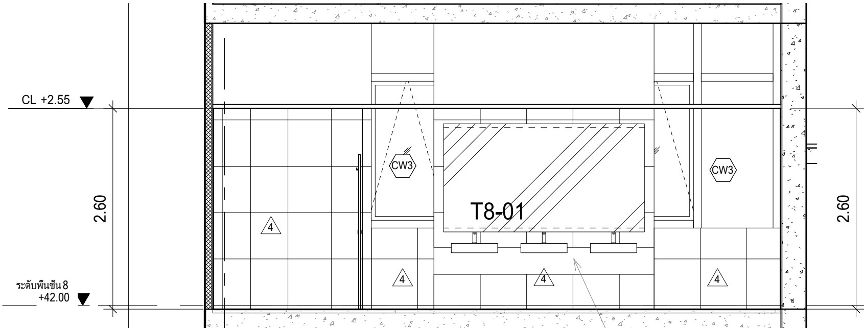
WC6 - รูปด้าน E03 มาตราส่วน 1 : 50
