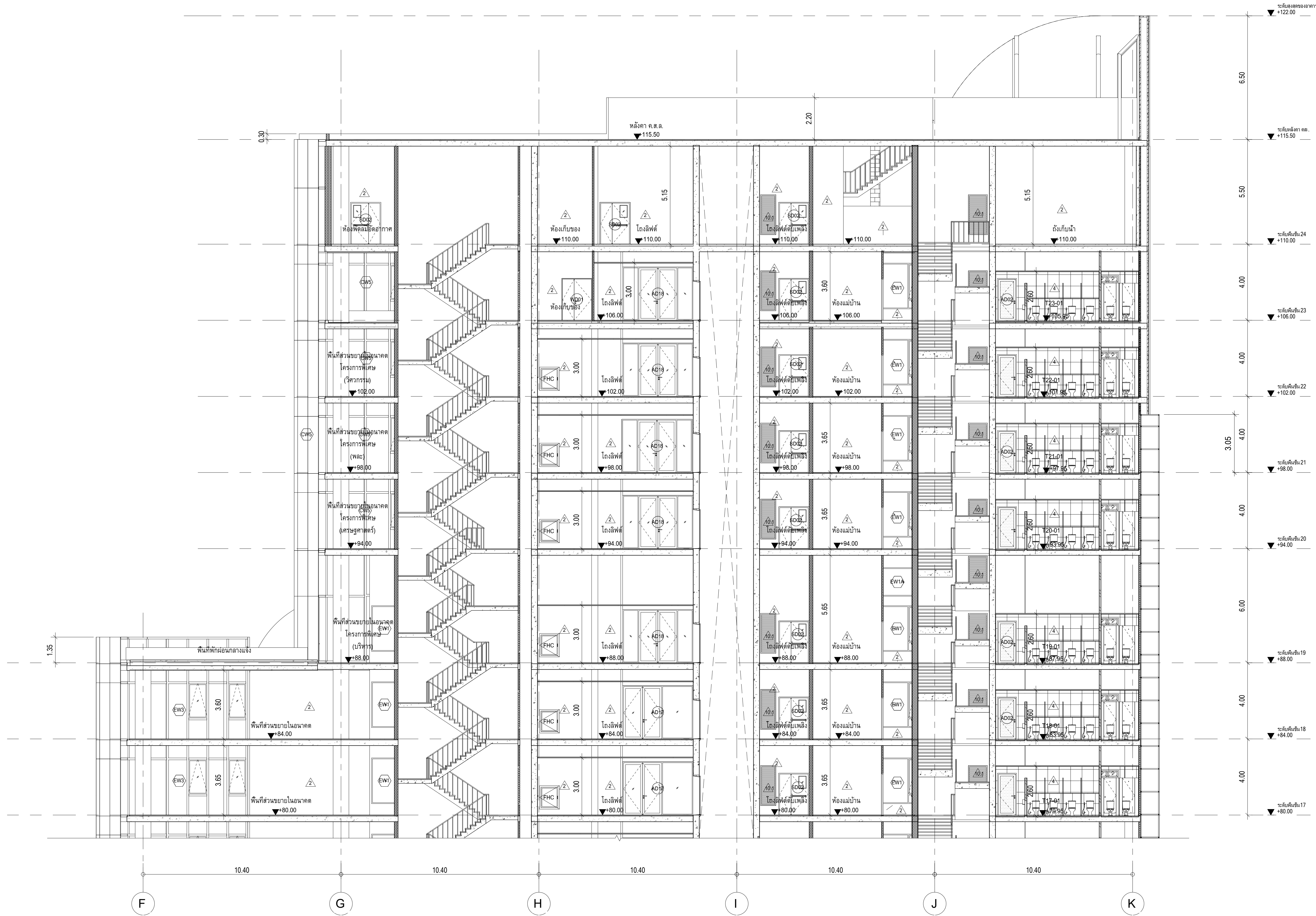
รูปตัดอาคารแนว A-A, ส่วนที่ 4 มาตราส่วน 1 : 100
