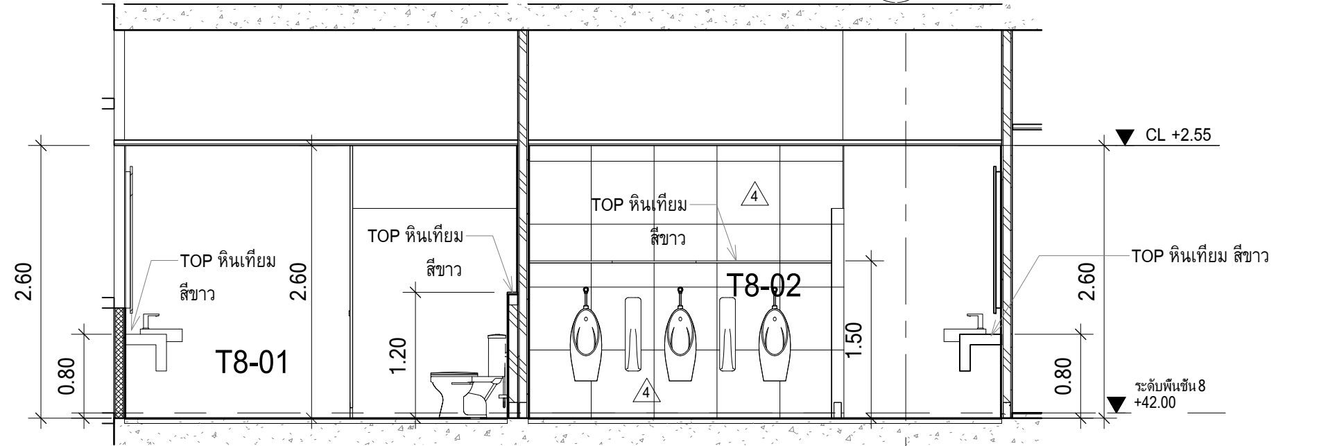
WC6 - รูปด้าน E06 มาตราส่วน 1 : 50
