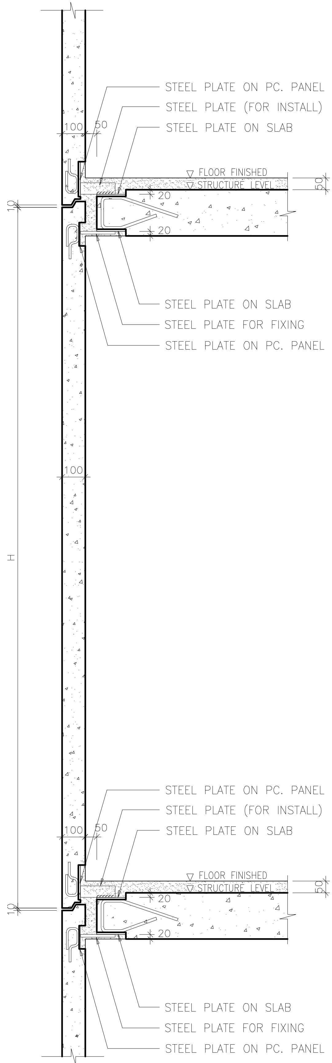
TYPICAL SECTION OF PC. FOR FLOOR TO FLOOR มาตราส่วน 1 : 10
