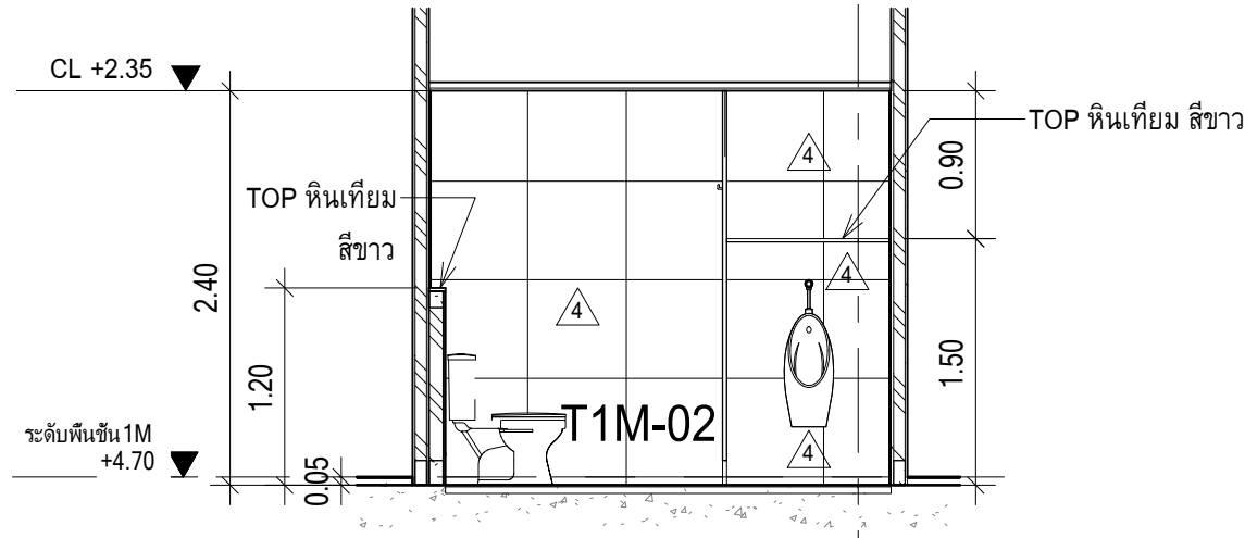
WC2 - รูปด้าน E02 มาตราส่วน 1 : 50
