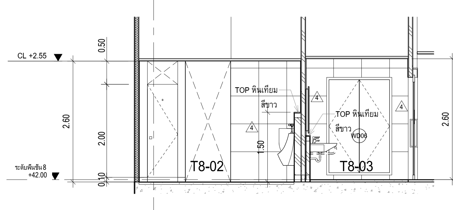
WC6 - รูปด้าน E02 มาตราส่วน 1 : 50
