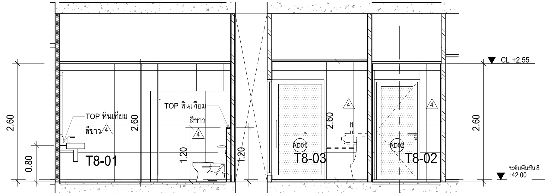
WC6 - รูปด้าน E04 มาตราส่วน 1 : 50
