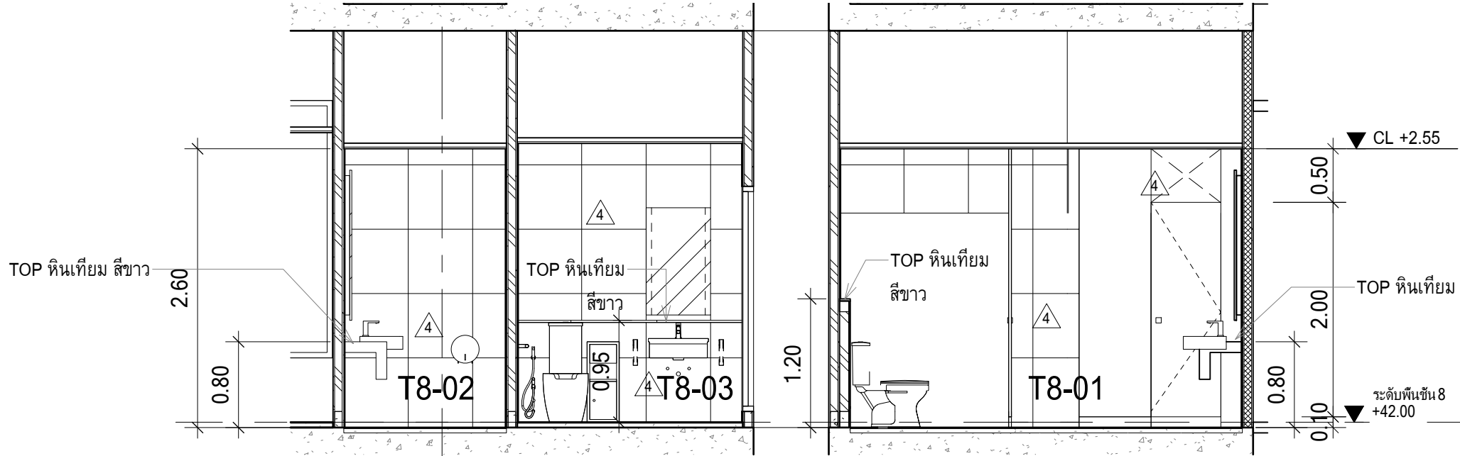
WC6 - รูปด้าน E05 มาตราส่วน 1 : 50
