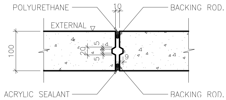
DETAIL OF VERTICAL JOINT SEALANT มาตราส่วน 1 : 5
