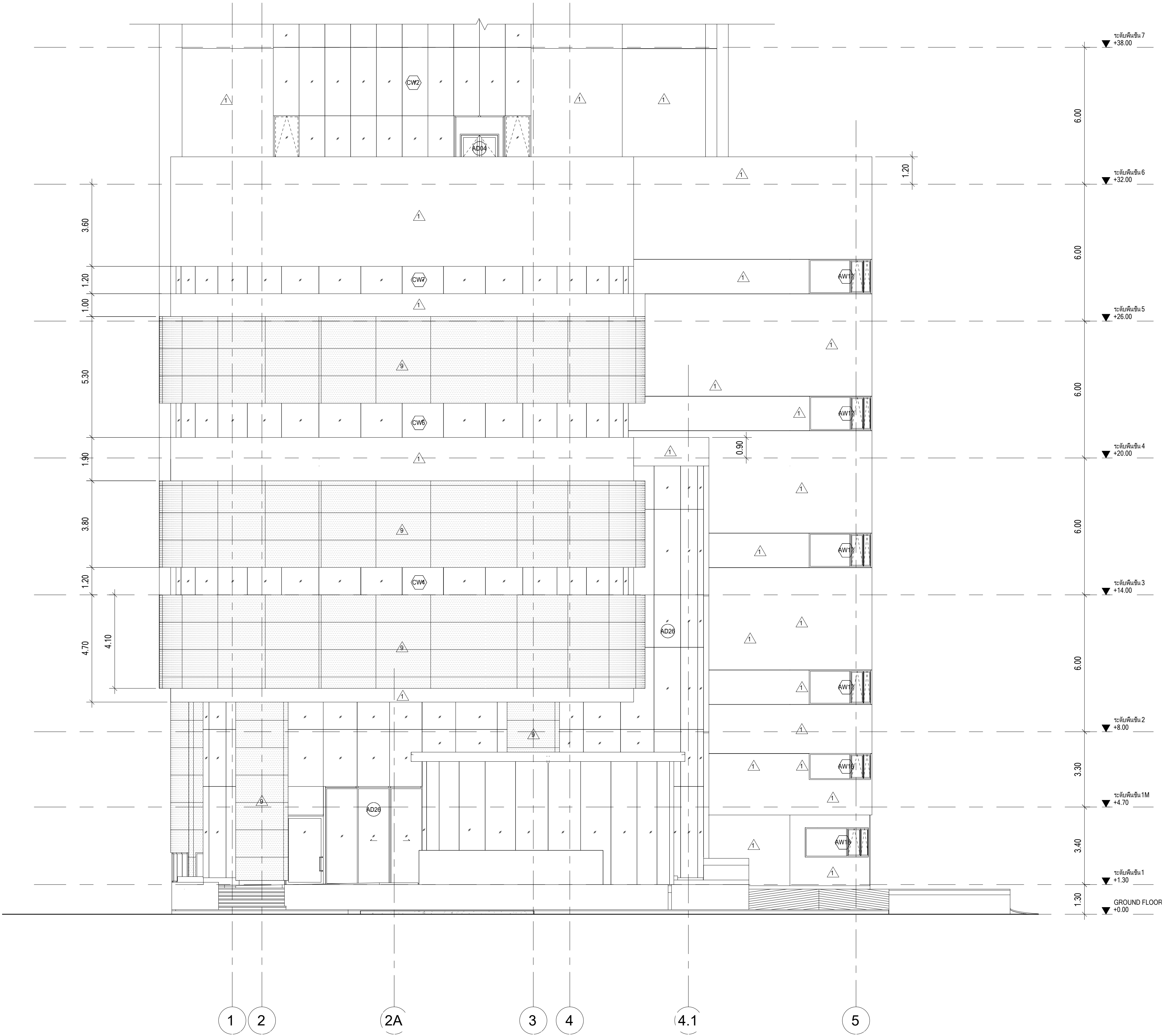
รูปด้านอาคาร 4, ส่วนที่ 1 มาตราส่วน 1 : 100
