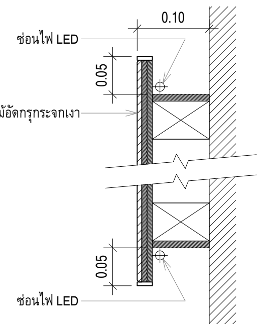
SECTION แบบขยายการซ่อนไฟที่กระจกเงา มาตราส่วน 1 : 5
