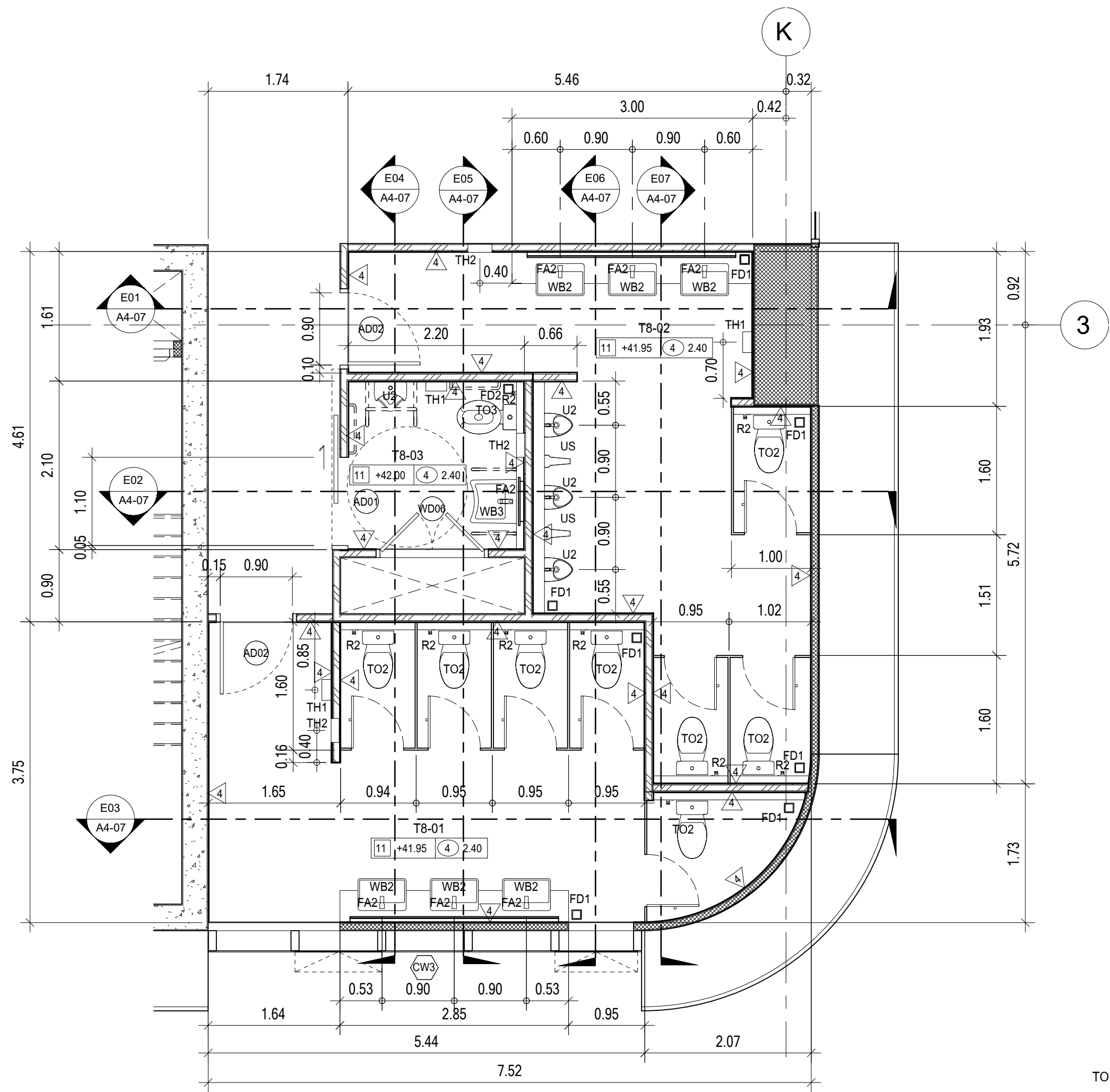
WC6 - แปลน มาตราส่วน 1 : 50
