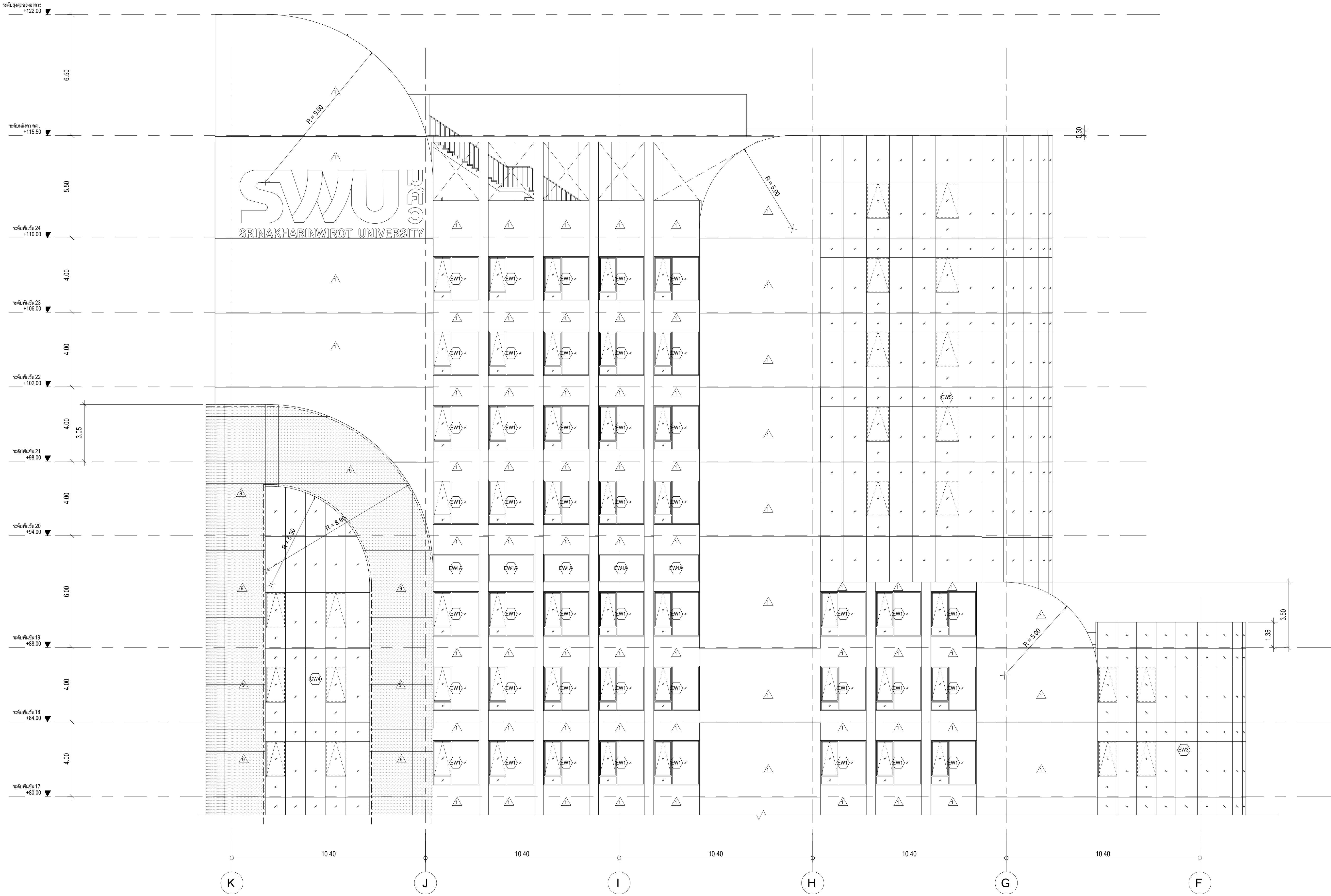
รูปด้านอาคาร 2, ส่วนที่ 4 มาตราส่วน 1 : 100
