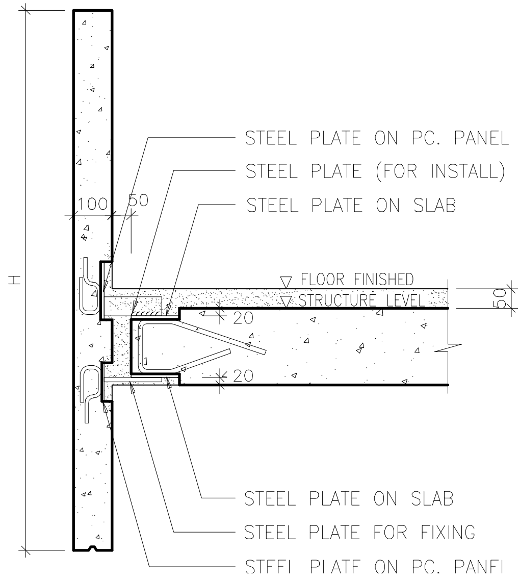
TYPICAL SECTION OF PC. PARAPET มาตราส่วน 1 : 10
