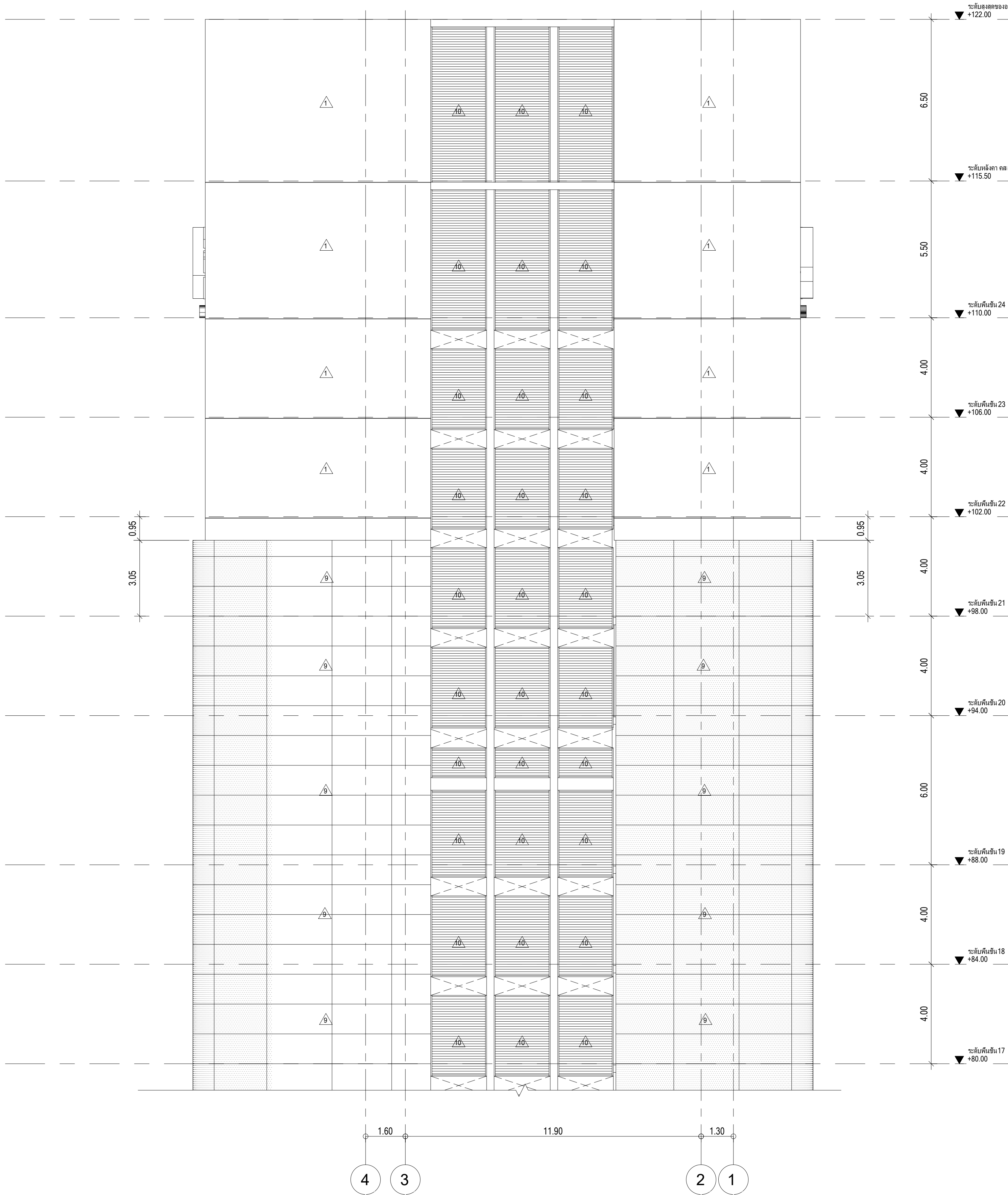
รูปด้านอาคาร 3, ส่วนที่ 3 มาตราส่วน 1 : 100
