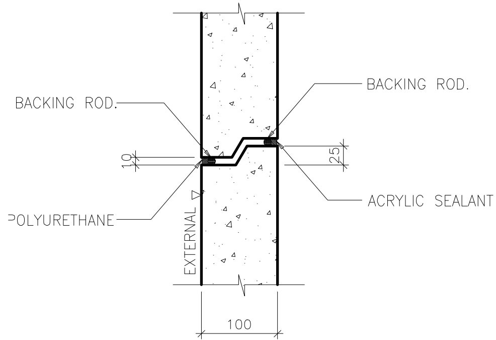
DETAIL OF HORIZONTAL JOINT SEALANT มาตราส่วน 1 : 5
