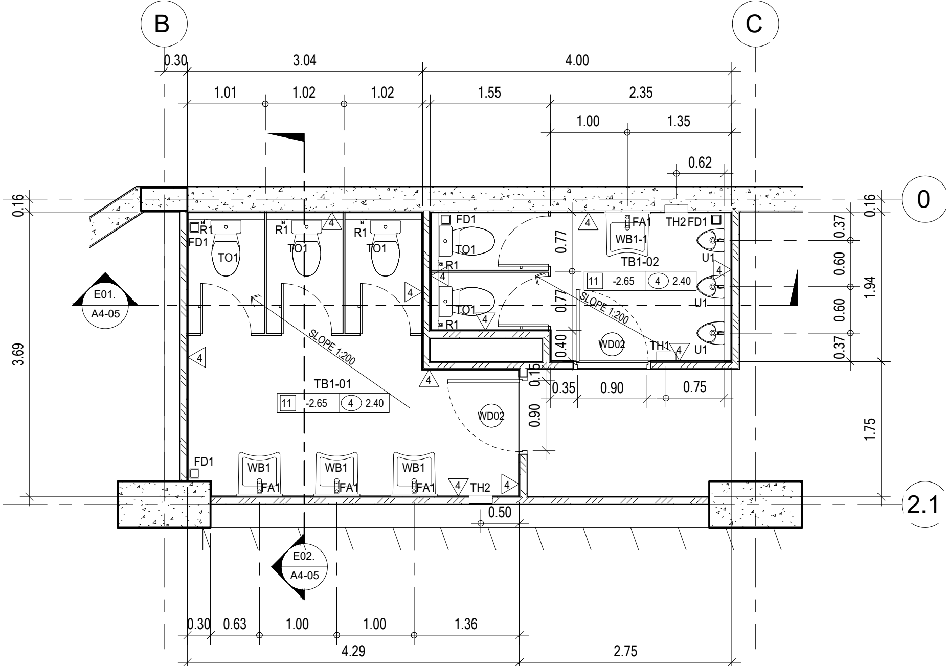
WC7 - แปลน มาตราส่วน 1 : 50
