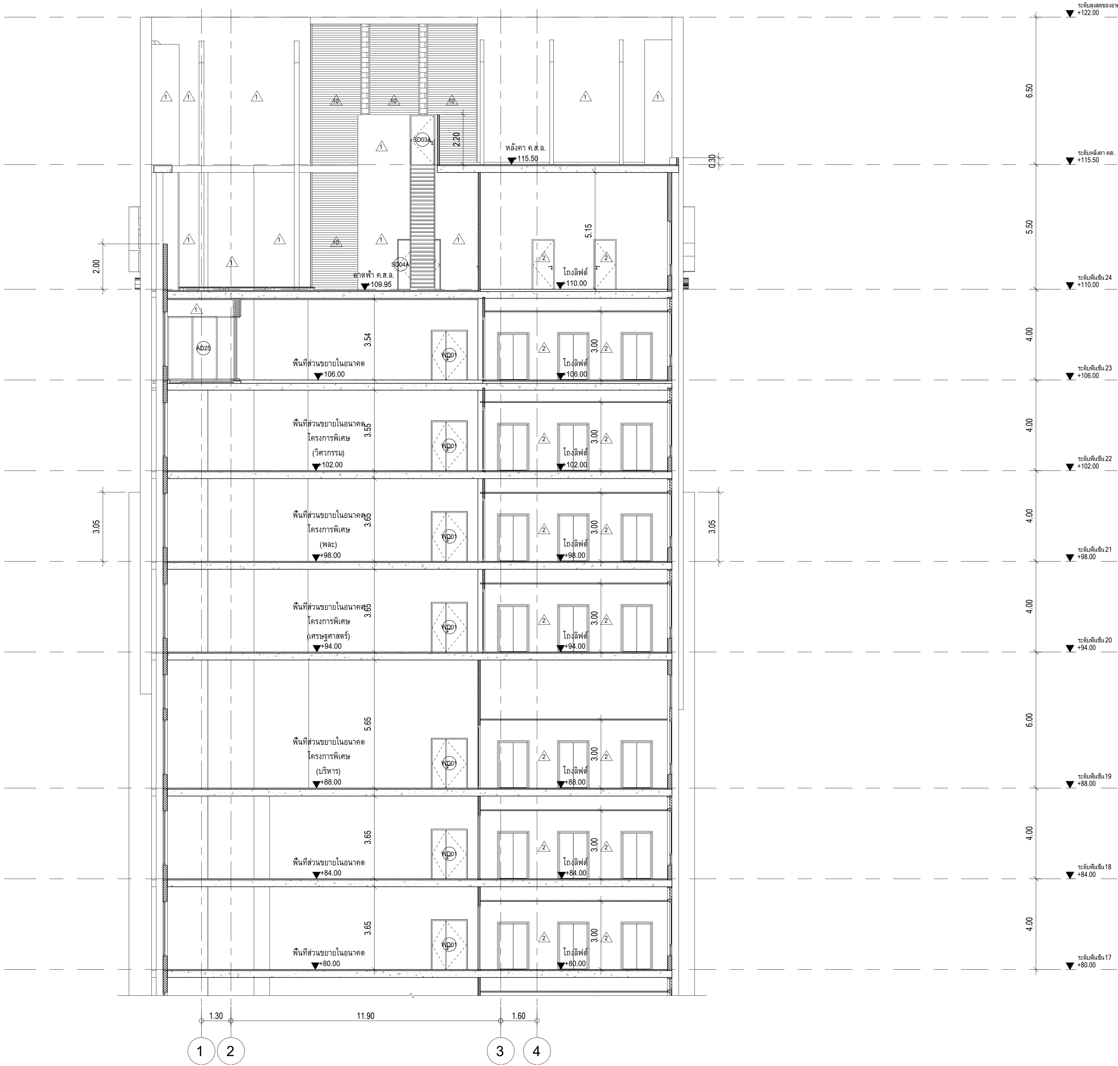
รูปตัดอาคารแนว C-C, ส่วนที่ 3 มาตราส่วน 1 : 100
