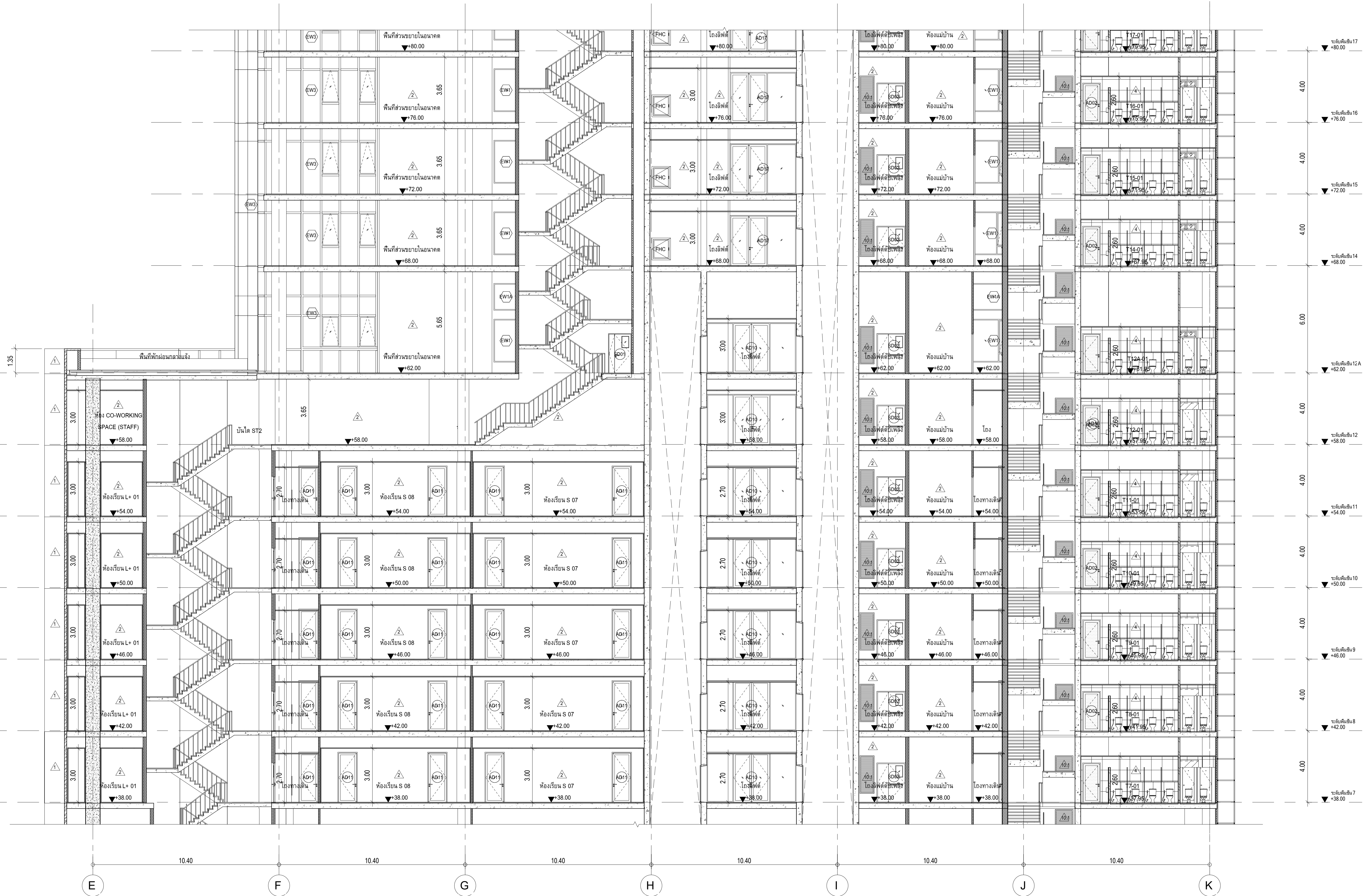
รูปตัดอาคารแนว A-A, ส่วนที่ 3 มาตราส่วน 1 : 100
