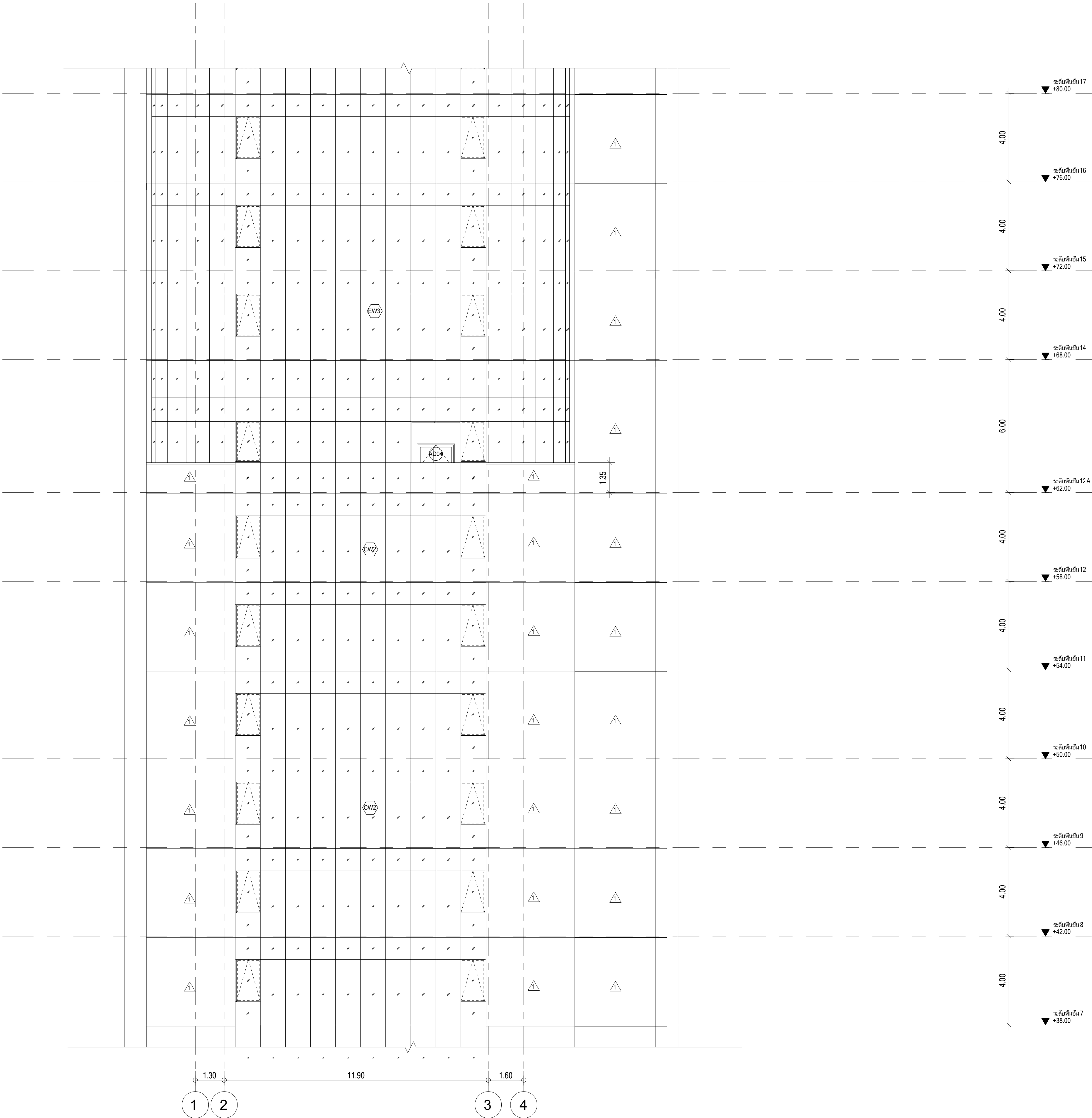
รูปด้านอาคาร 4, ส่วนที่ 2 มาตราส่วน 1 : 100
