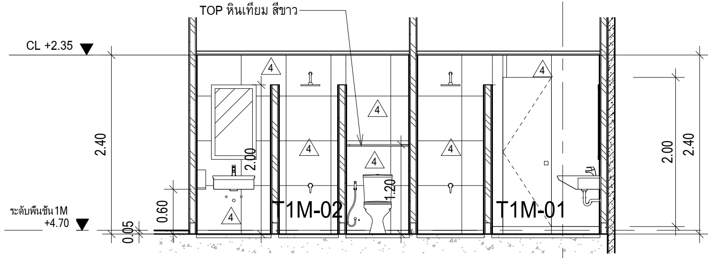
WC2 - รูปด้าน E01 มาตราส่วน 1 : 50
