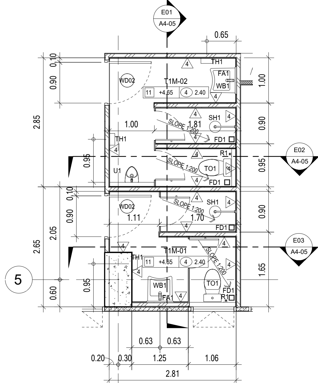
WC2 - แปลน มาตราส่วน 1 : 50
