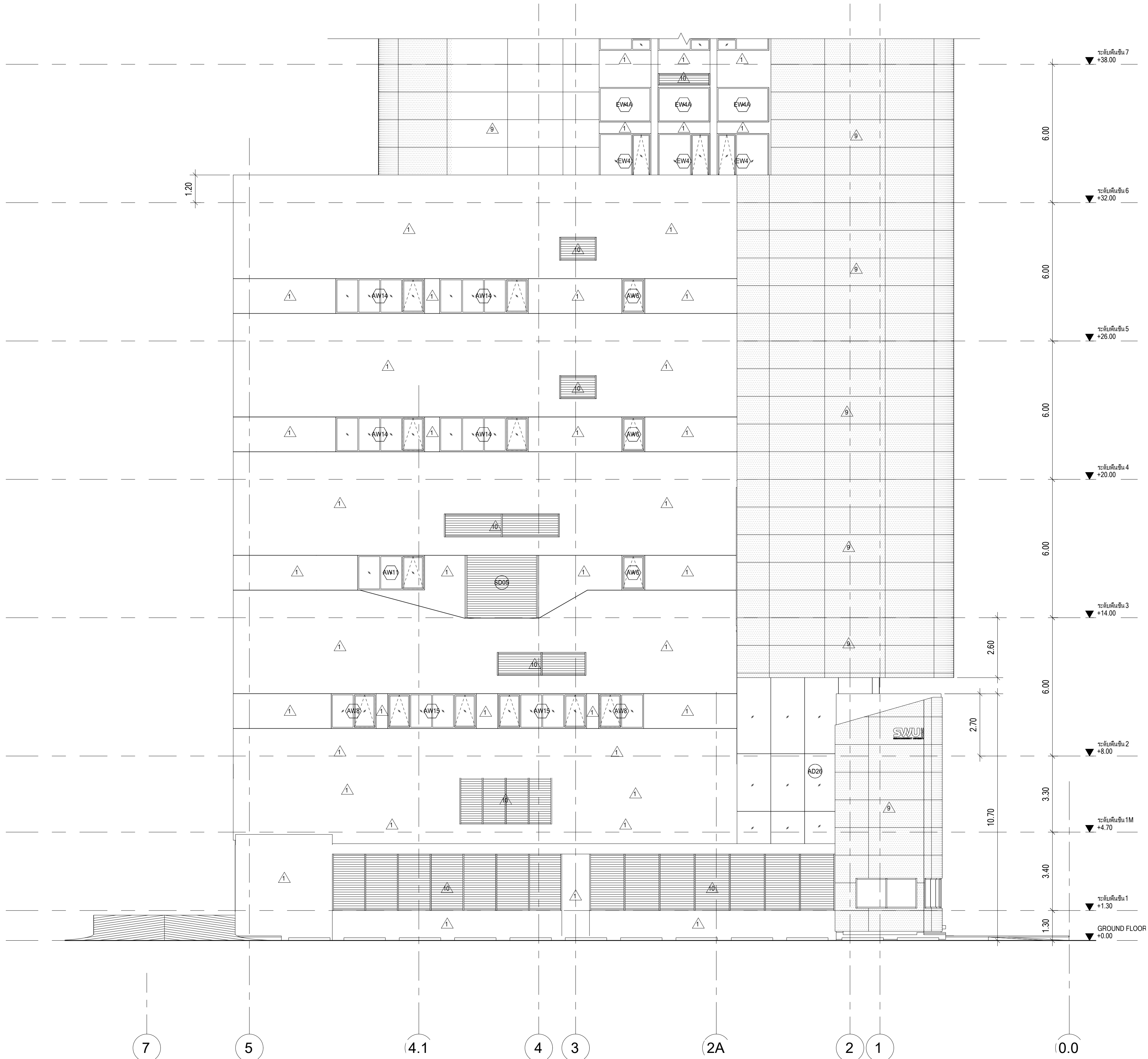
รูปด้านอาคาร 3, ส่วนที่ 1 มาตราส่วน 1 : 100
