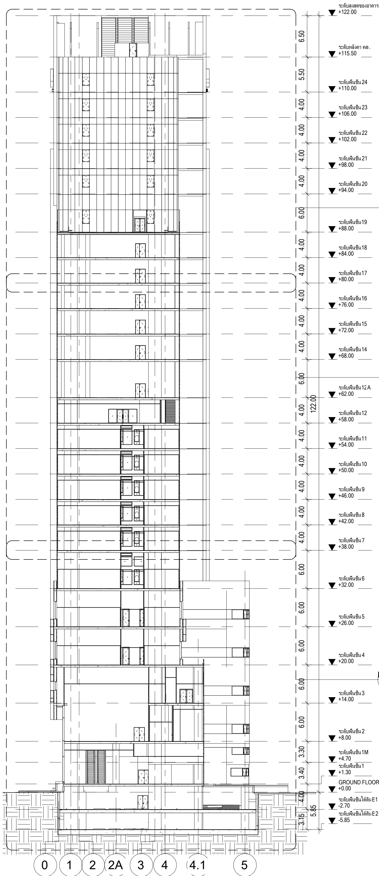
รูปตัดอาคารแนว B-B มาตราส่วน 1 : 300
