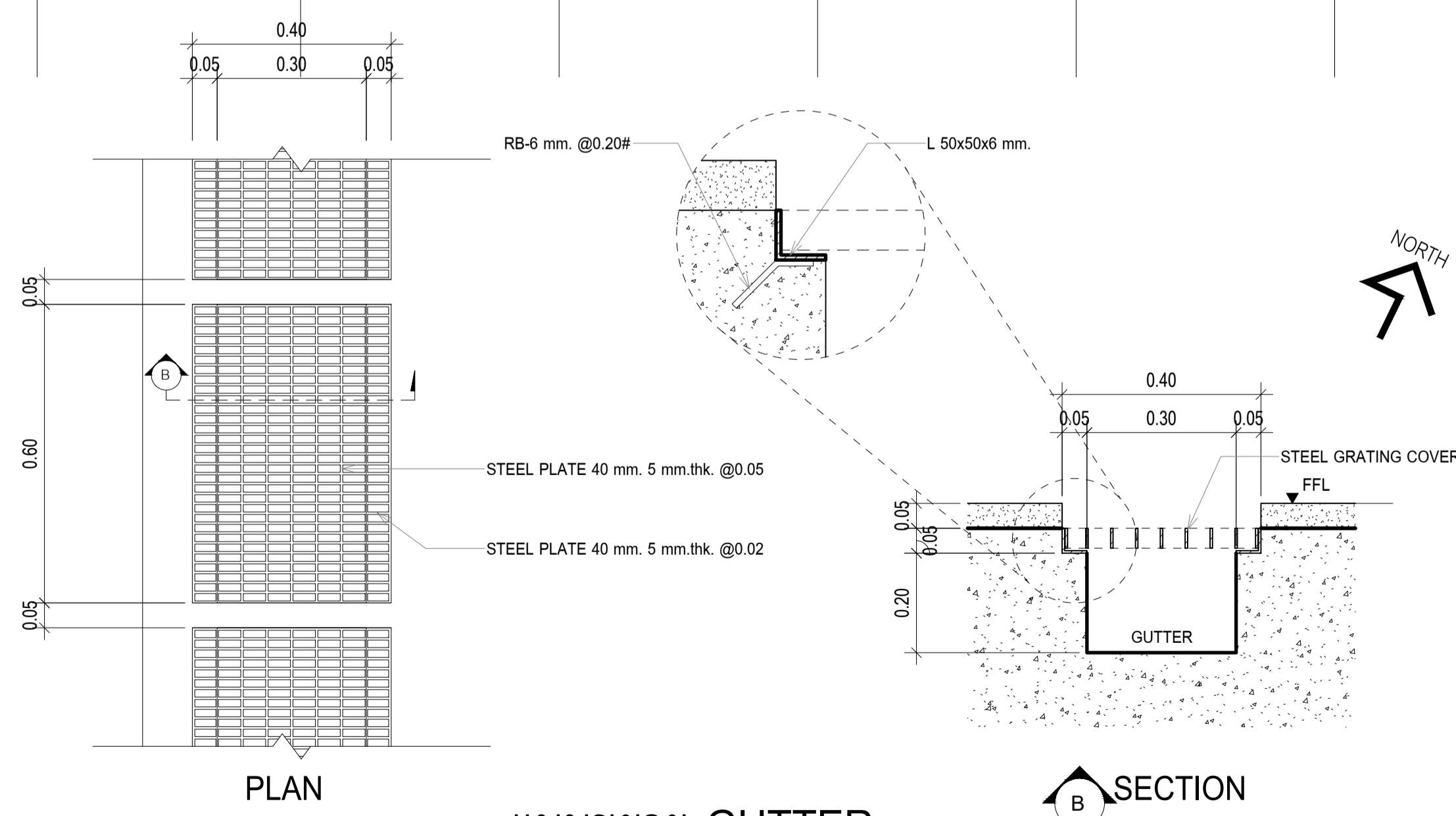
แบบขยาย GUTTER มาตรฐาน 1 : 10
