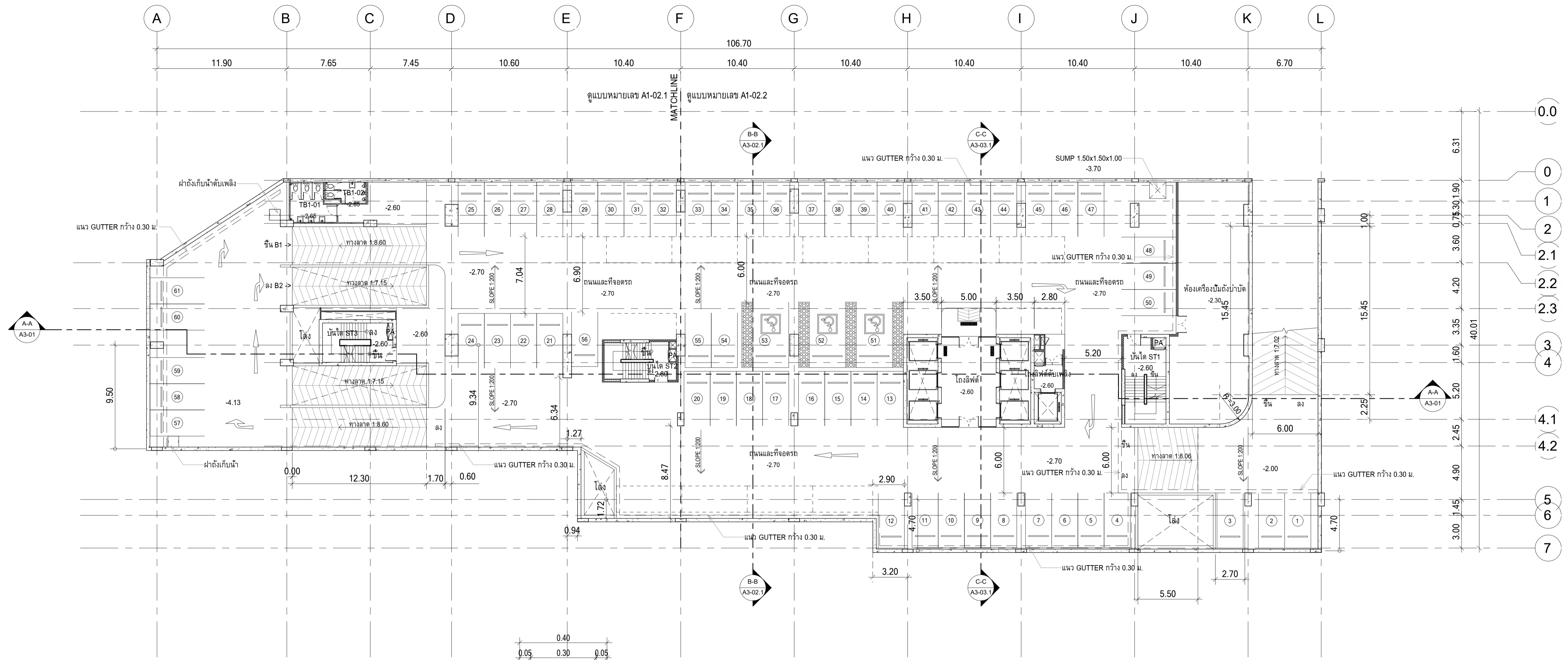
ผังพื้นชั้นใต้ดิน B1 มาตราส่วน 1 : 200
