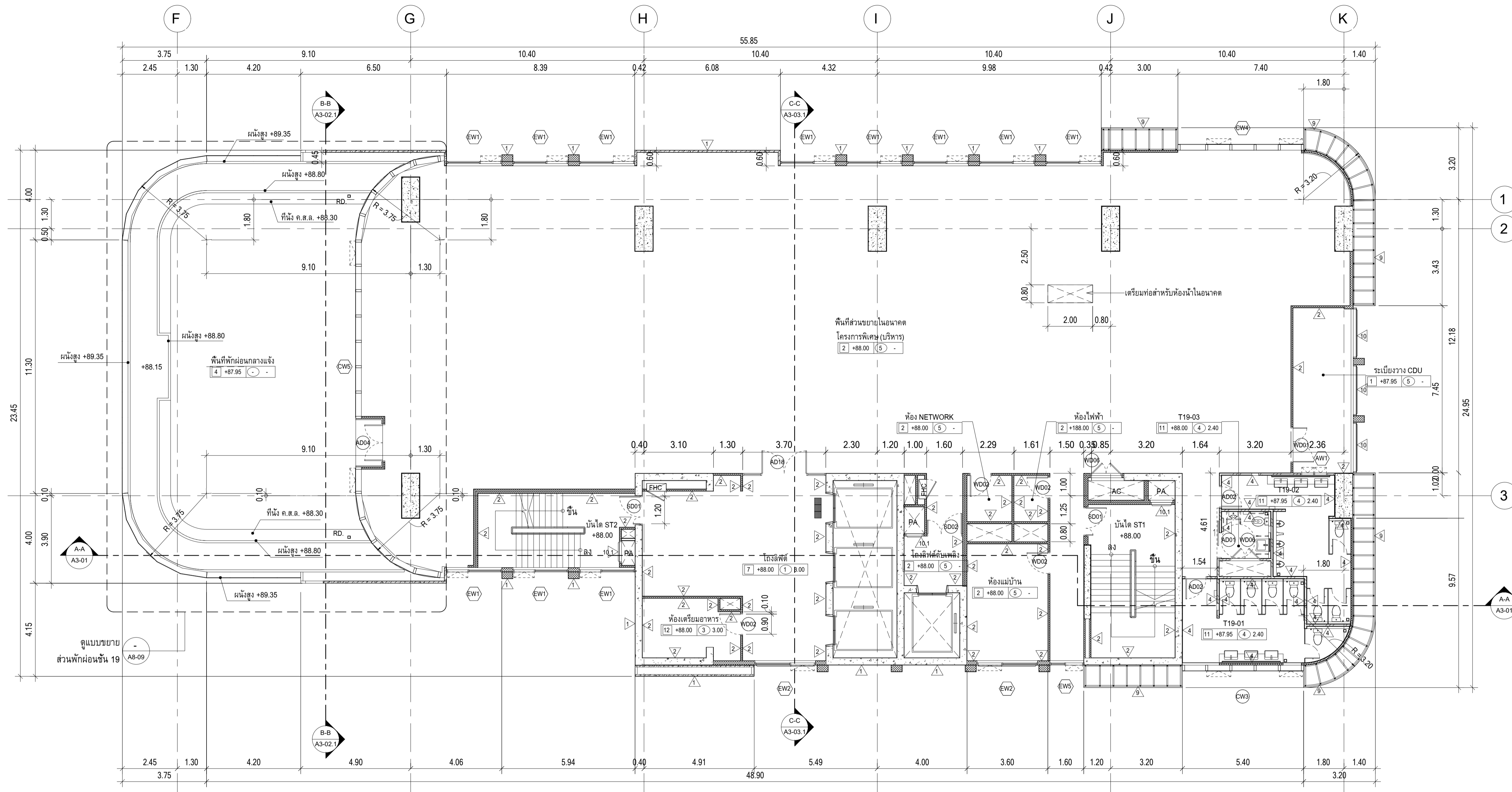
ผังพื้นชั้น 19 มาตรฐาน 1 : 100
