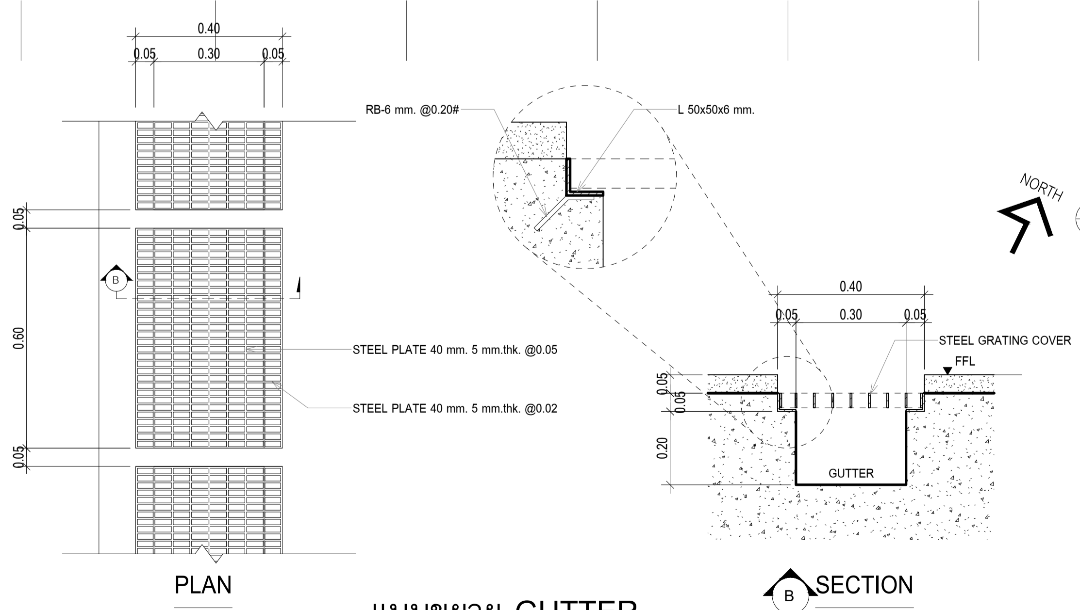
แบบขยาย GUTTER มาตราส่วน 1 : 10
