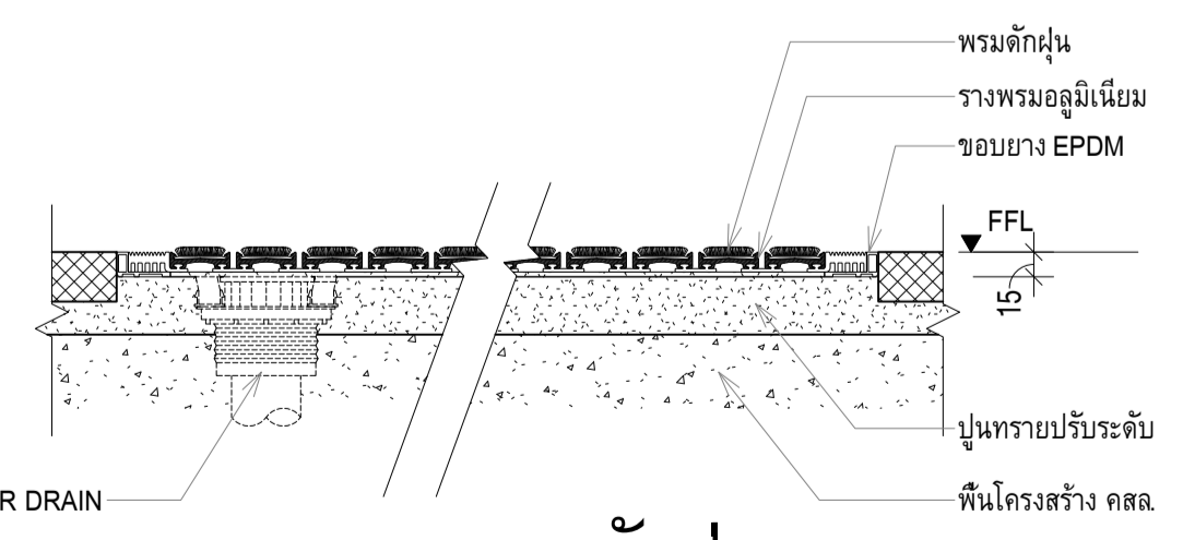
แบบขยายพรมดักฝุ่น มาตราส่วน 1 : 5
