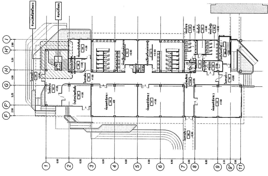
ชั้นที่ 3 SCALE 1:200
