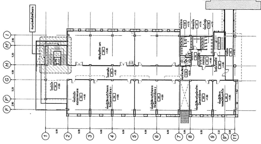
ชั้นที่ 2 SCALE 1:200
