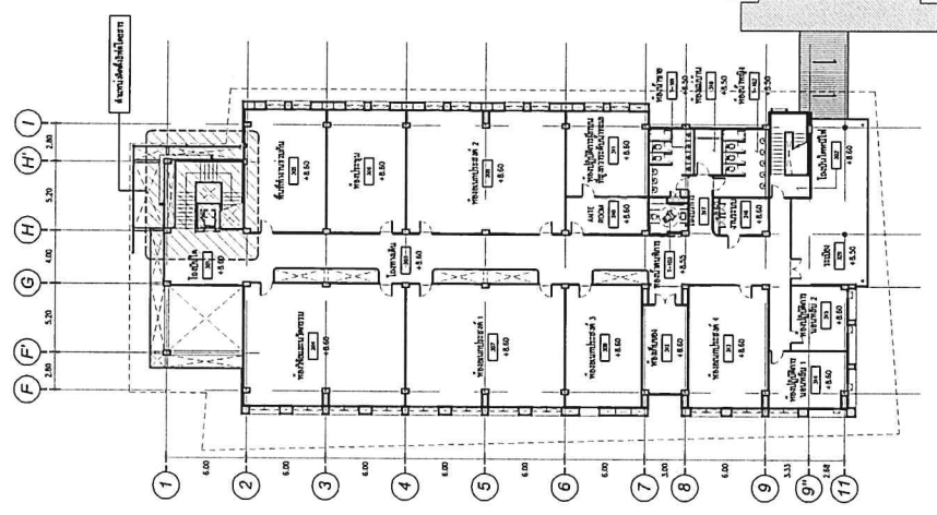
ชั้นที่ 1 SCALE 1:200
