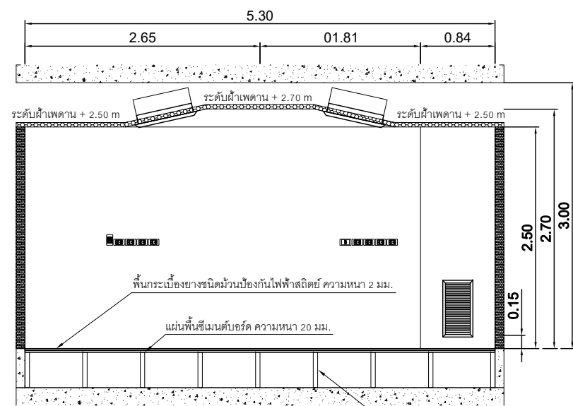
รูปตัด D
