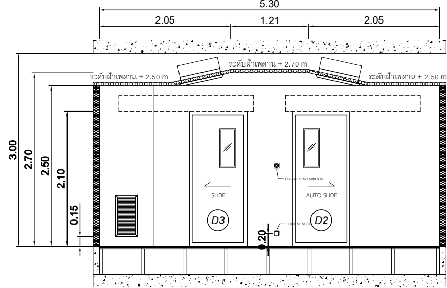
รูปตัด B
