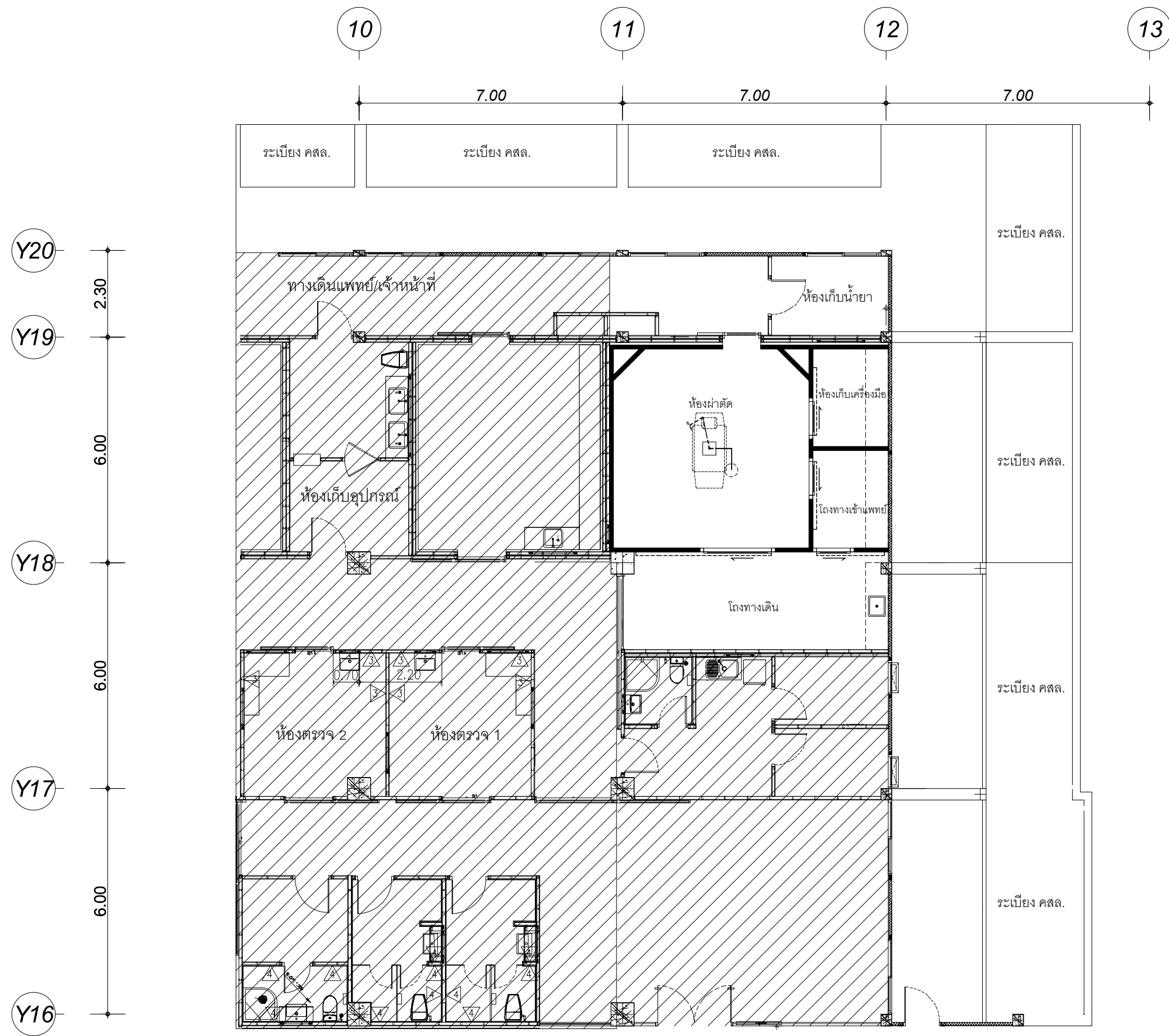
แบบแปลนปรับปรุงห้องผ่าตัด
