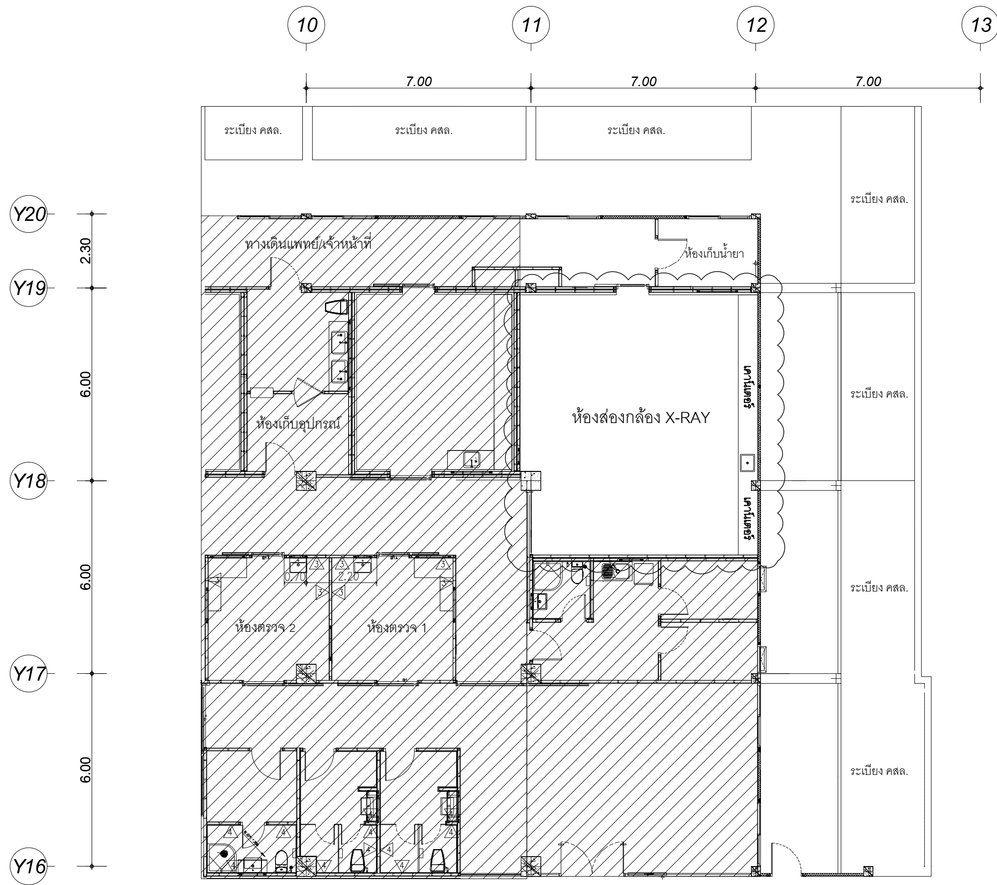
แบบแปลนเดิม ชั้น 2 อาคาร 80 ปี
