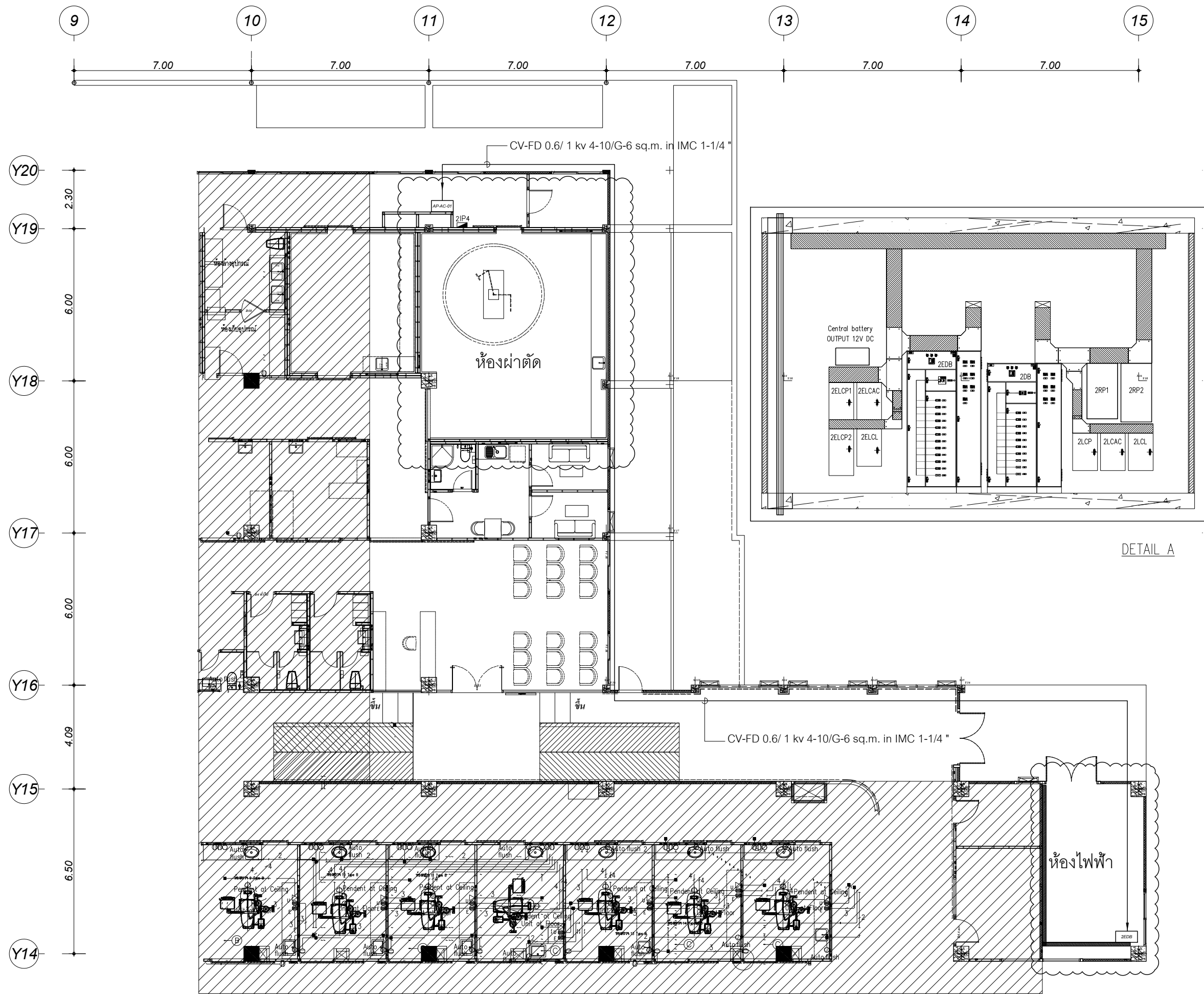
แบบเมนไฟฟ้าระบบปรับอากาศห้องผ่าตัด
