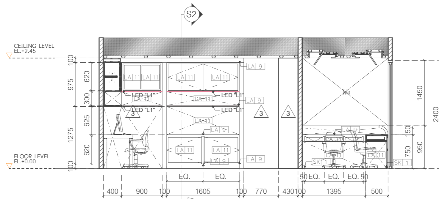
1 ELEVATION-E3 SCALE 1 : 50
