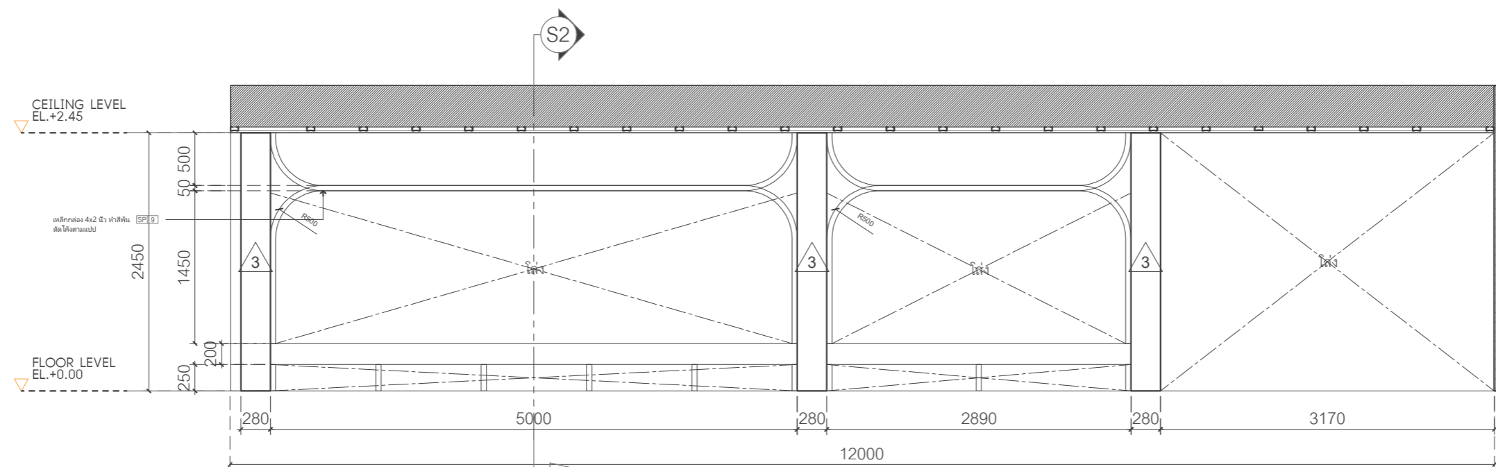
2 ELEVATION-E3 SCALE 1 : 50
