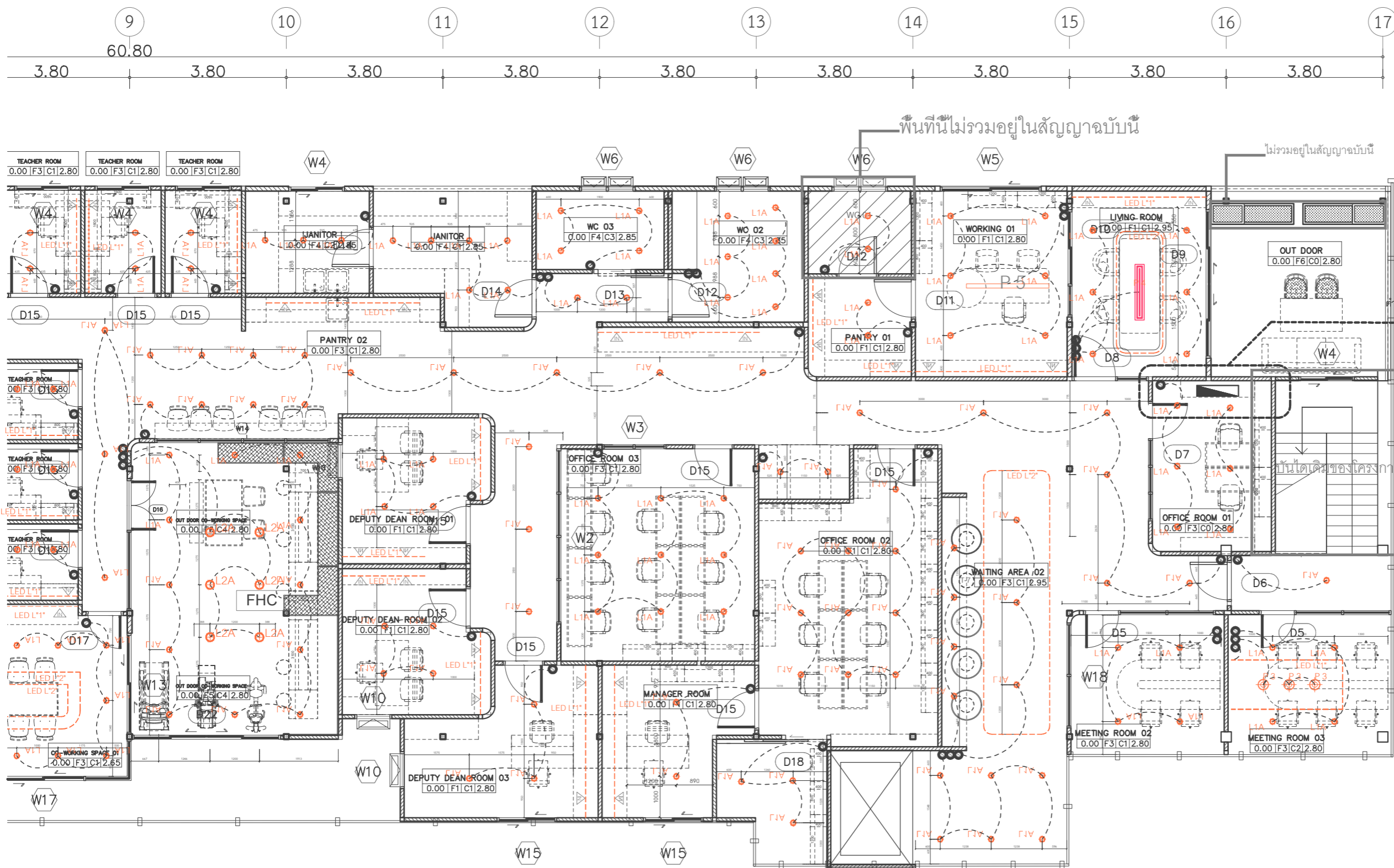
มหาวิทยาลัยศรีนครินทรวิโรฒ CCI LIGHTING PLAN FLOOR 4-2 SCALE 1:100
