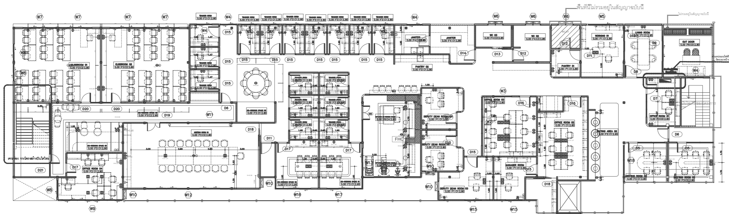
มหาวิทยาลัยศรีนครินทรวิโรฒ CCI ELECTRICAL OUTLET PLAN FLOOR 4 SCALE 1 : 200
