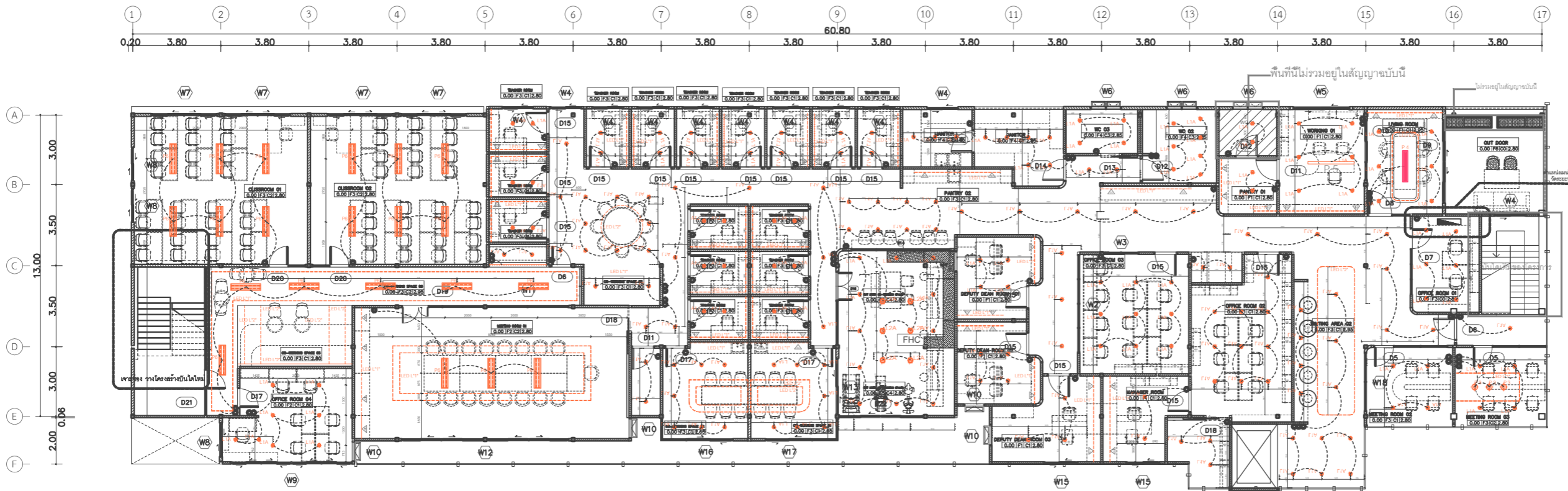
มหาวิทยาลัยศรีนครินทรวิโรฒ CCI LIGHTING PLAN FLOOR 4 SCALE 1 : 200
