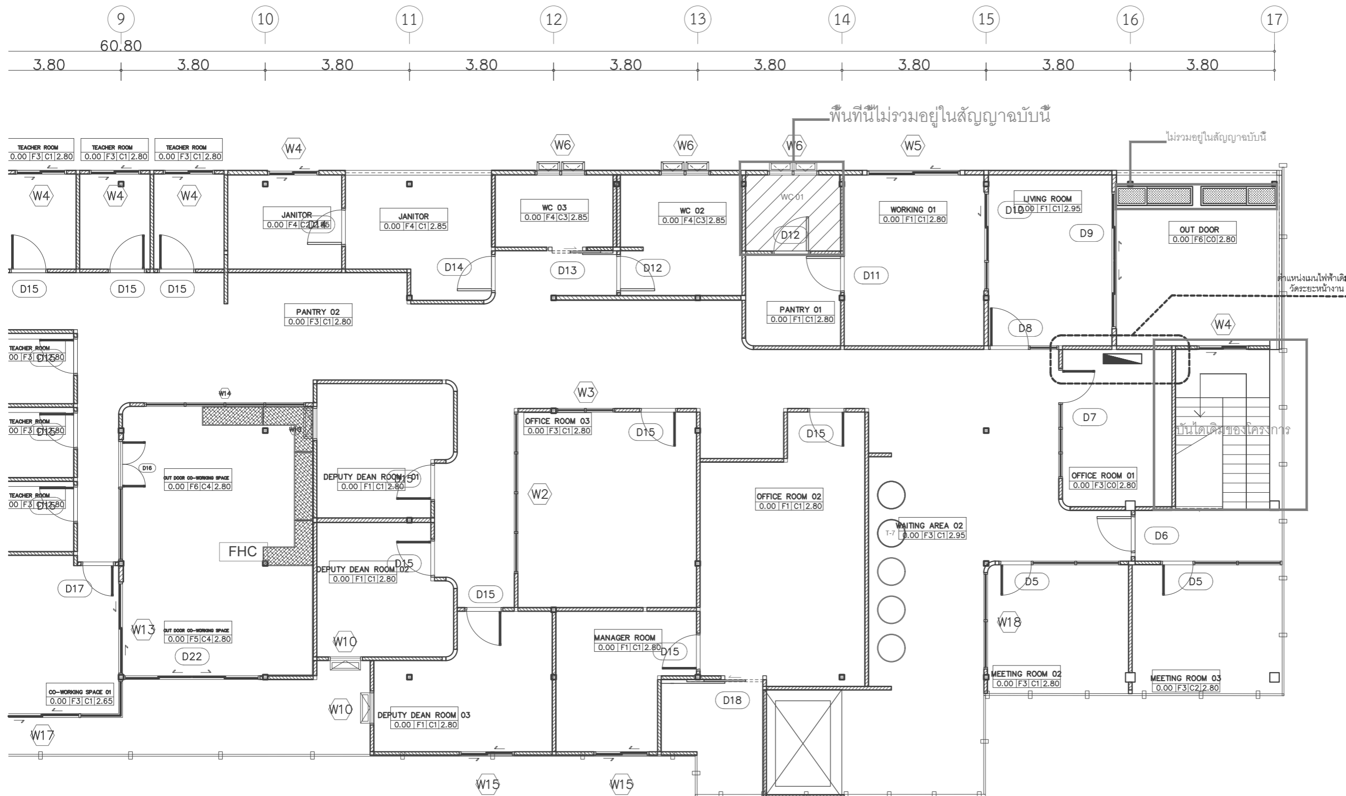
มหาวิทยาลัยศรีนครินทรวิโรฒ CCI ELECTRICAL OUTLET PLAN FLOOR 4-2 SCALE 1:100
