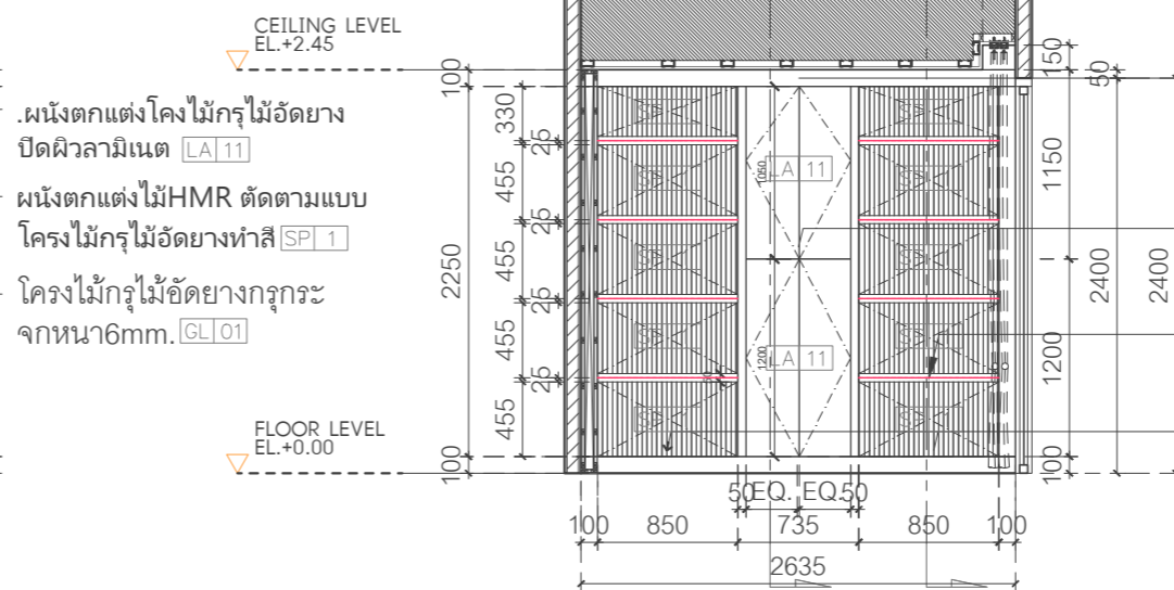
4 ELEVATION-E3 SCALE 1 : 50
