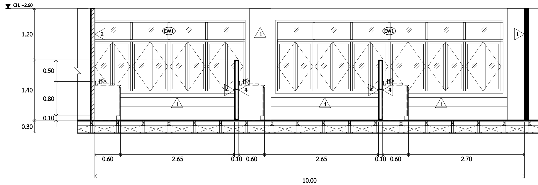
รูปตัด A AA7.02 SCALE 1 : 50
