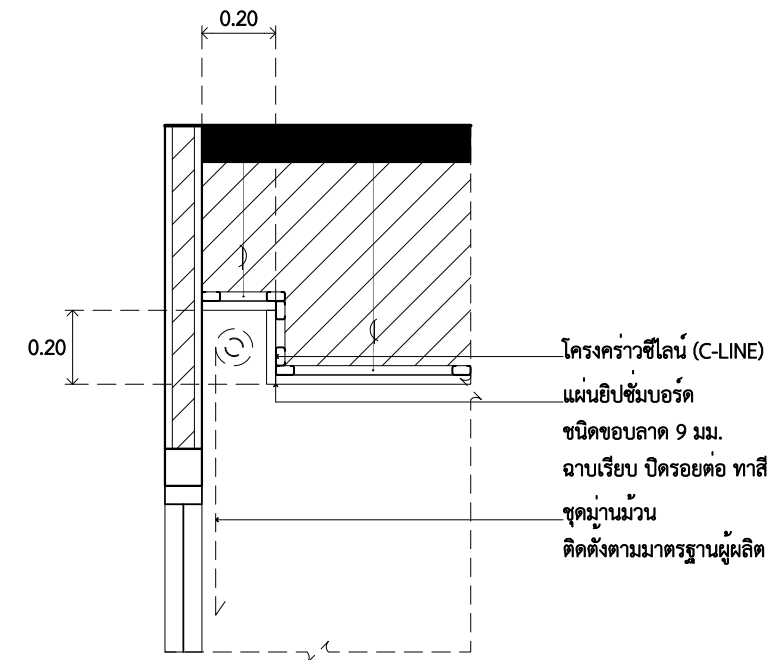
2 แบบขยายฝ้าเพดาน AA9.03 SCALE 1 : 200
