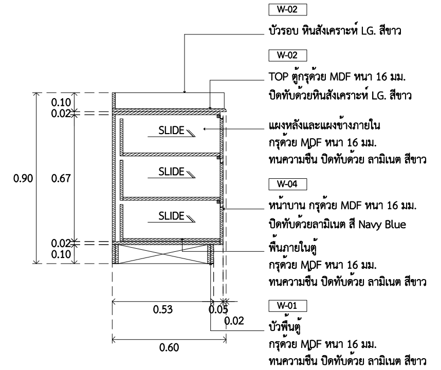
A รูปตัด A AA8.01 SCALE 1 : 50
