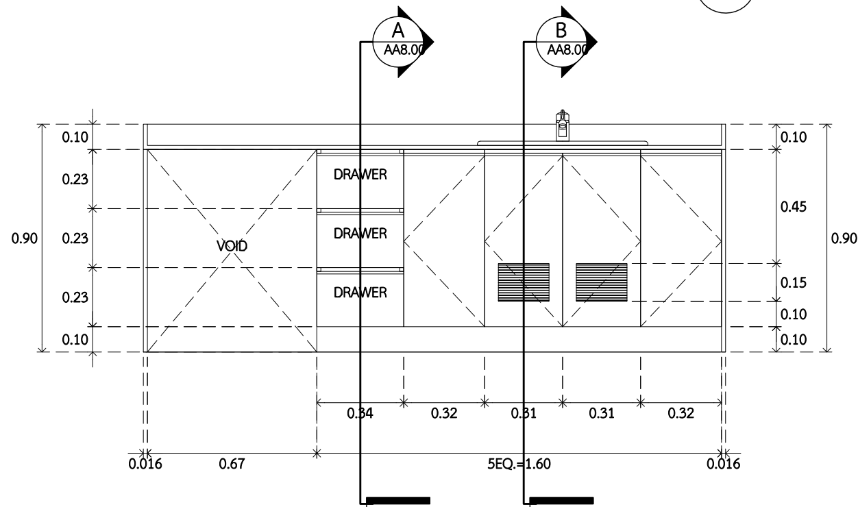
1 รูปด้าน 1 AA8.00 SCALE 1 : 20
