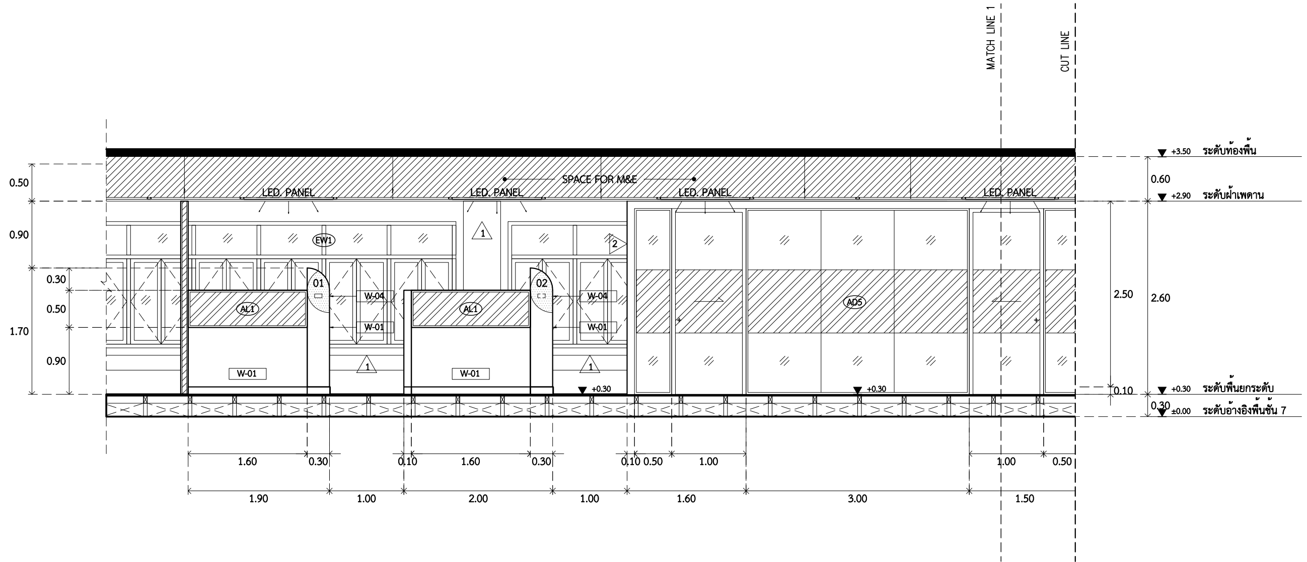
รูปด้าน 1 (ส่วนที่ 1) AA4.01 SCALE 1 : 50
