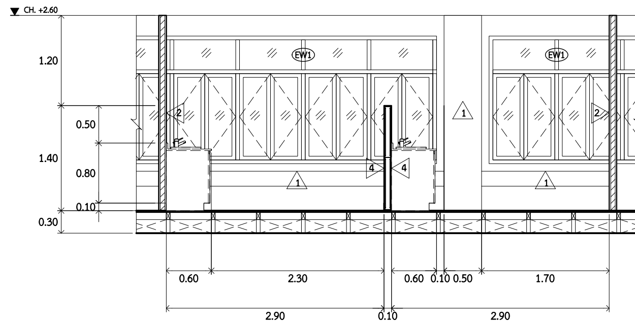
รูปตัด B SCALE 1 : 50
