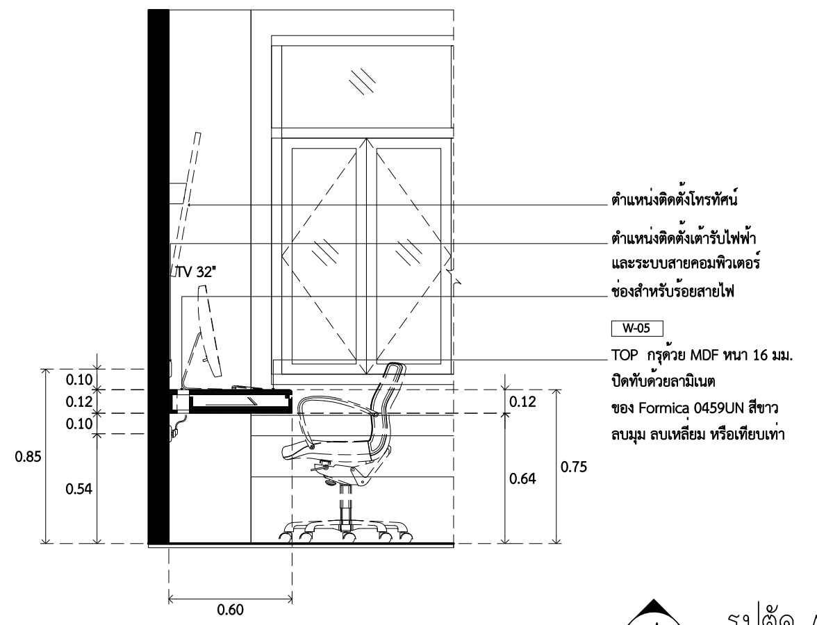
1 แบบขยายเฟอร์นิเจอร์ B7 AA8.06 SCALE 1 : 25
