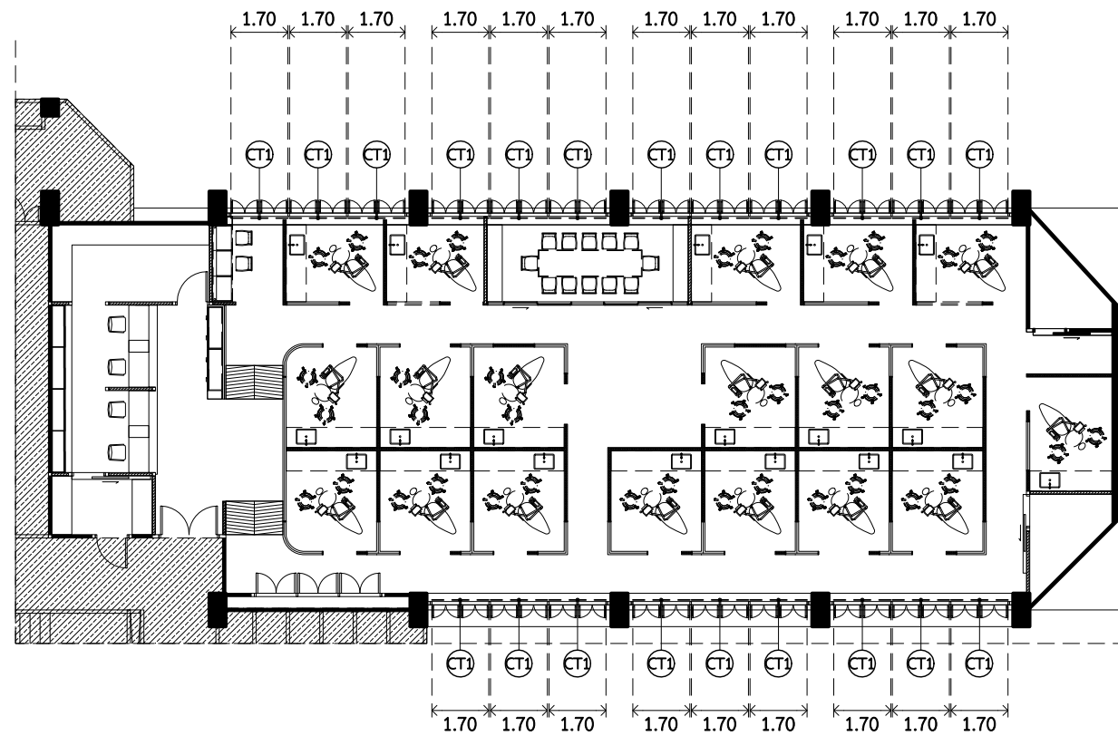
1 ผังรายละเอียดชุดม่านบังแสง AA9.03 SCALE 1 : 200
