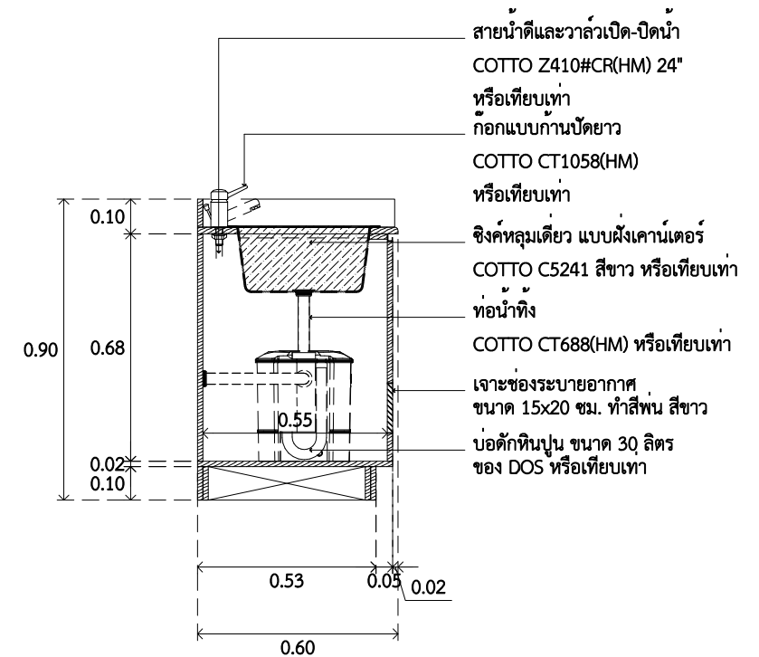
B รูปตัด B AA8.00 SCALE 1 : 20
