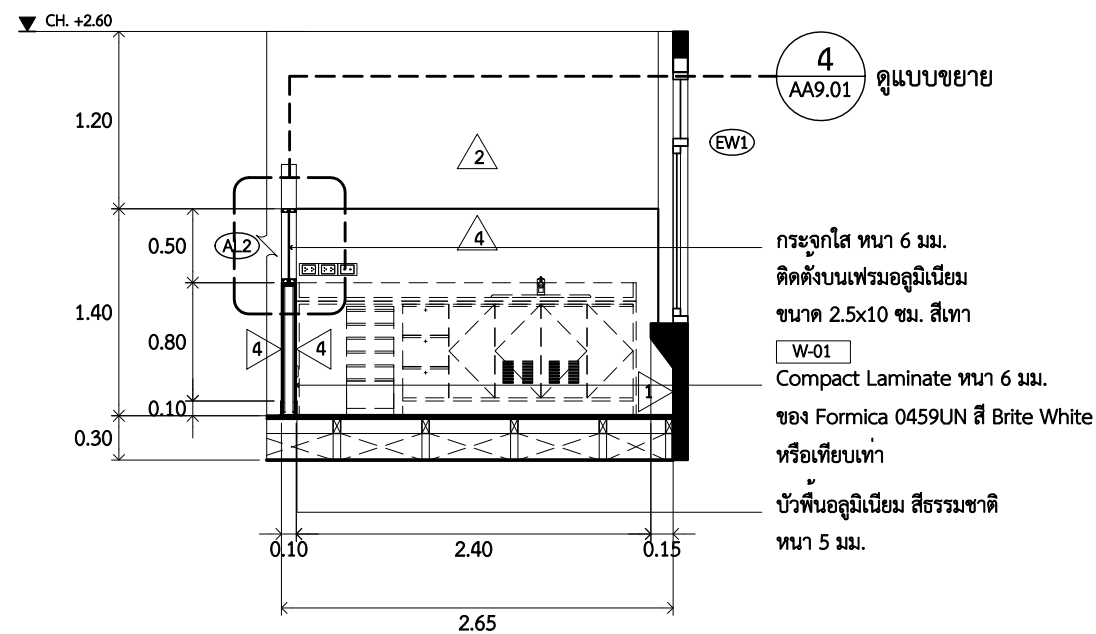
รูปตัด B AA7.02 SCALE 1 : 50
