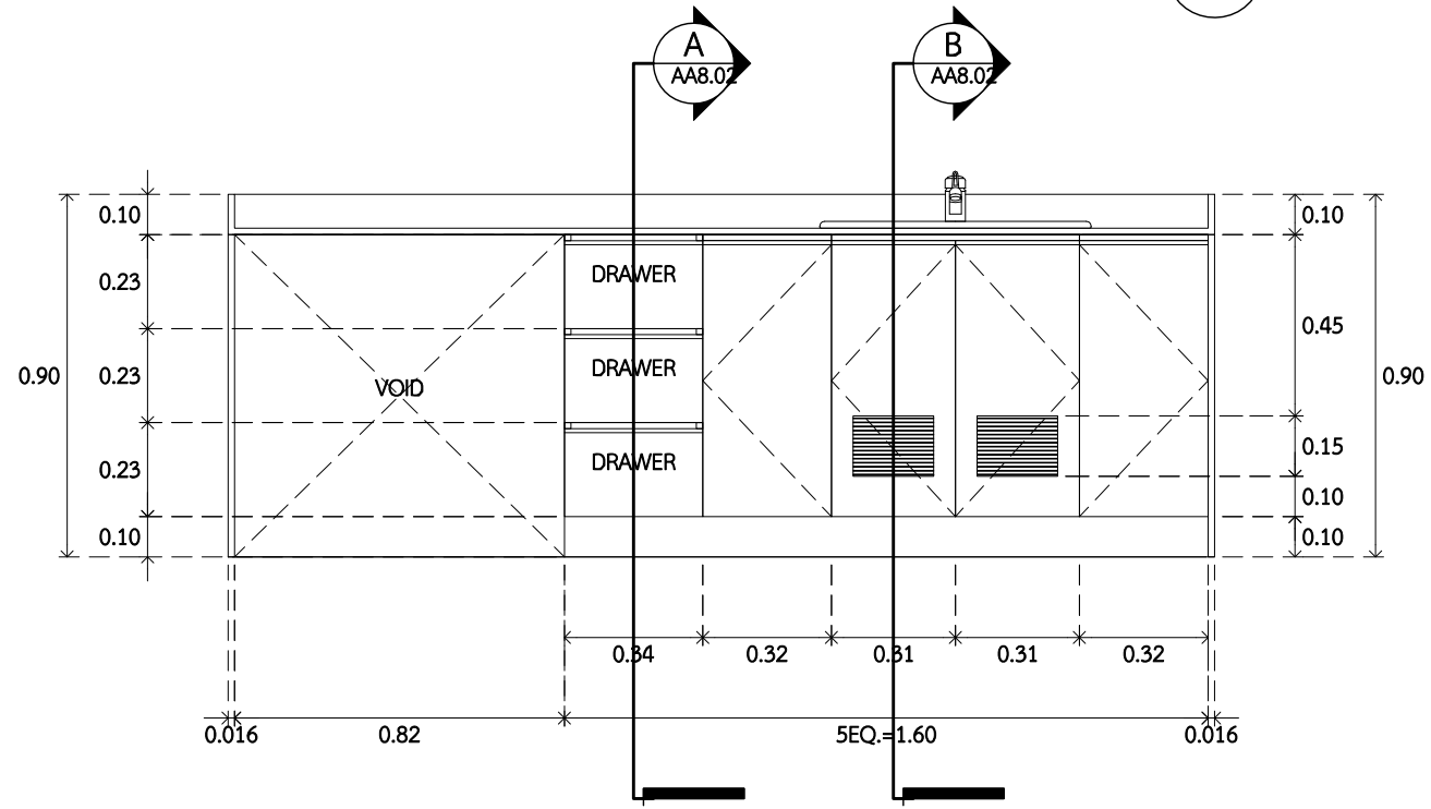
1 รูปด้าน 1 AA8.02 SCALE 1 : 20
