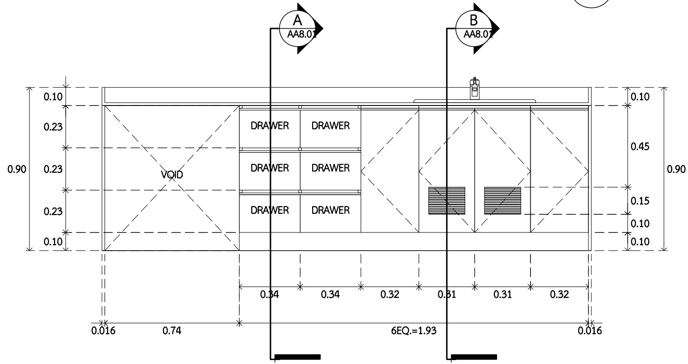
1 รูปด้าน 1 AA8.01 SCALE 1 : 20
