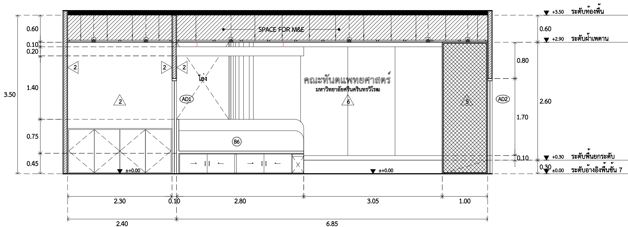
รูปด้าน 6 SCALE 1 : 50
