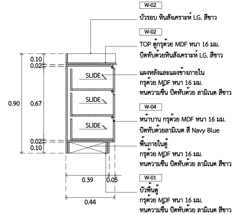
รูปตัด A A3.03 SCALE 1 : 50
