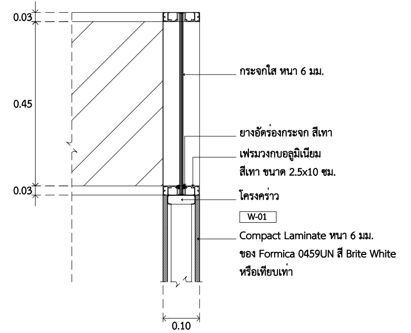
4 แบบขยายผนัง 4 AA9.01 SCALE 1 : 10
