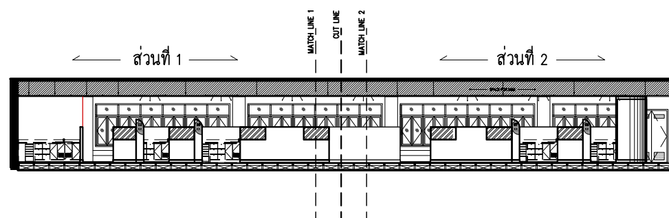
รูปด้าน 4 SCALE 1 : 200
