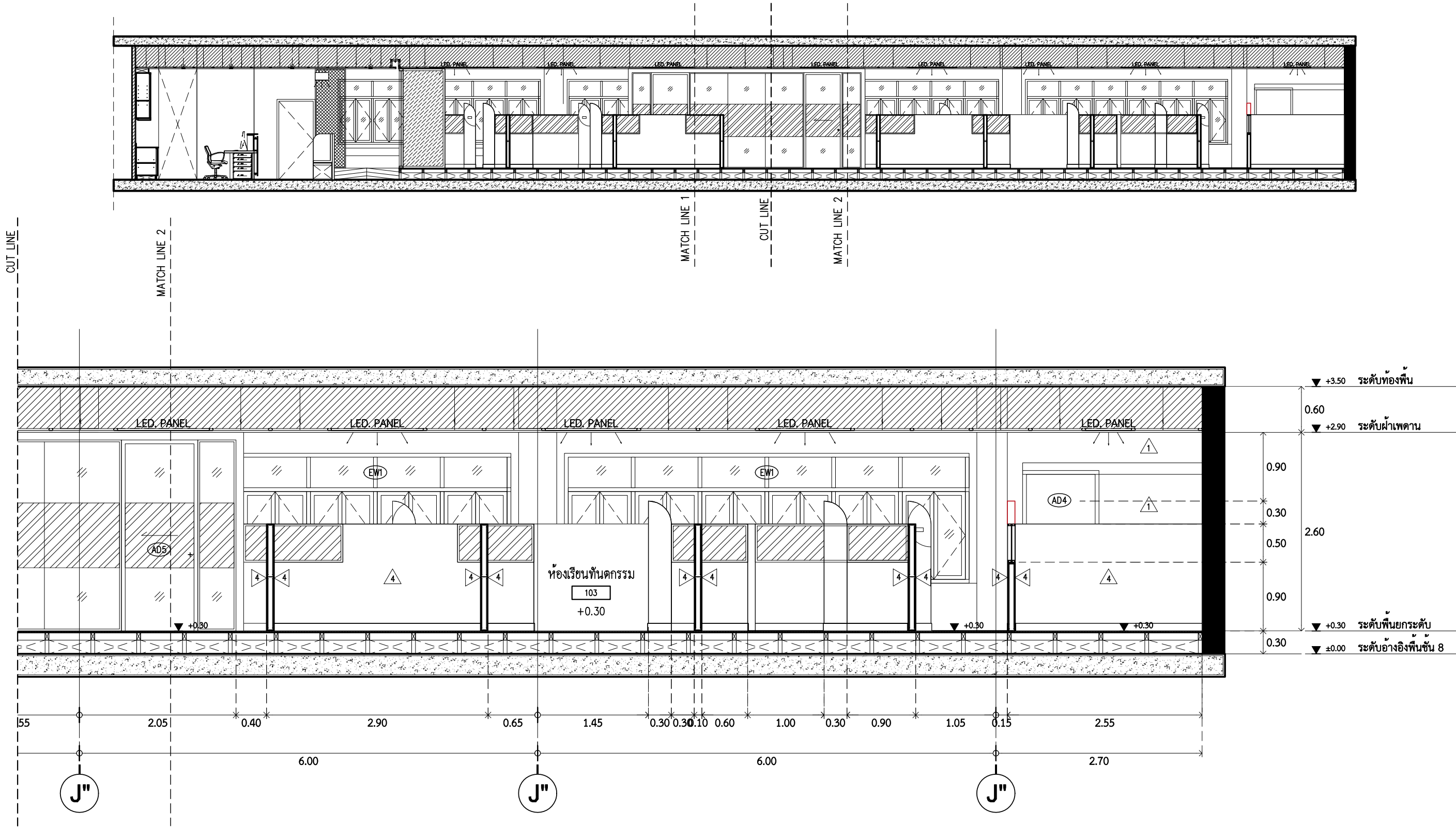
B AA3.02 รูปตัด B (ส่วนที่ 2) SCALE 1 : 50
