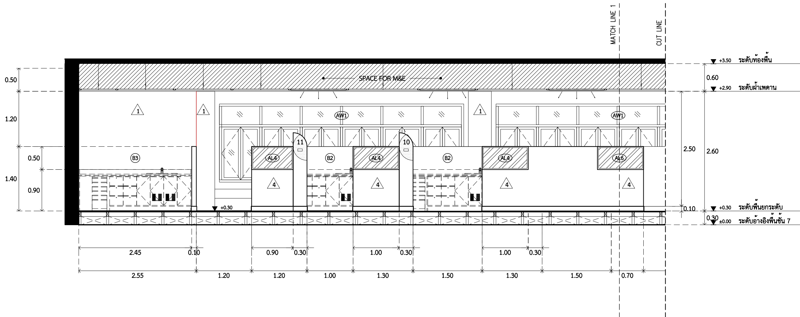
รูปด้าน 4 (ส่วนที่ 1) SCALE 1 : 50
