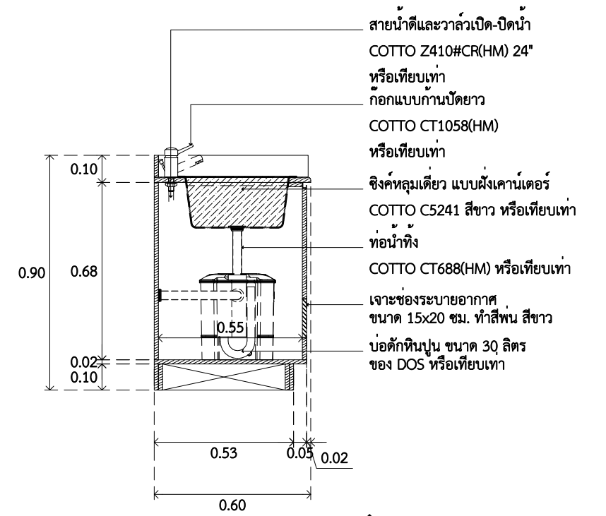
B รูปตัด B AA8.02 SCALE 1 : 50
