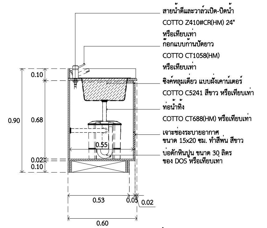
B รูปตัด B AA8.01 SCALE 1 : 50
