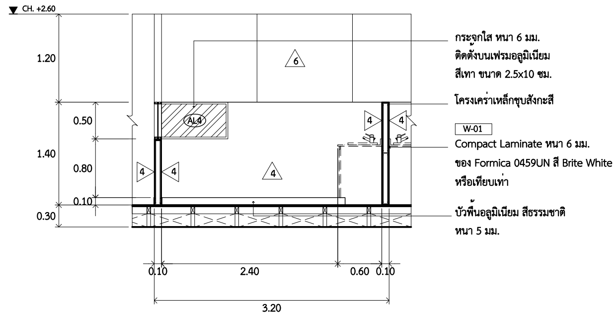
รูปตัด B AA7.04 SCALE 1 : 50
