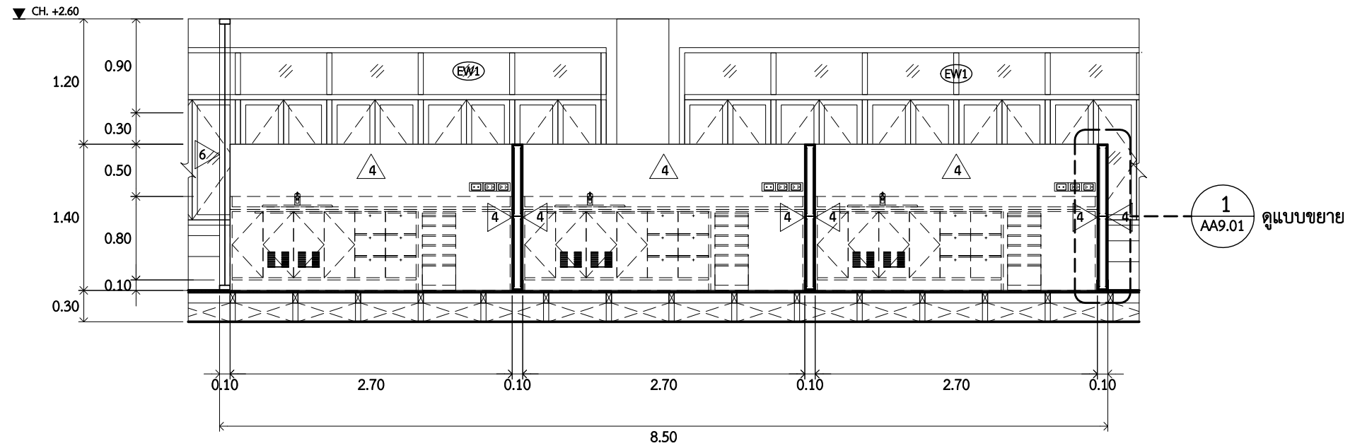
รูปตัด A AA7.04 SCALE 1 : 50
