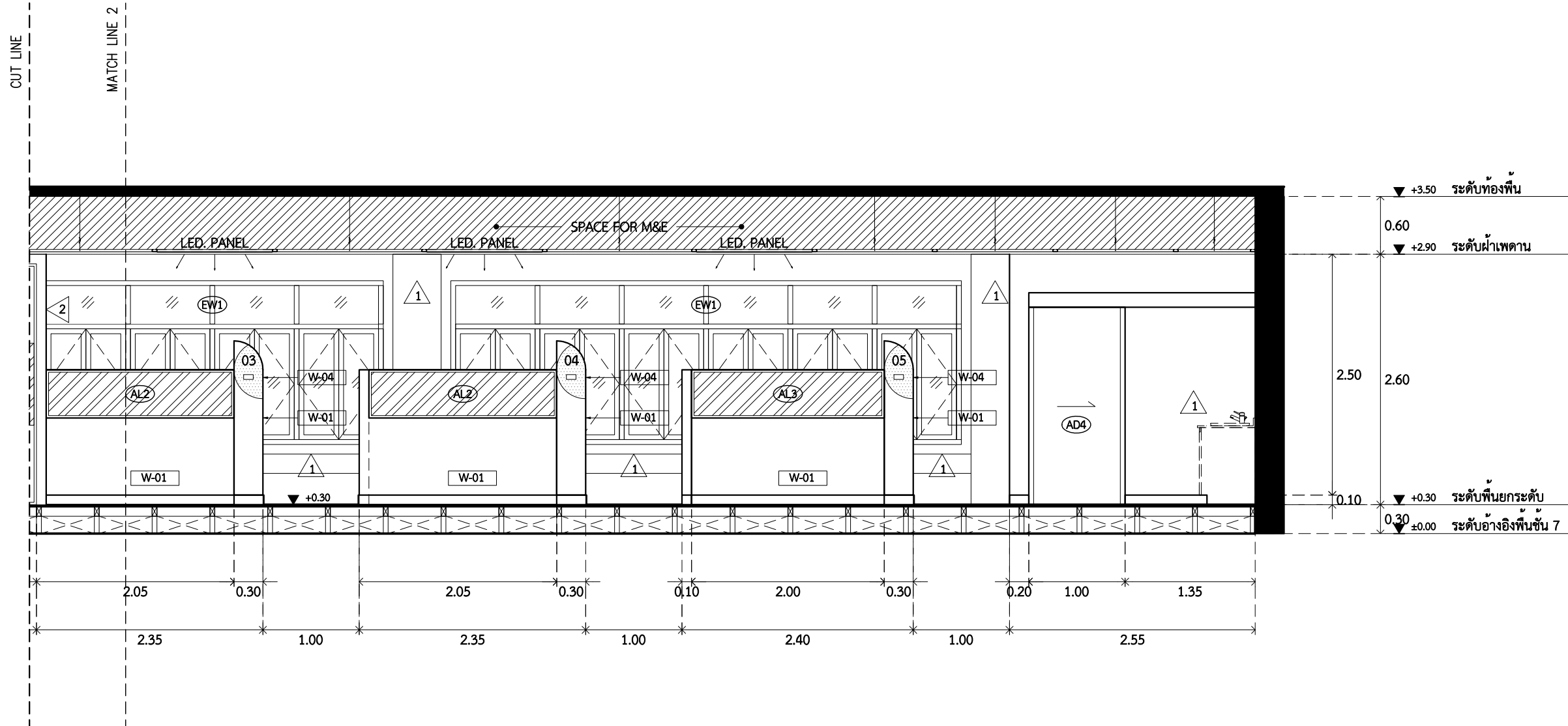
รูปด้าน 1 (ส่วนที่ 2) SCALE 1 : 50
