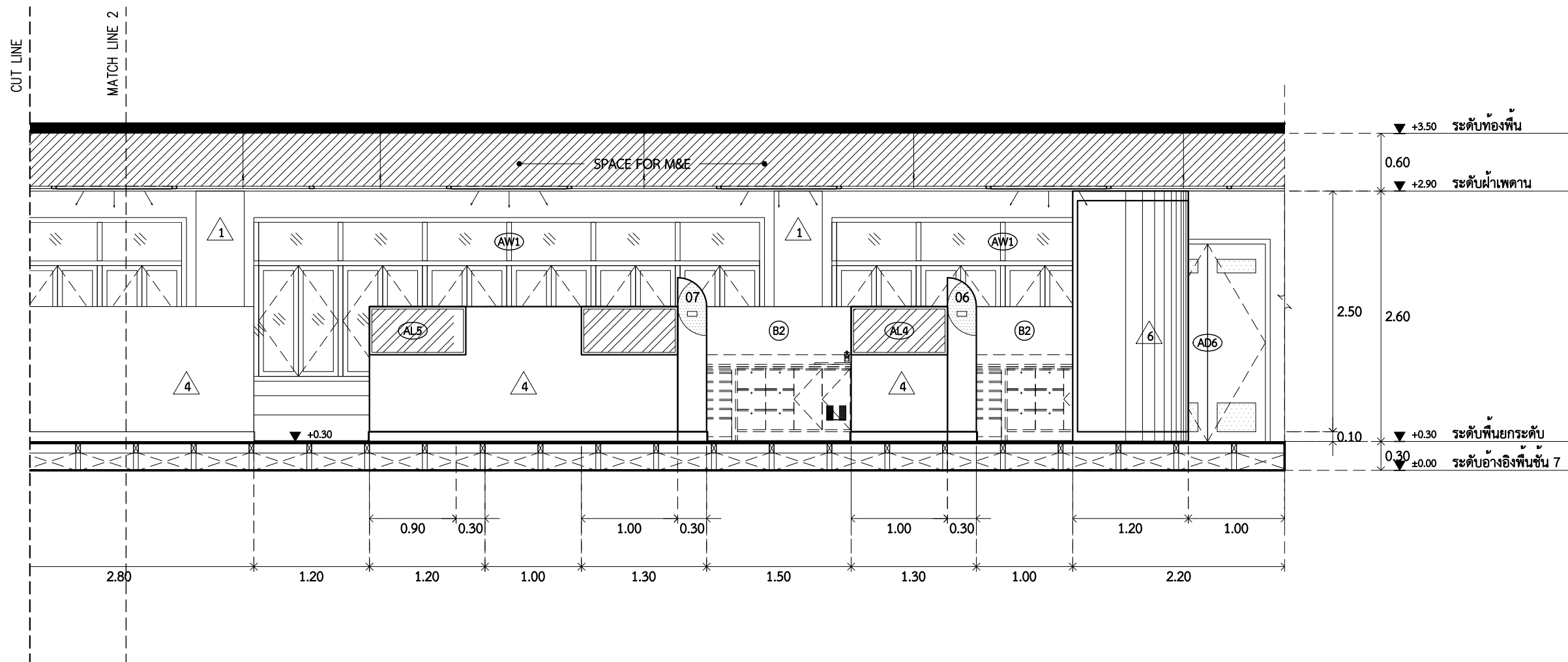
รูปด้าน 4 (ส่วนที่ 2) SCALE 1 : 50
