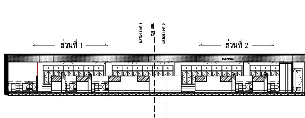
รูปด้าน 4 SCALE 1 : 200
