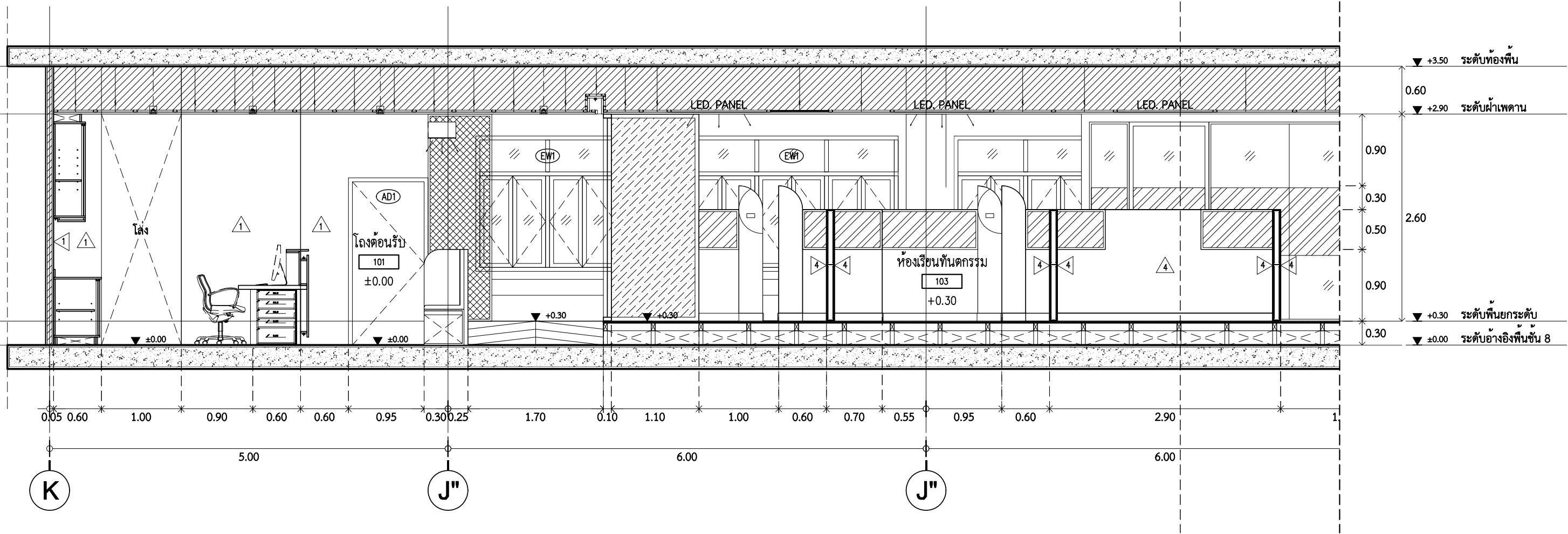
รูปตัด B (ส่วนที่ 1) AA3.01 SCALE 1 : 50
