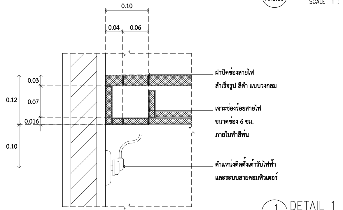
1 รูปด้าน 1 A2.00 SCALE 1 : 25
