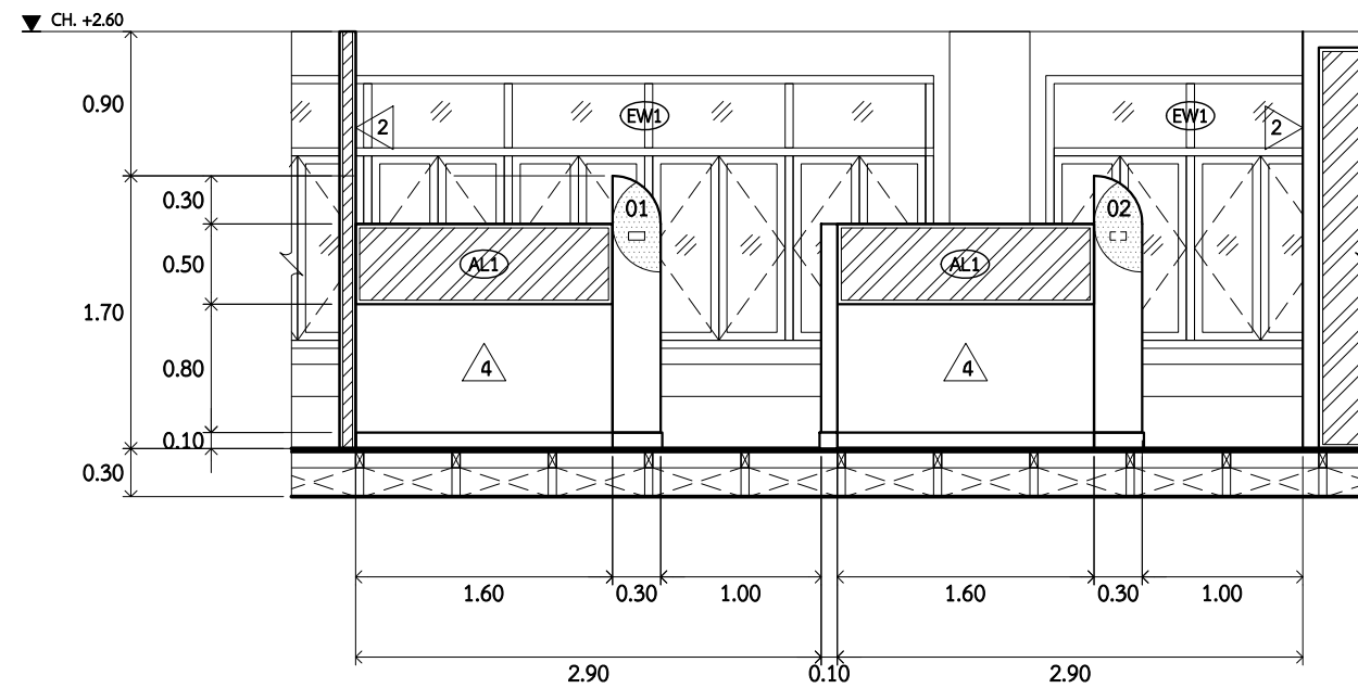
รูปตัด 1 SCALE 1 : 50
