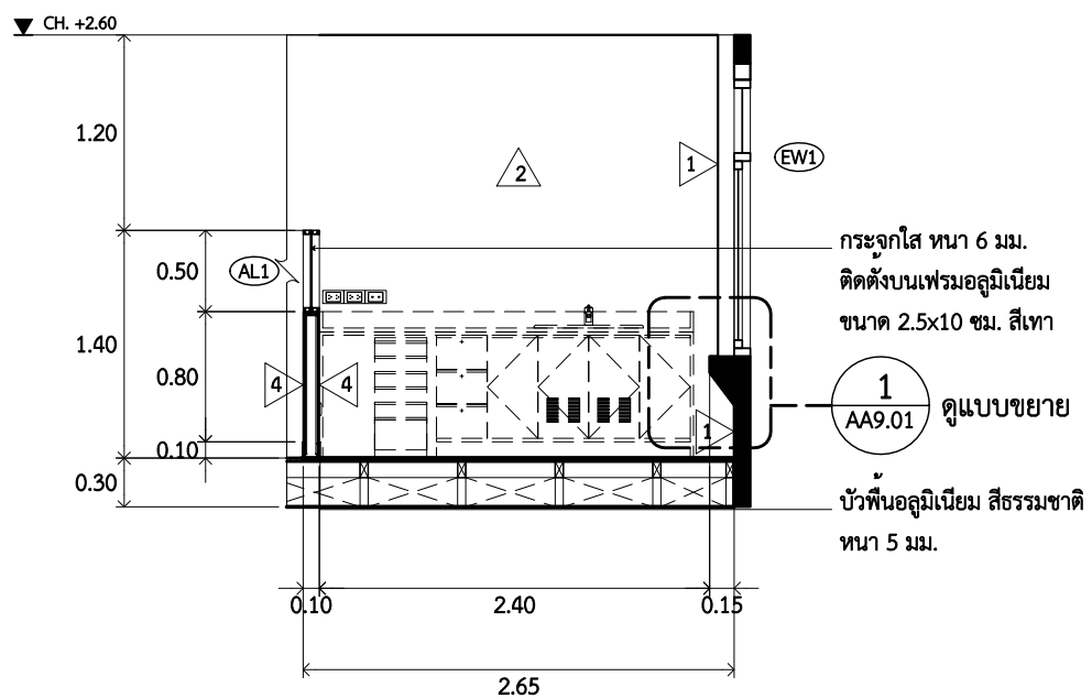
1 AA7.00 ผังยูนิตทันตกรรมแบบที่ 1 SCALE 1 : 50
