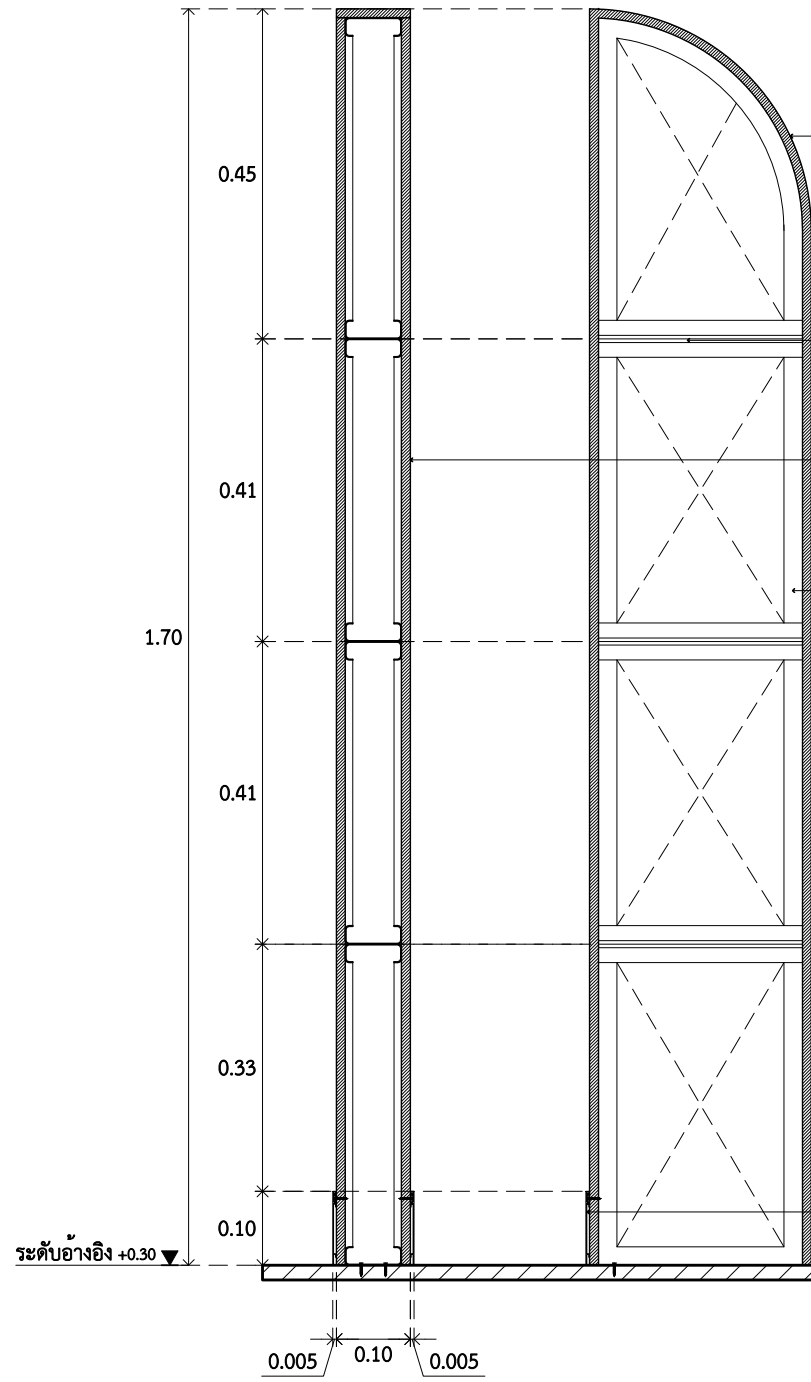
1 รูปด้าน 1 AA9.00 SCALE 1 : 10
