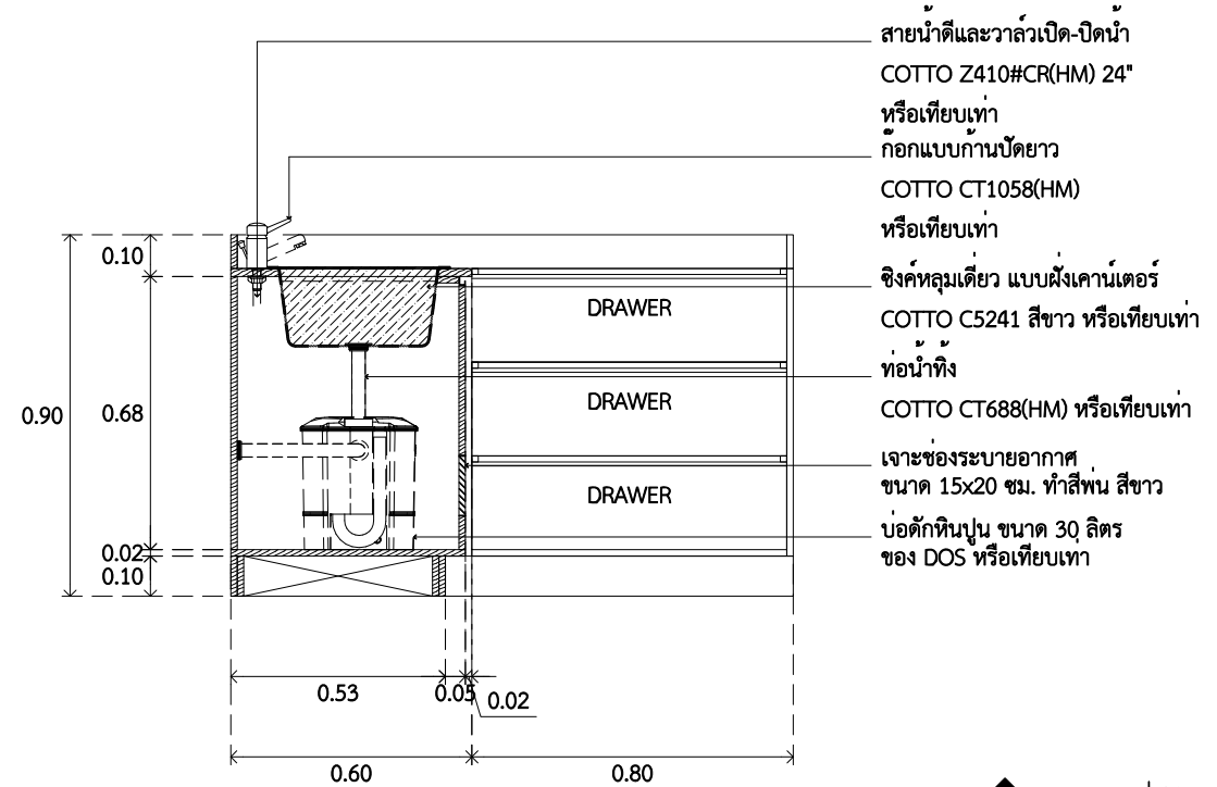
รูปตัด B AA8.03 SCALE 1 : 50
