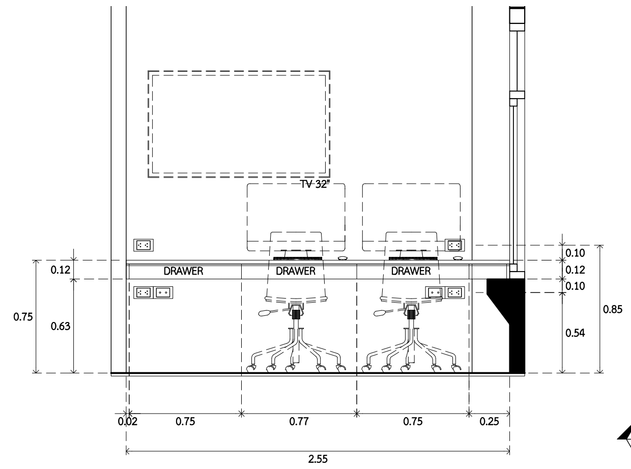
1 แบบขยายเฟอร์นิเจอร์ B7 AA8.06 SCALE 1 : 25
