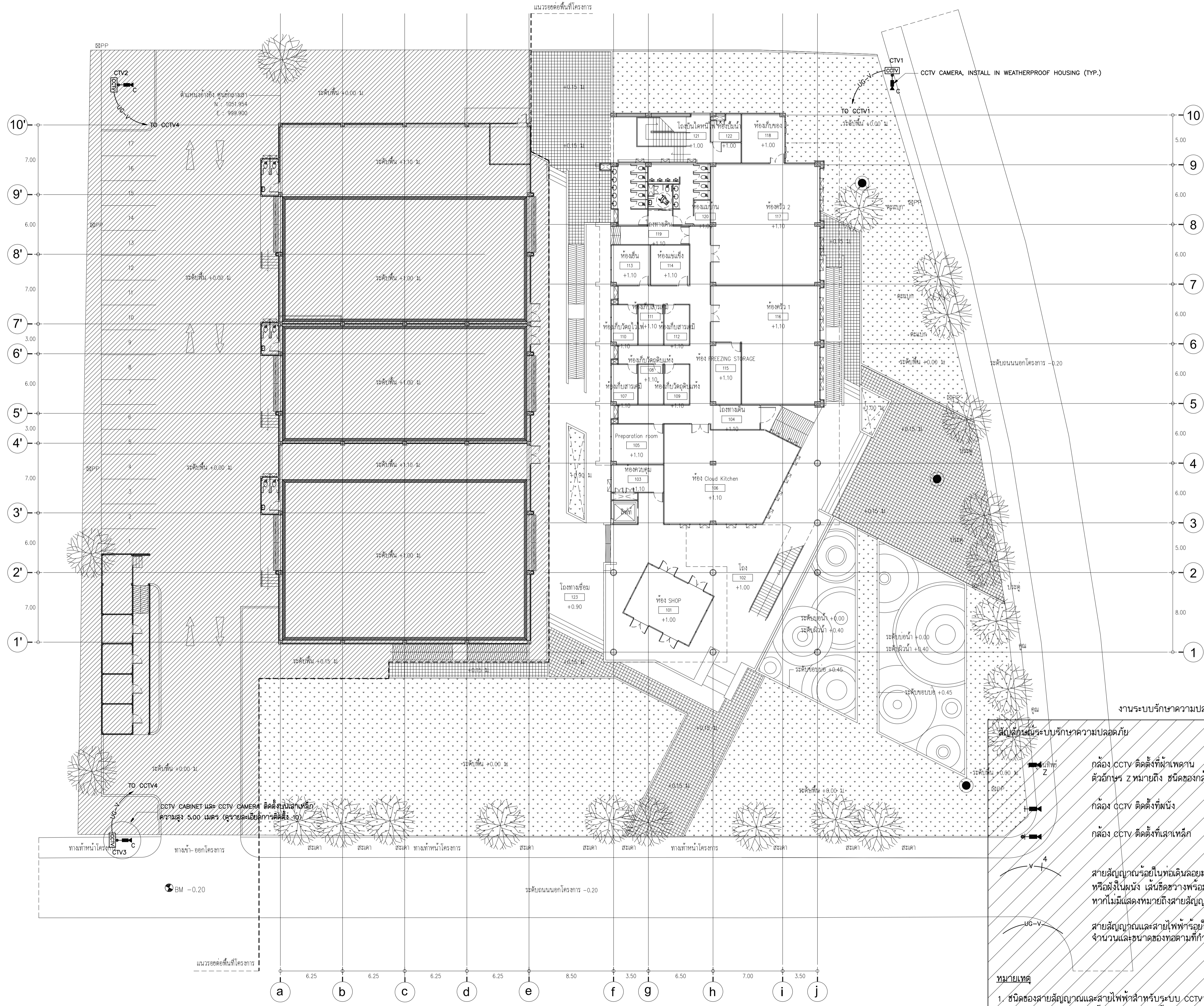
ผังระบบรักษาความปลอดภัยภายนอกอาคาร SCALE 1 : 200
