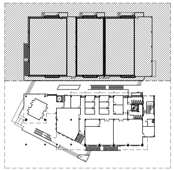
ผังพื้นที่อาคารปฏิบัติการ
