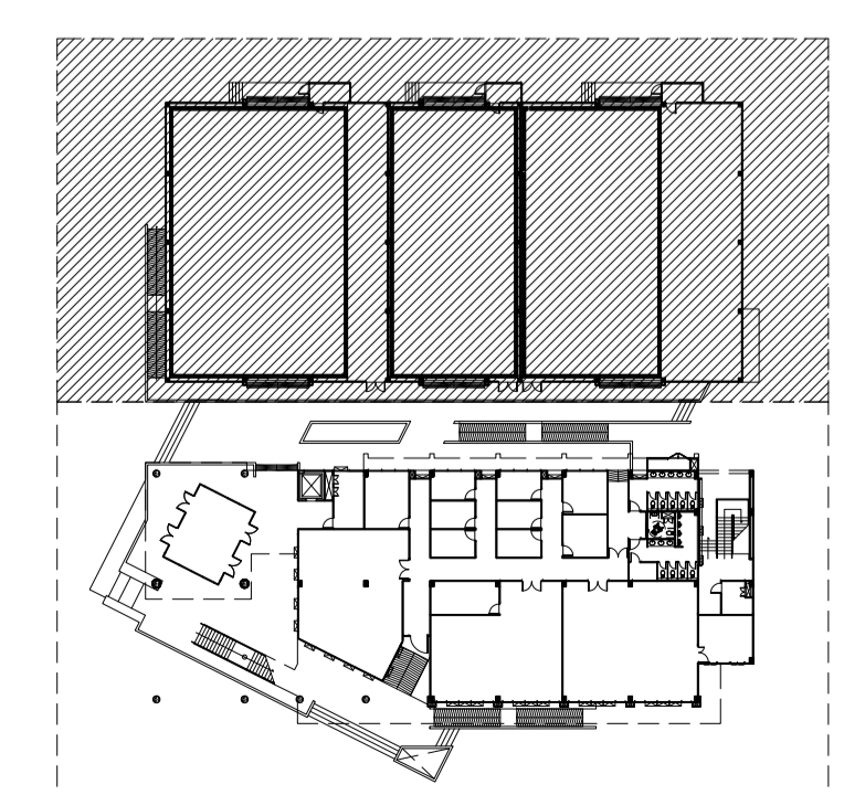
ผังพื้นที่อาคารปฏิบัติการ
