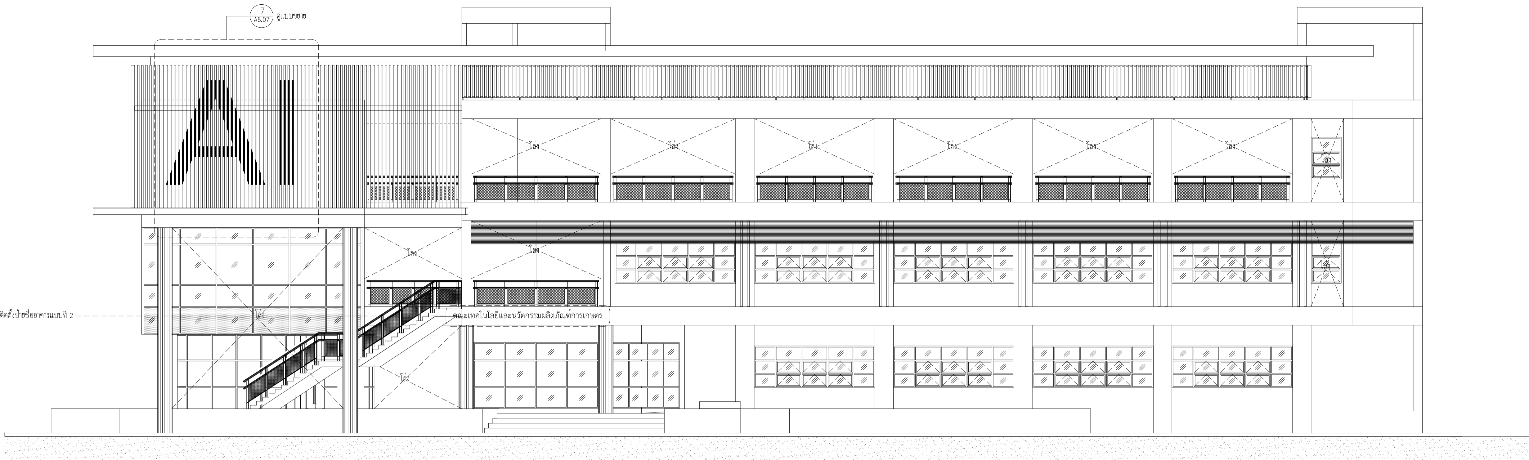
รูปด้าน 1 (แสดงตำแหน่งการติดตั้งป้าย) SCALE 1 : 100
