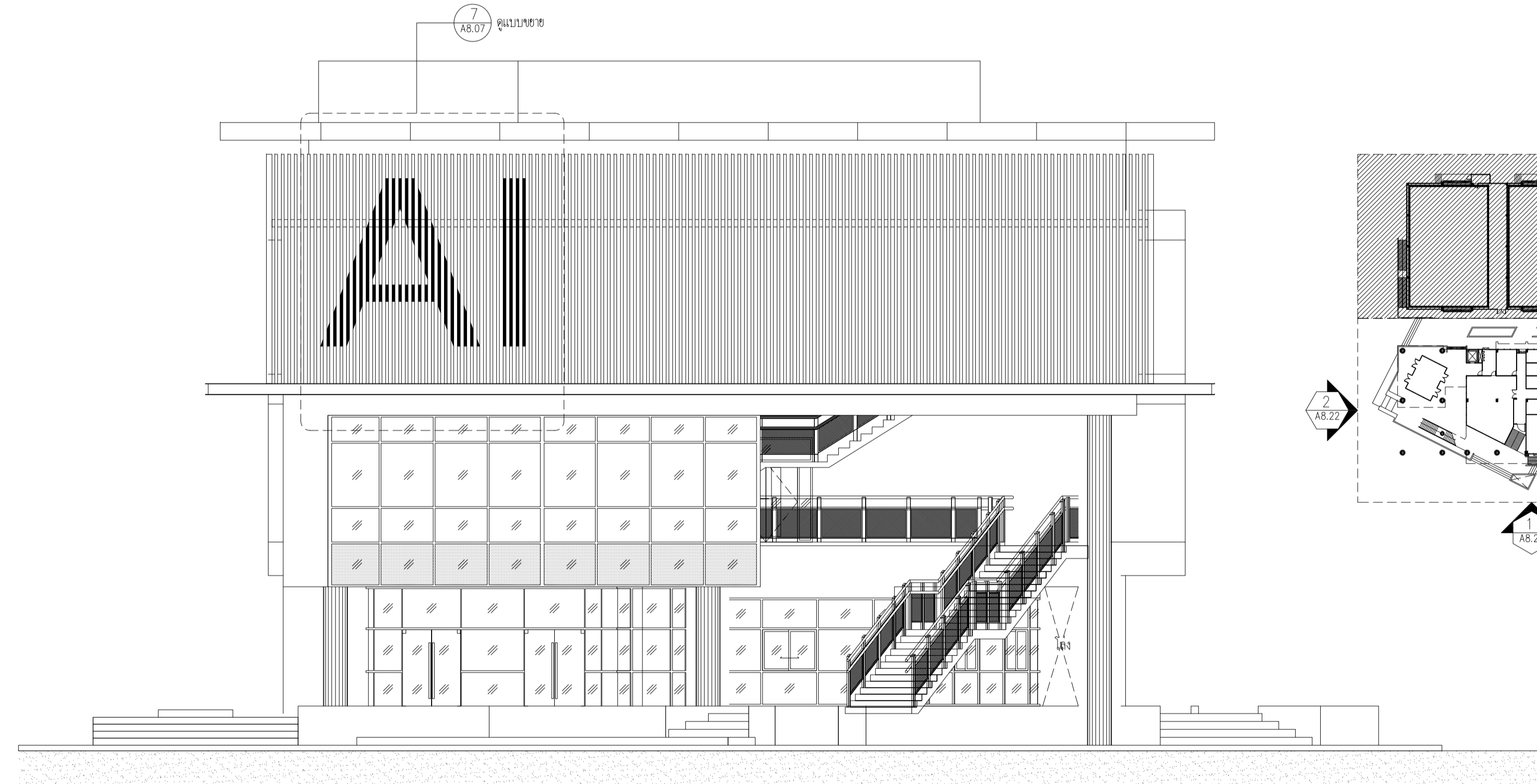
รูปด้าน 1 (แสดงตำแหน่งการติดตั้งป้าย) SCALE 1 : 100
