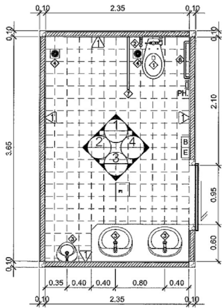
แปลนขยายห้องน้ำคนพิการ
