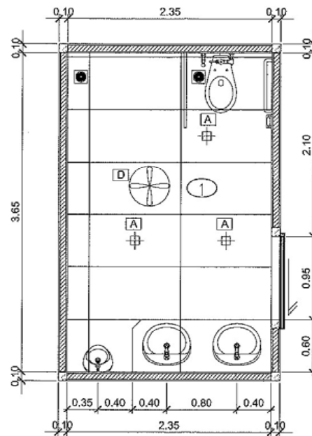
แปลนไฟฟ้าเพดานห้องน้ำคนพิการ
