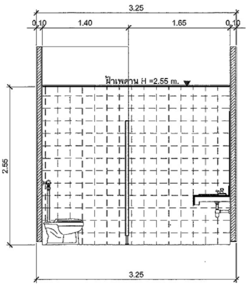
รูปตัดขยาย - 3 มาตรฐาน 1:50
