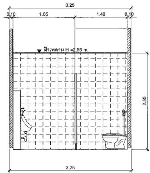
รูปตัดขยาย - 1 มาตรฐาน 1:50
