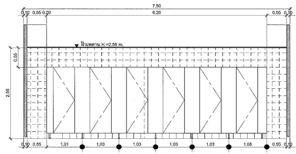
รูปตัดขยาย - 2 มาตรฐาน 1:50
