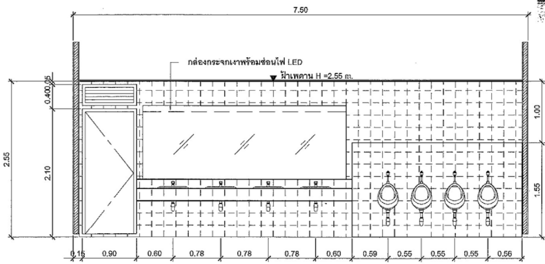
รูปตัดขยาย - 4 มาตรฐาน 1:50
