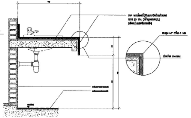
รูปตัดขยายเคาน์เตอร์
