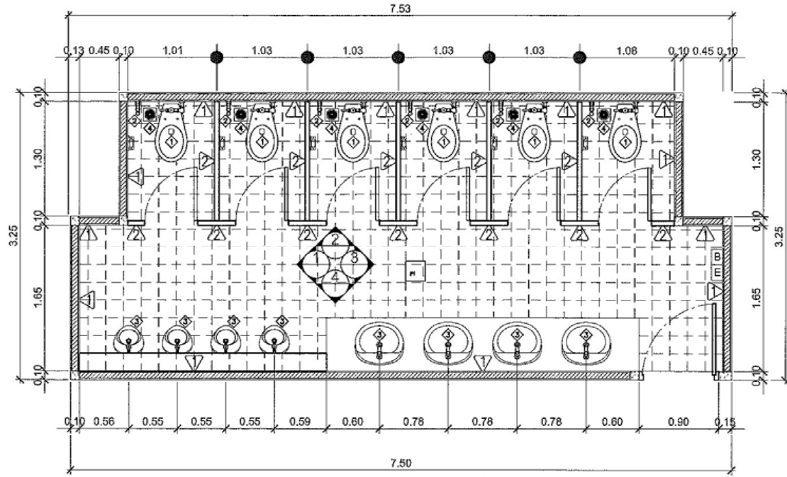
แปลนขยายห้องน้ำ 106
