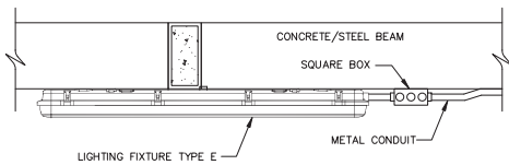
รายละเอียดการติดตั้ง 3 การติดตั้งโคมไฟกั้นน้ำชนิดติดตั้งที่ผนัง NOT TO SCALE
