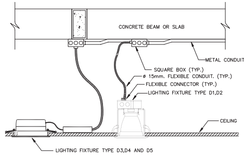
รายละเอียดการติดตั้ง 2 การติดตั้งโคมไฟ DOWNLIGHT ชนิดฝังฝ้าเพดาน NOT TO SCALE
