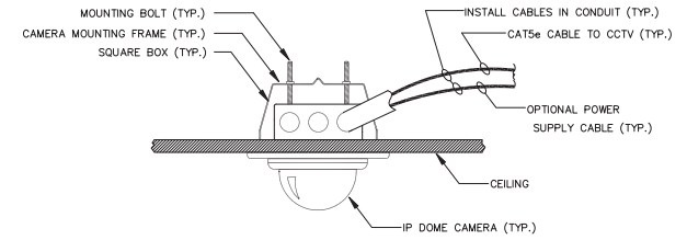
รายละเอียดการติดตั้ง 6 การติดตั้ง INDOOR IP DOME CAMERA แบบฝังฝ้าเพดาน NOT TO SCALE
