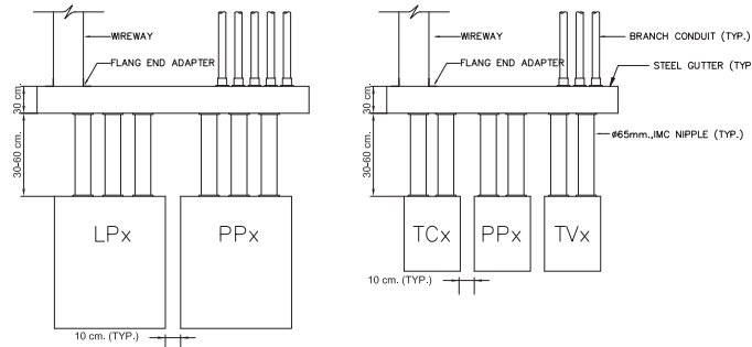
รายละเอียดการติดตั้ง 8 TYPICAL ARRANGEMENT INSTALLATION OF ELECTRICAL PANELBOARD AND COMMUNICATION PANEL NOT TO SCALE
