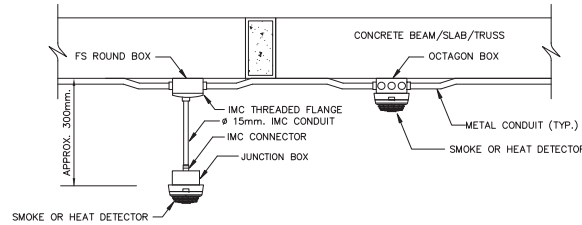
รายละเอียดการติดตั้ง 4 การติดตั้ง FIRE ALARM DETECTOR แบบติดตั้งใต้ฝ้าเพดาน NOT TO SCALE
