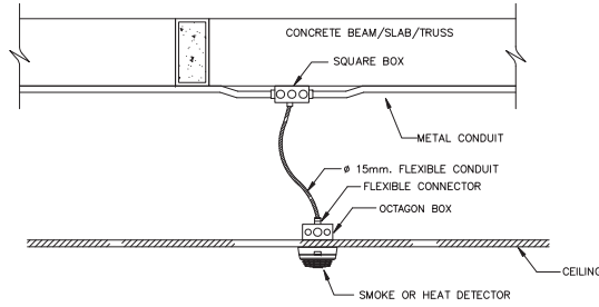
รายละเอียดการติดตั้ง 4 การติดตั้ง FIRE ALARM DETECTOR แบบติดตั้งใต้ฝ้าเพดาน NOT TO SCALE
