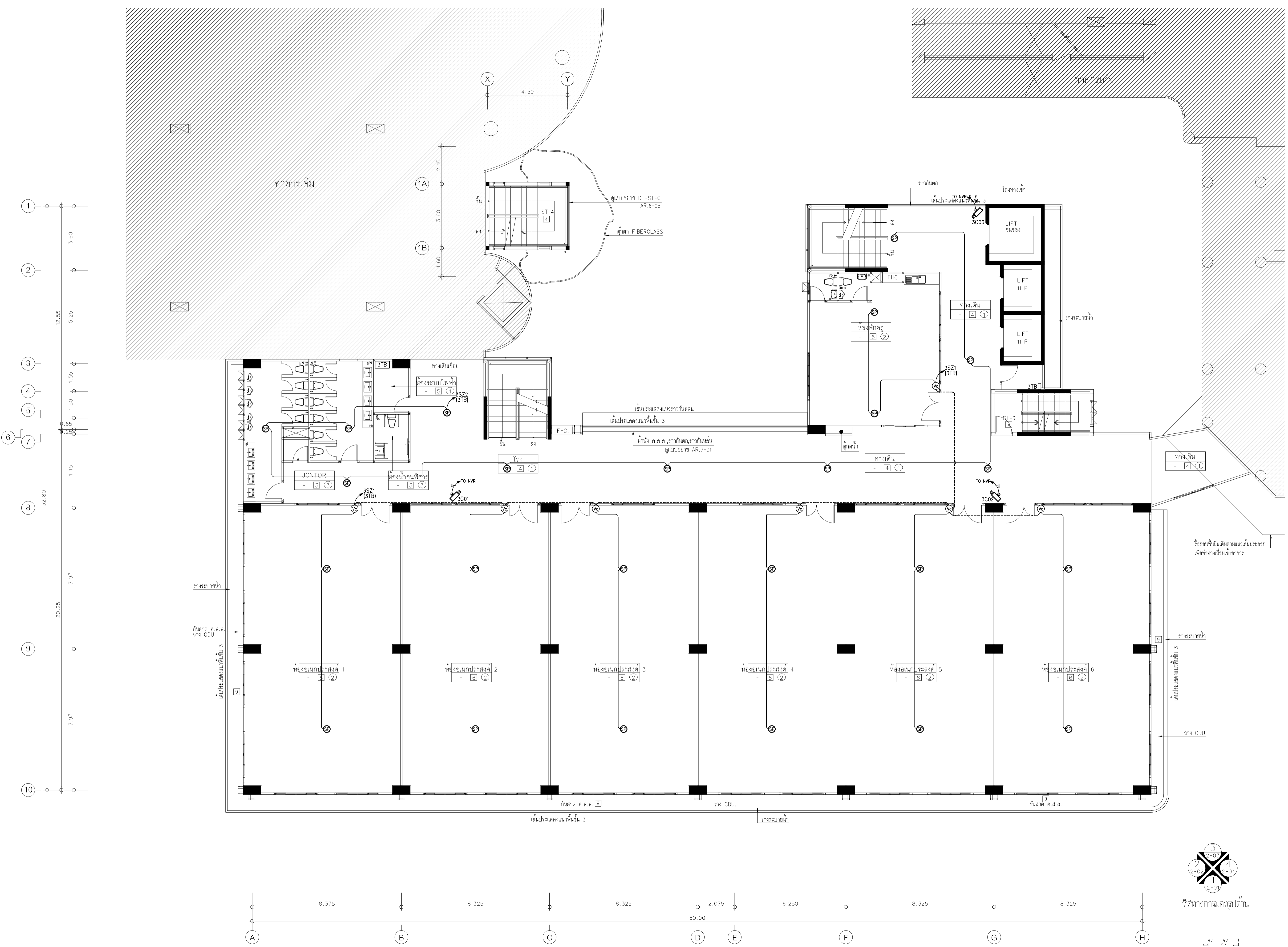
ผังระบบเสียงและระบบรักษาความปลอดภัย ชั้น 3 มาตราส่วน 1:100
