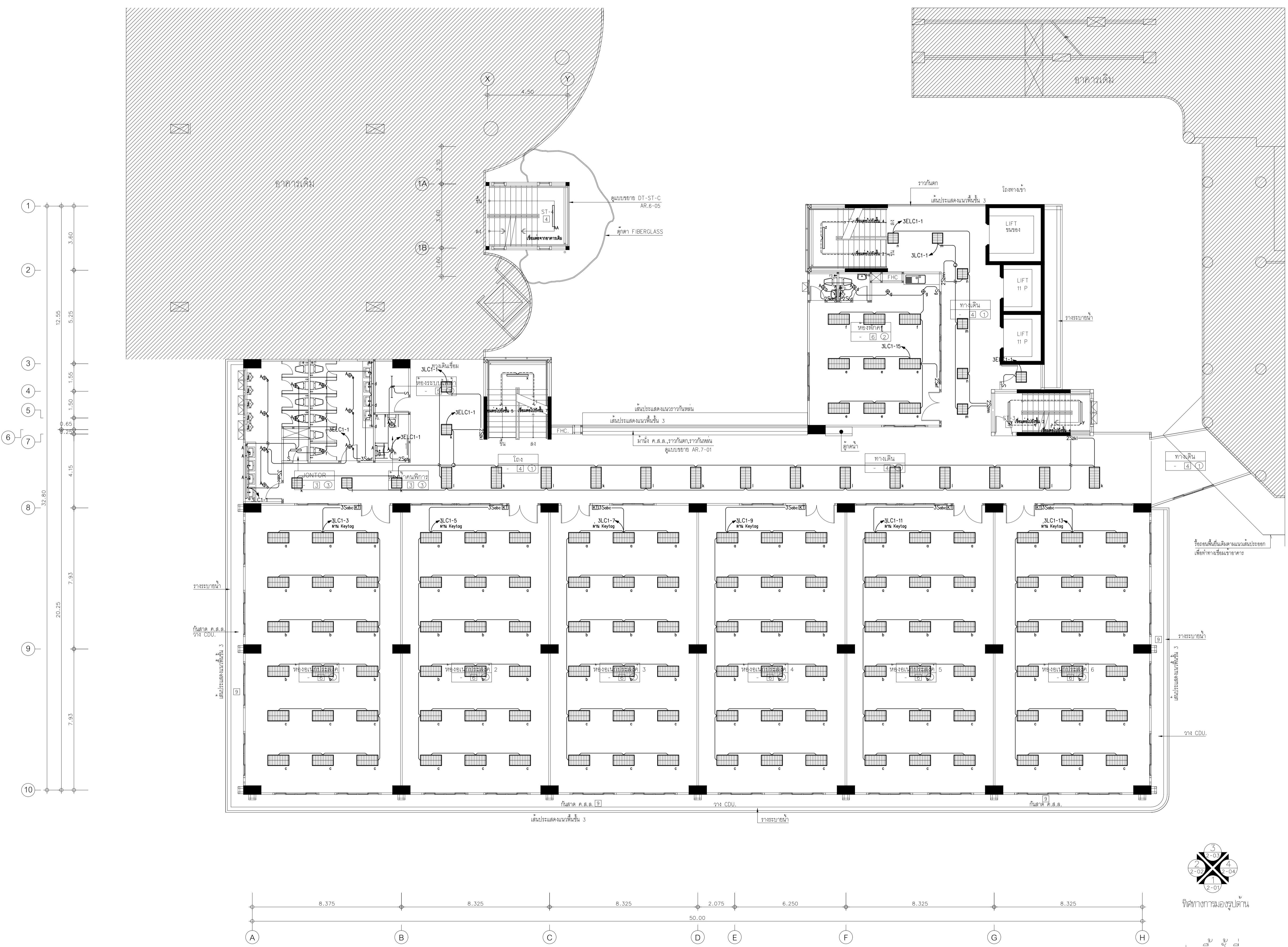
ผังระบบแสงสว่าง ชั้นที่ 3 มาตรฐาน 11100
