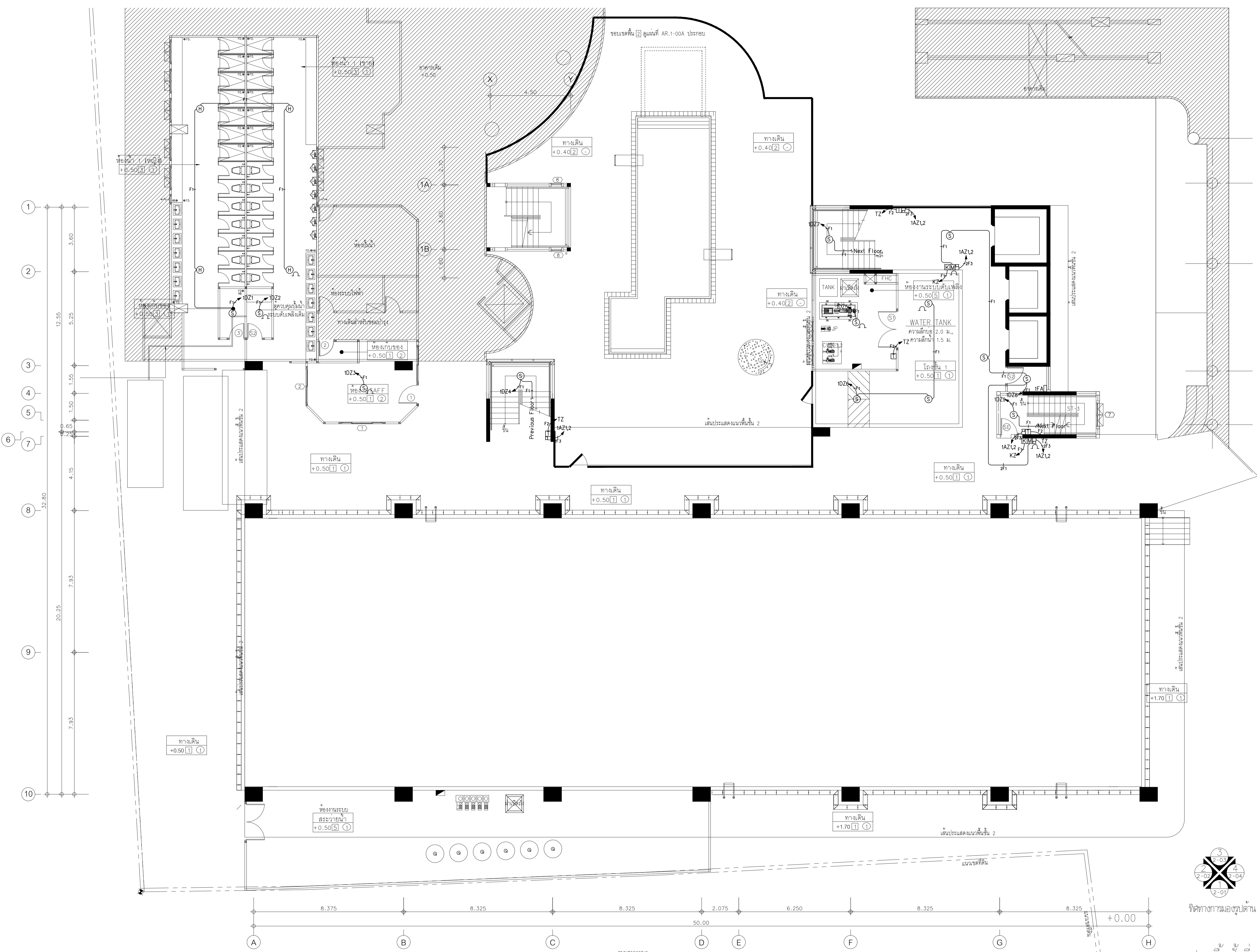
ผังระบบแรงเหวี่ยงใหม่ ชั้น 1 มาตราส่วน 1:100
