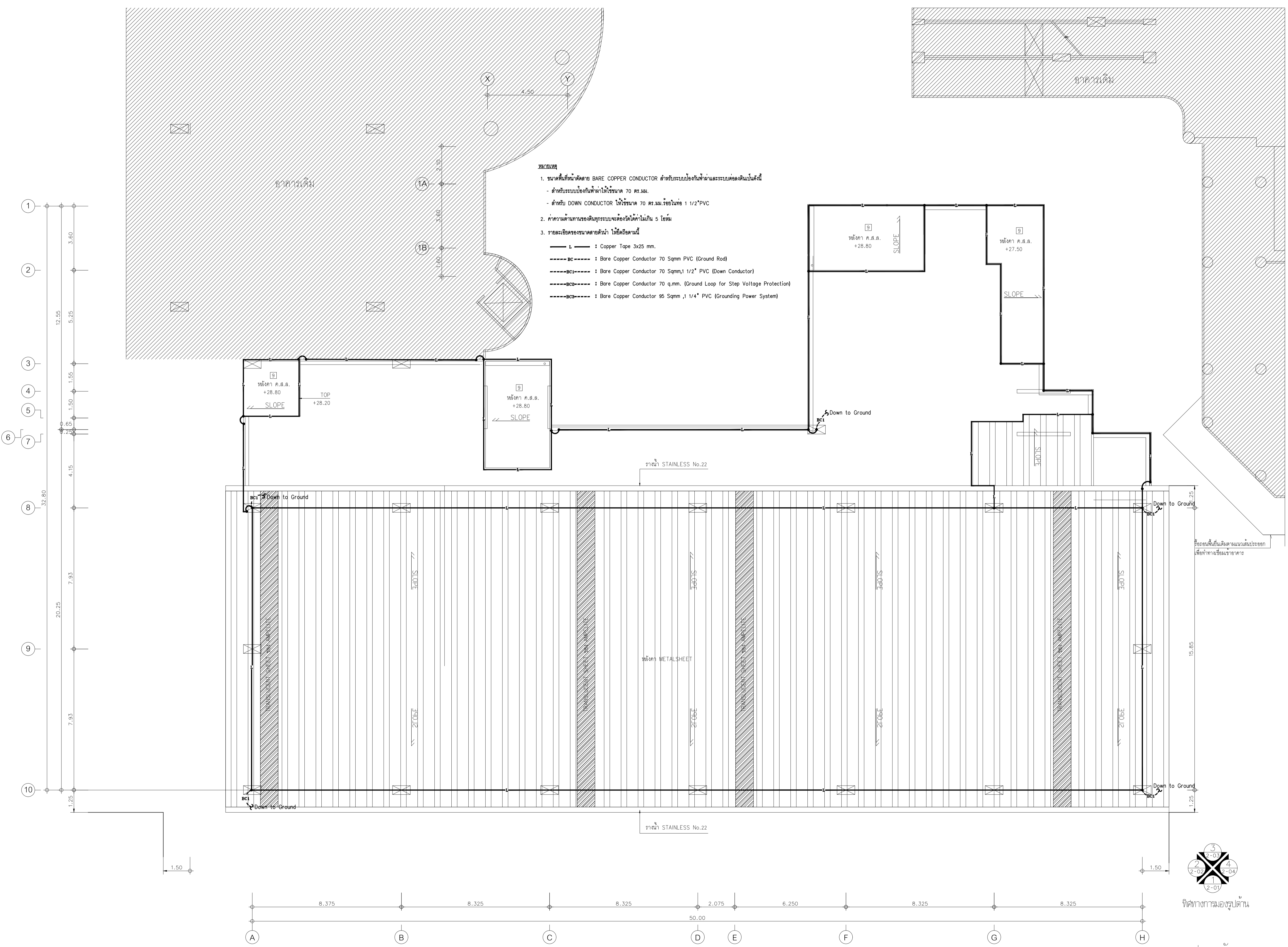
ผังระบบป้องกันฟ้าผ่า ชั้นดาดฟ้า มาตรฐาน 1:100
