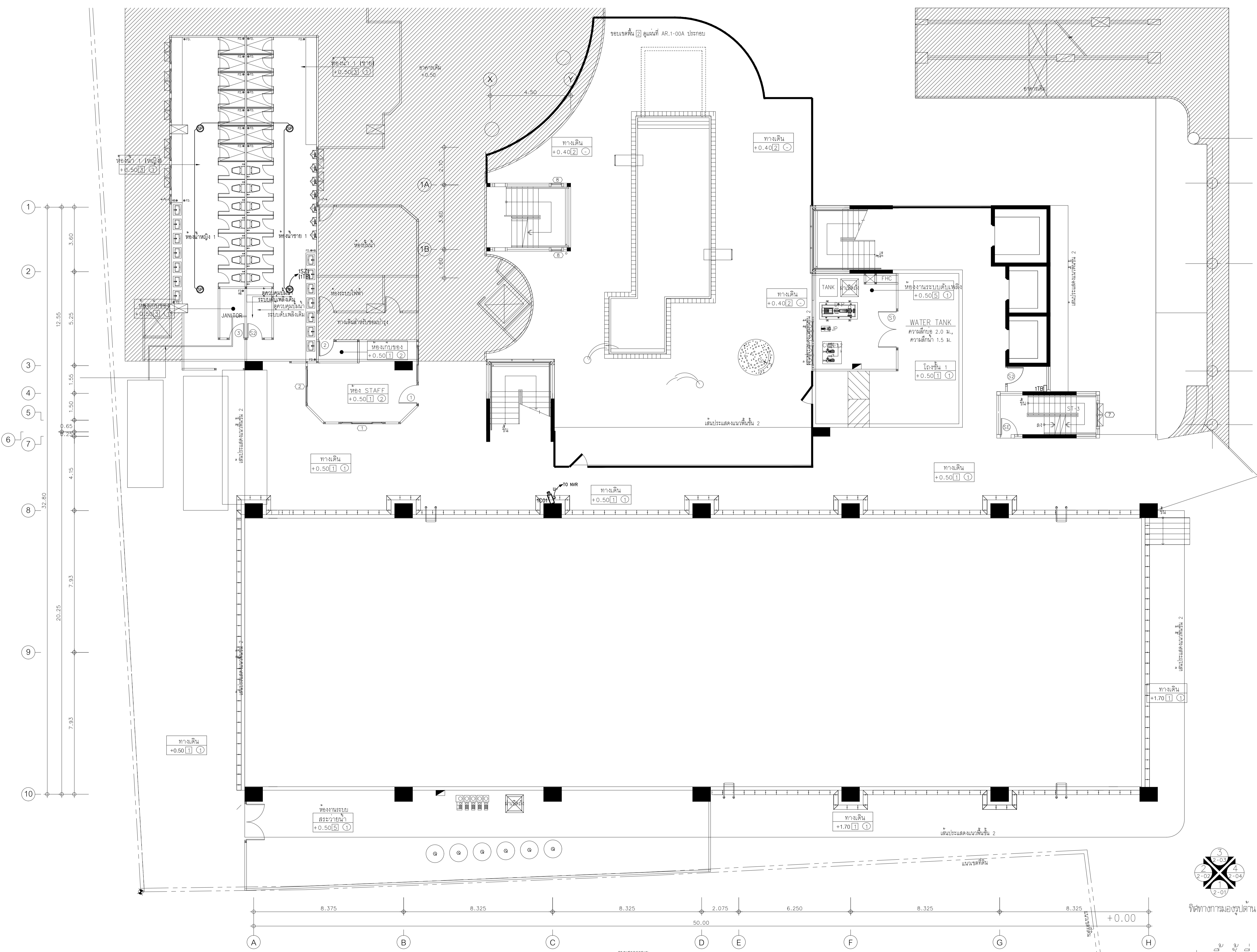
ผังระบบเสียงและระบบรักษาความปลอดภัย ชั้น 1 มาตราส่วน 1:100
