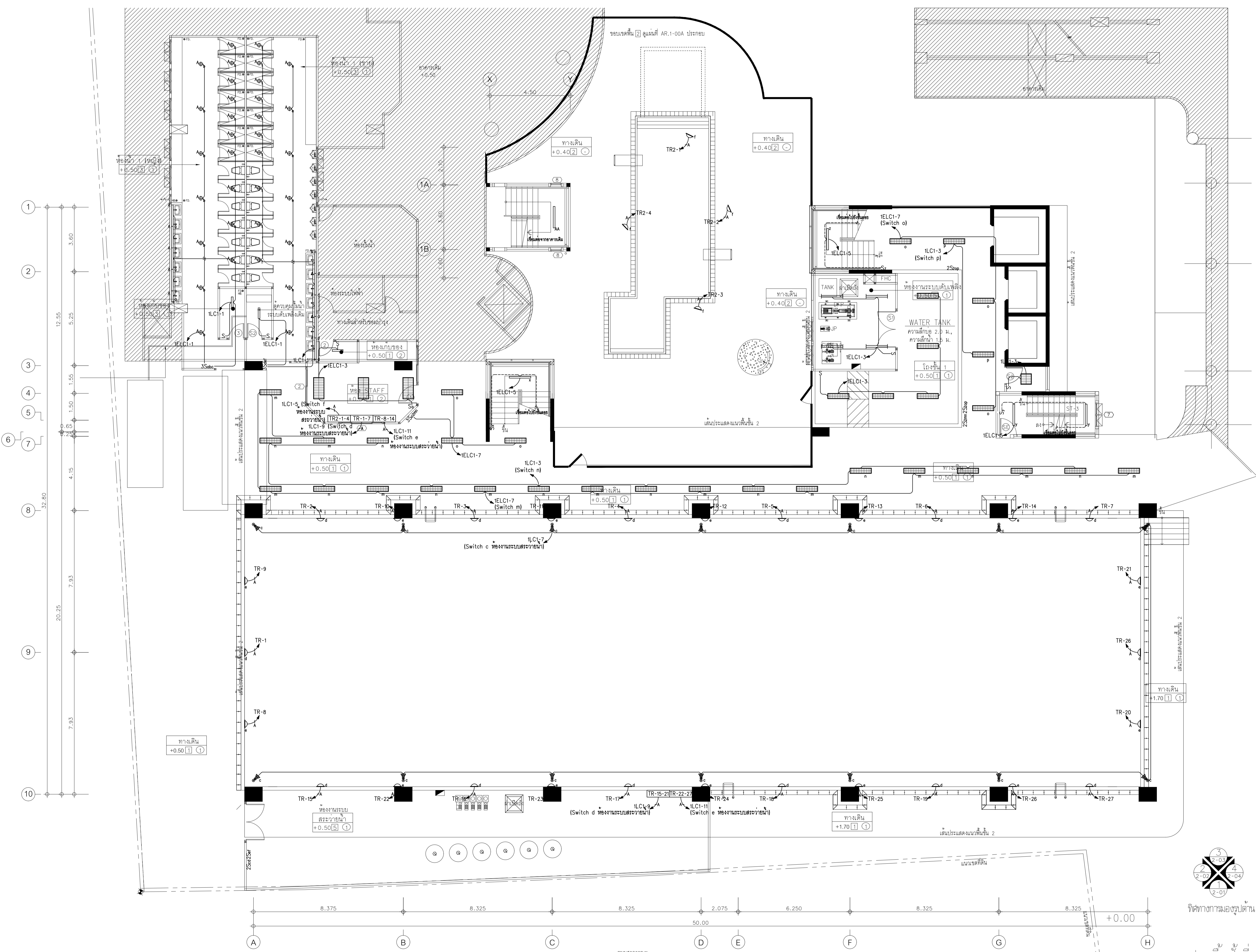
แผนอาคารรวมใจ ผังระบบแสงสว่าง ชั้นที่ 1 มาตรฐาน 1:100
