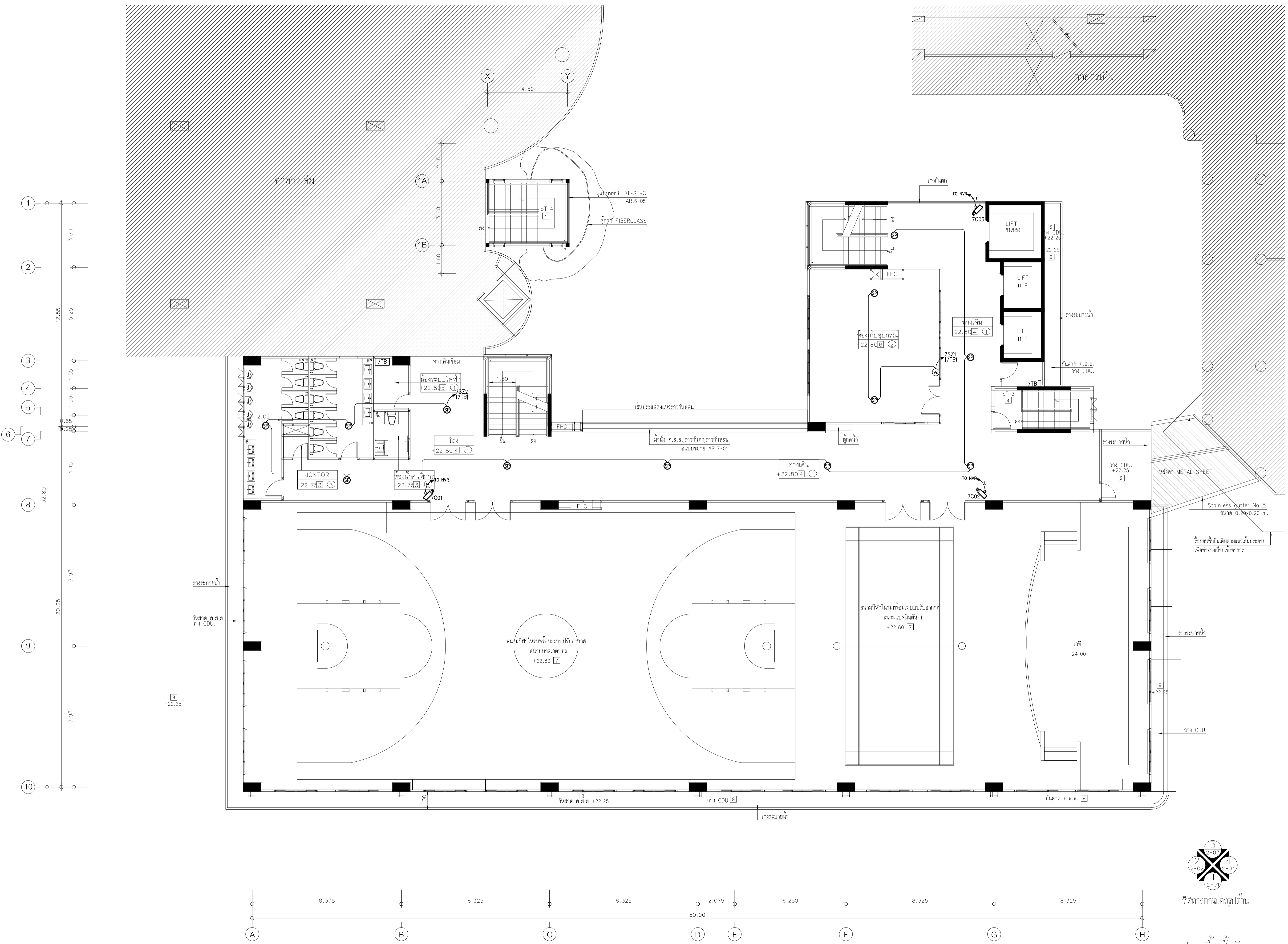
ผังระบบเสียงและระบบรักษาความปลอดภัย ชั้น 7 มาตราส่วน 1:100
