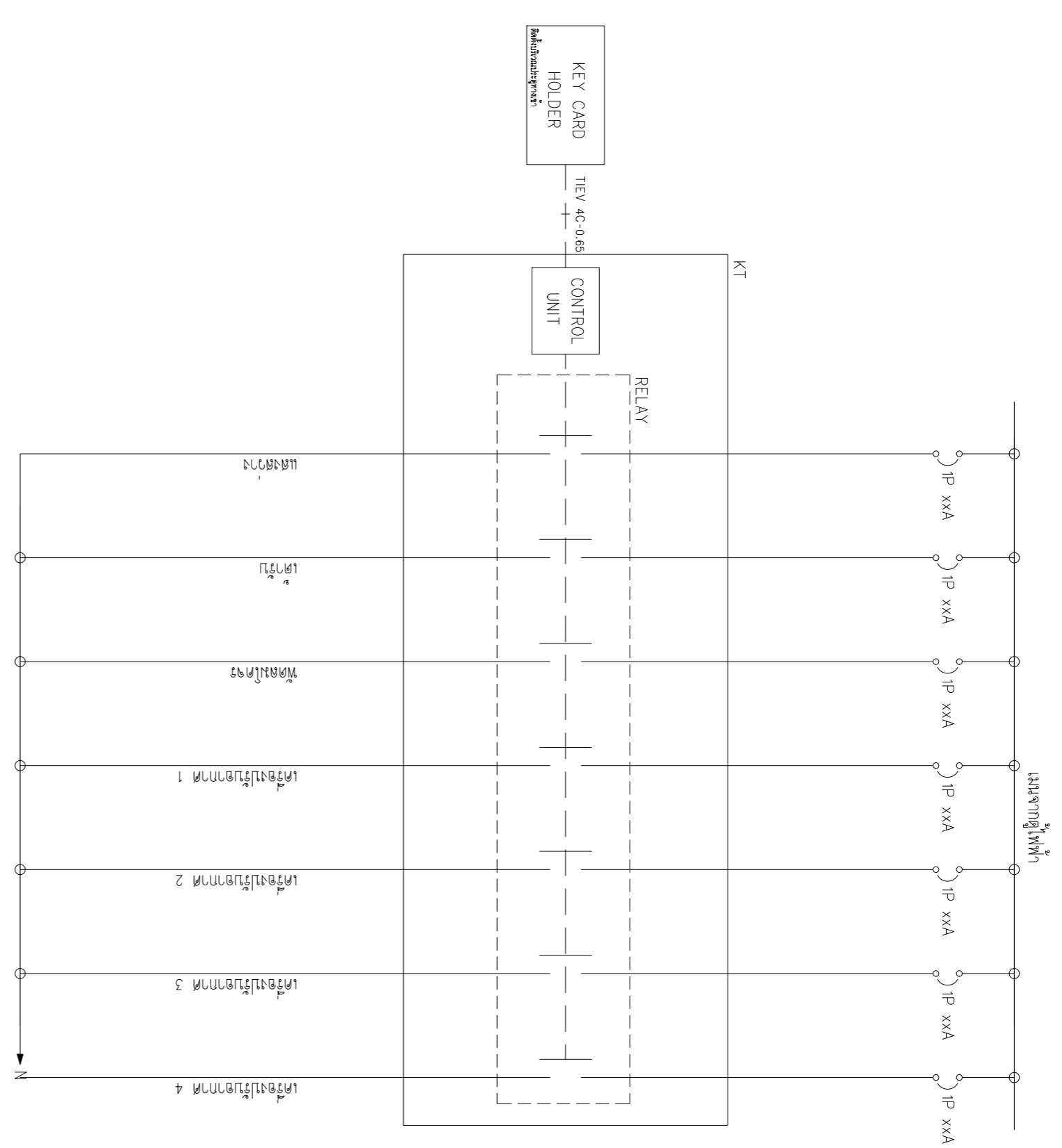
รายละเอียด KEYTAG (KT) : สำหรับห้องเครื่องปรับอากาศ 4 เครื่อง
