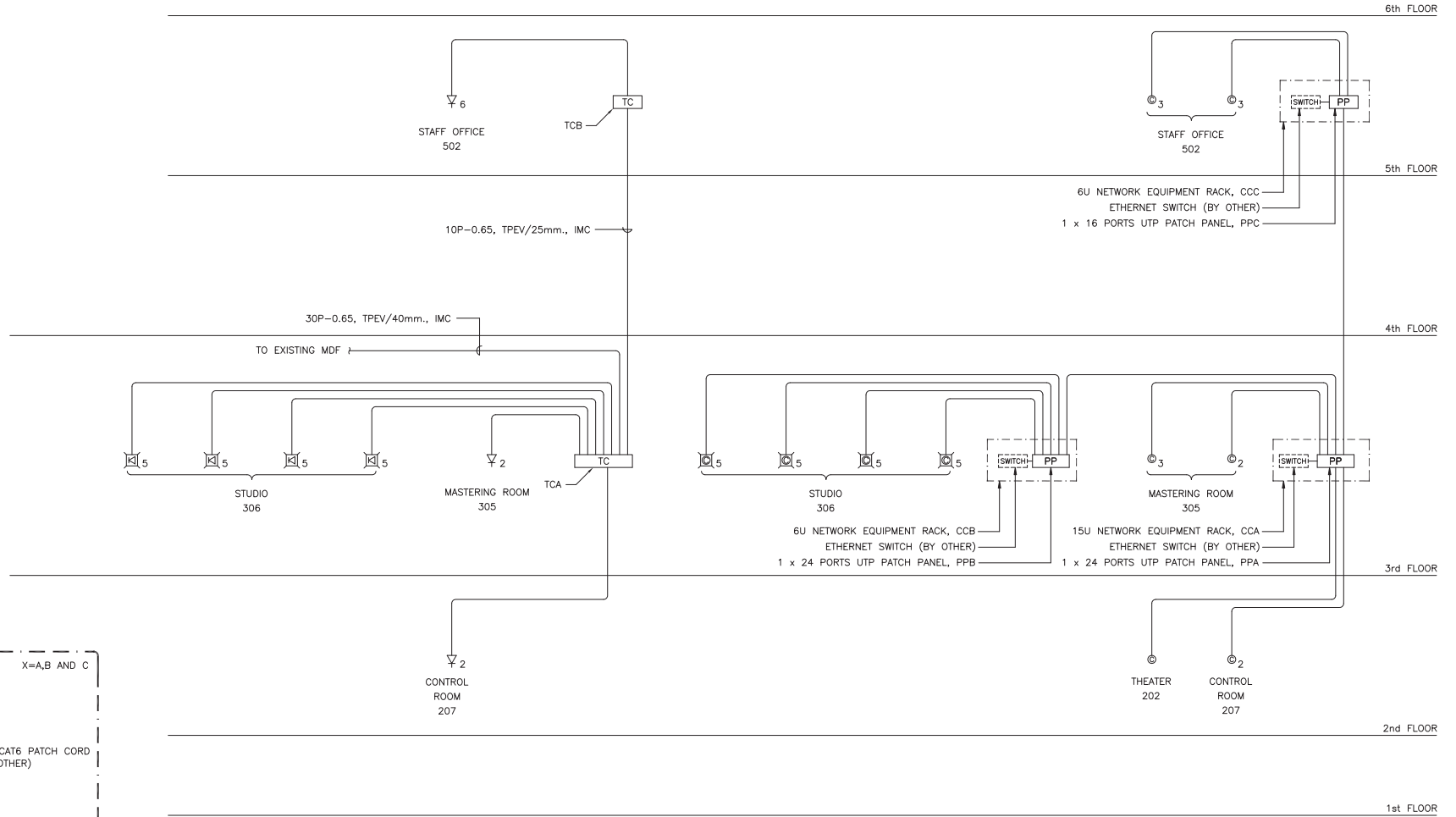
RISER DIAGRAM ระบบโทรศัพท์
