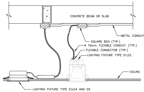
รายละเอียดการติดตั้ง 4 การติดตั้งโคมไฟ DOWNLIGHT ชนิดฝังฝ้าเพดาน NOT TO SCALE
