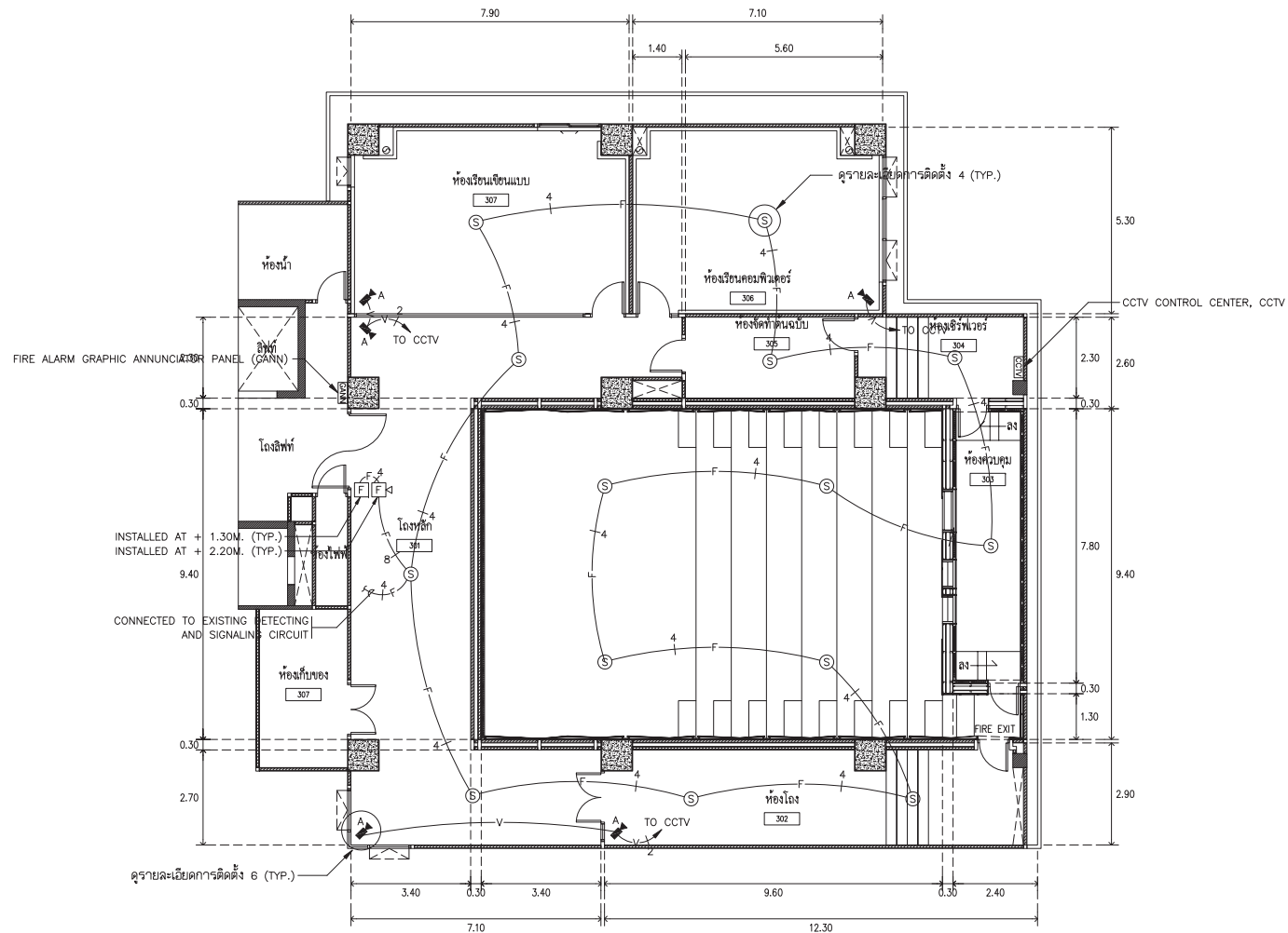
ผังระบบสัญญาณแจ้งเพลิงไหม้ และระบบโทรทัศน์วงจรปิด ชั้นที่ 3 SCALE 1 : 100
