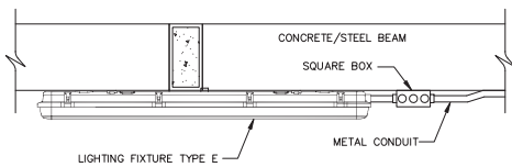
รายละเอียดการติดตั้ง 7 การติดตั้งโคมไฟกั้นน้ำชนิดติดตั้งที่ผนัง NOT TO SCALE
