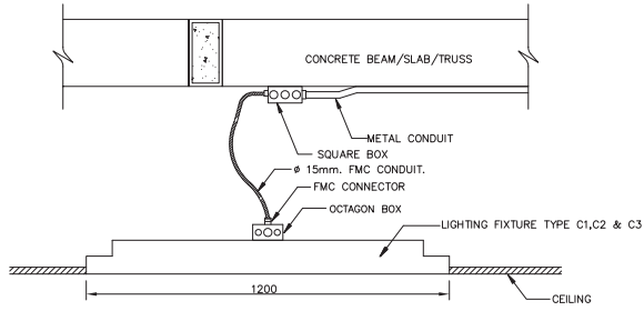
รายละเอียดการติดตั้ง 1 การติดตั้งโคมไฟแสงสว่างชนิดฝังฝ้าเพดาน NOT TO SCALE
