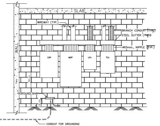
รายละเอียดการติดตั้ง 9 ELECTRICAL AND COMMUNICATION DISTRIBUTION PANEL INSTALLATION DETAIL NOT TO SCALE
