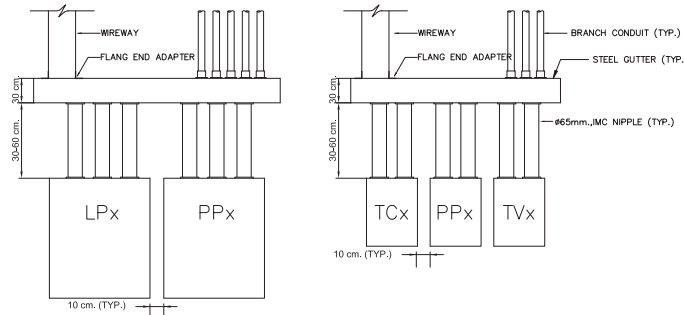
รายละเอียดการติดตั้ง 8 TYPICAL ARRANGEMENT INSTALLATION OF ELECTRICAL PANELBOARD AND COMMUNICATION PANEL NOT TO SCALE
