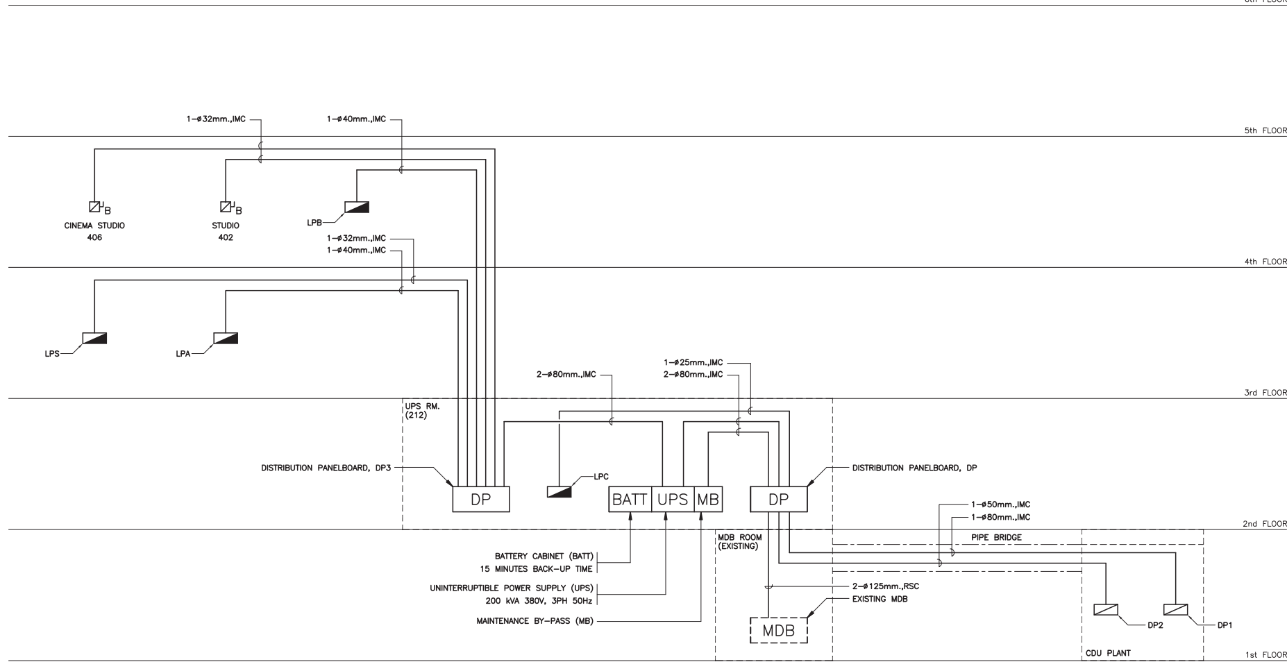
RISER DIAGRAM ระบบไฟฟ้ากำลัง
