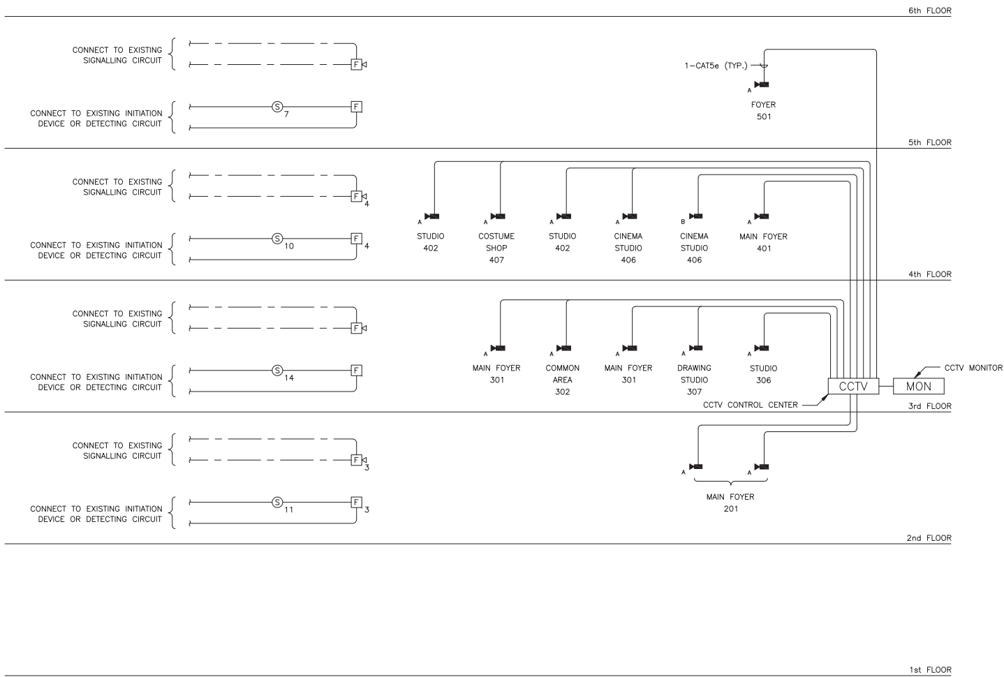
RISER DIAGRAM ระบบสัญญาณแจ้งเพลิงไหม้
