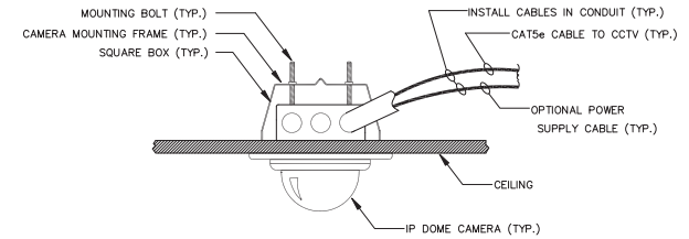
รายละเอียดการติดตั้ง 3 การติดตั้ง INDOOR IP DOME CAMERA แบบฝังฝ้าเพดาน NOT TO SCALE
