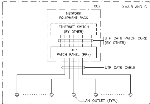
RISER DIAGRAM ระบบสายสัญญาณเครือข่ายคอมพิวเตอร์
