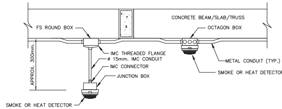
รายละเอียดการติดตั้ง 2 การติดตั้ง FIRE ALARM DETECTOR แบบติดตั้งใต้ฝ้าเพดาน NOT TO SCALE
