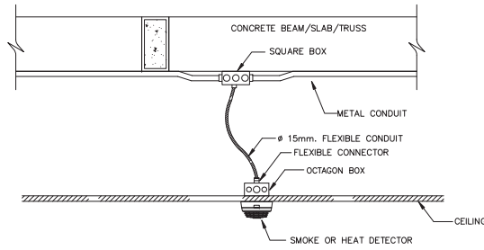
รายละเอียดการติดตั้ง 2 การติดตั้ง FIRE ALARM DETECTOR แบบติดตั้งใต้ฝ้าเพดาน NOT TO SCALE
