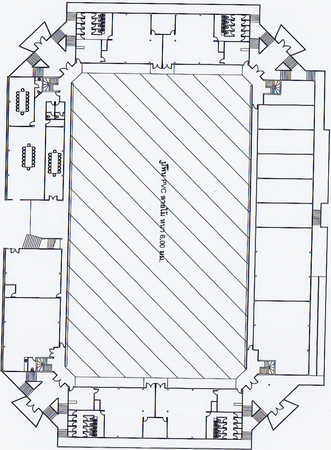
แปลนอาคารกีฬา (ชั้นแข่งขัน) ม. ศรีนครินทรวิโรฒ องครักษ์ SCALE 1 : 350
